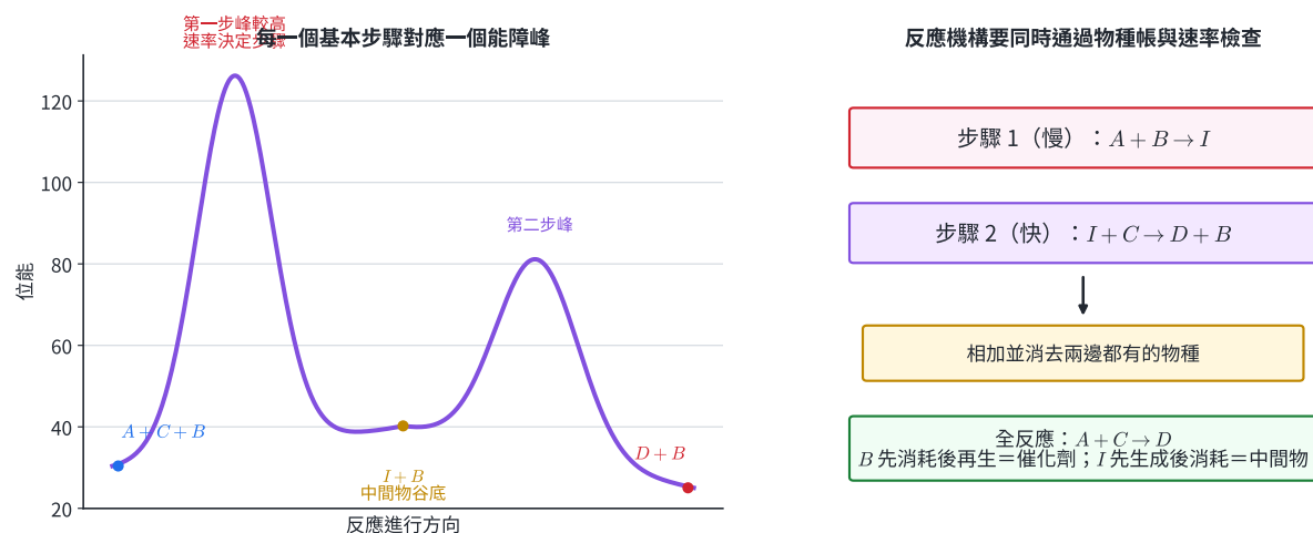
圖 8 | 兩個基本步驟對應兩個能障峰； B 在第一步消耗、第二步再生， I 在第一步生成、第二步消耗。
