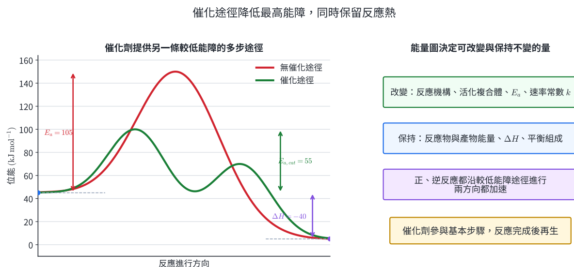
圖 10 | 催化與無催化途徑共用同一對反應物、產物能階；催化途徑的最高能障較低， \Delta H = -40 \text{ kJ mol}^{-1} 保持不變。
