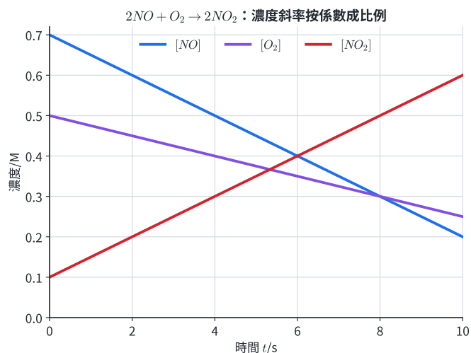
圖 2 | 在 2NO + O_2 \rightarrow 2NO_2 中，NO 與 NO 2 的濃度斜率大小是 O 2 的兩倍；以係數歸一後皆得到同一個 r 。
