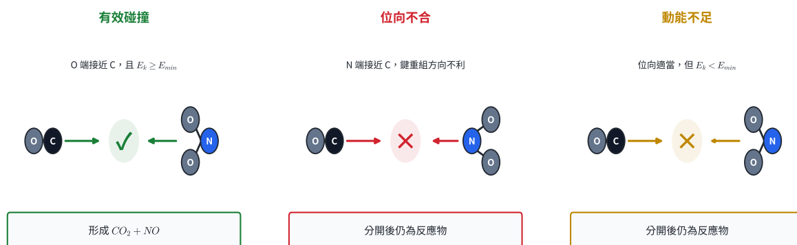
圖 5 | 對 \text{CO} + \text{NO}_2 \rightarrow \text{CO}_2 + \text{NO} 而言，CO 的 C 端接近 \text{NO}_2 的 O 端，並有足夠碰撞動能時，才能完成 O 原子轉移。
