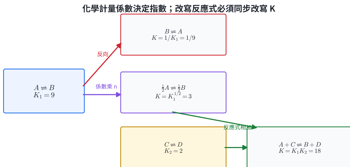
圖 2 | 由同一個 K=9 的反應出發，追蹤反向、係數乘二分之一與反應式相加。
