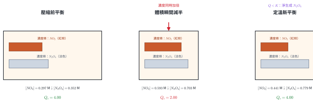
圖 8 | NO_2/N_2O_4 平衡的體積減半計算：濃度先加倍， Q 由 4.00 降至 2.00，再由 -2y 、 +y 建立新平衡。
