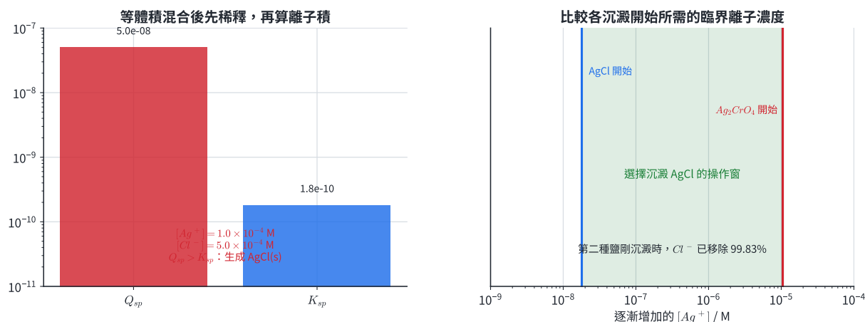
圖 14 | 左圖比較混合後 Q_{sp} 與 K_{sp} ；右圖以 \text{Ag}^+ 臨界濃度畫出 AgCl 與 \text{Ag}_2\text{CrO}_4 的選擇沉澱窗。
