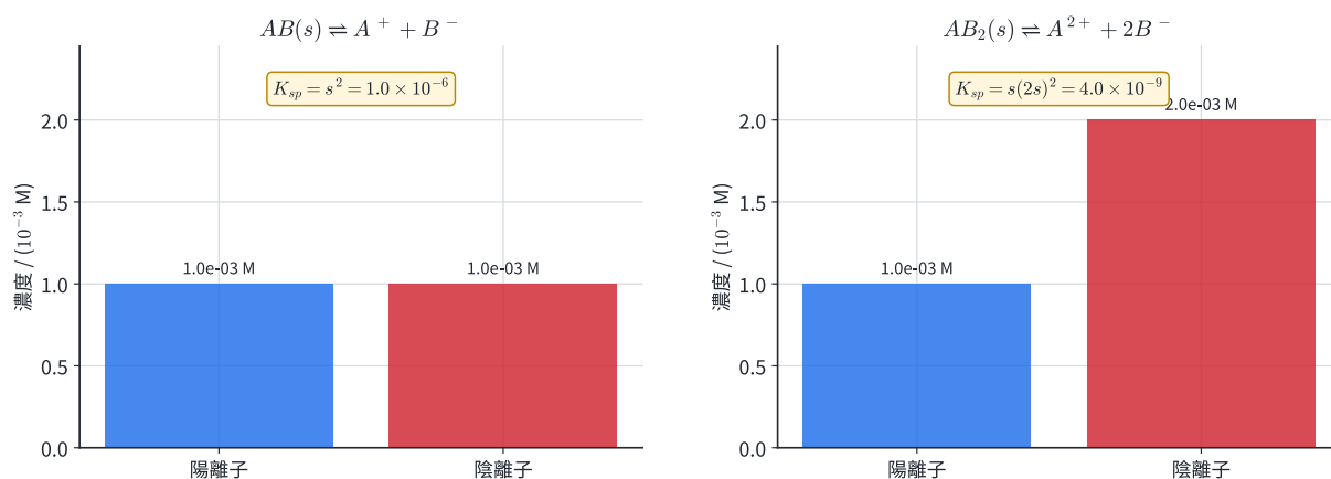
圖 12 | AB 與 AB 2 都取 s=10^{-3} M ；陰離子濃度與 K_{sp} 的次方因化學計量不同。
