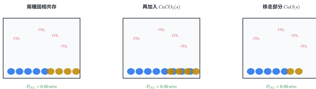
圖 5 | 只要 \text{CaCO}_3 、 \text{CaO} 兩固相仍共存，改變固體量不改變平衡 \text{CO}_2 分壓；相完全消失後，原平衡的適用條件改變。
