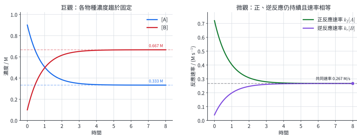
圖 1 | 左圖追蹤 A、B 濃度，右圖追蹤正、逆速率；平衡判準是速率相等，而各物種濃度各自停在固定值。
