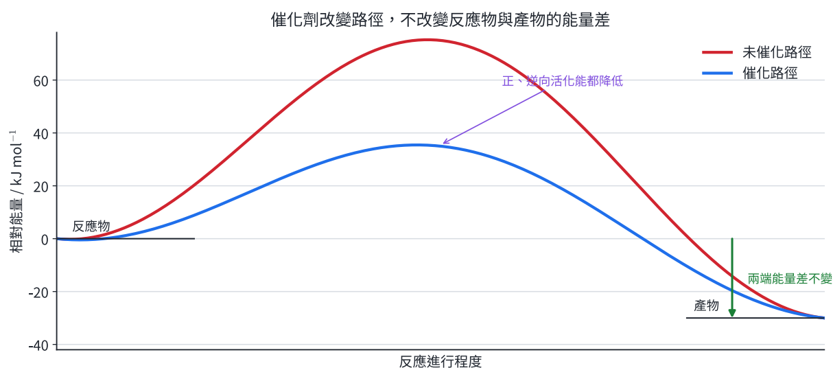
圖 10 | 催化與未催化路徑的兩端能量相同，催化路徑峰值較低；因此 K 與平衡位置相同。
