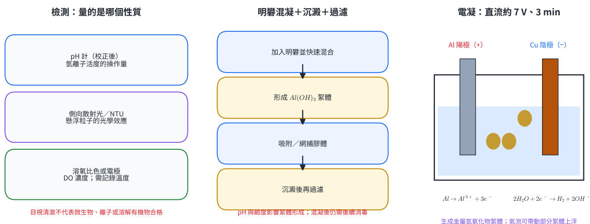
圖 8 | 三欄依序建立檢測量、明礬混凝流程與直流電凝的電極反應。
