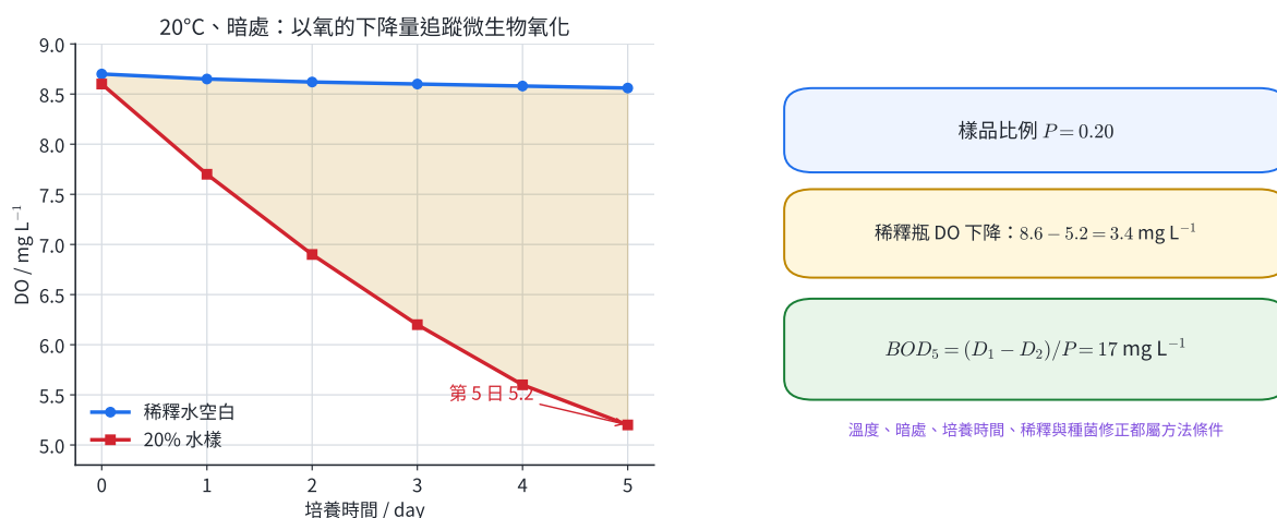
圖 5 | 左圖以暗處五日 DO 下降建立 BOD 證據；右圖顯示稀釋比例如何進入換算。
