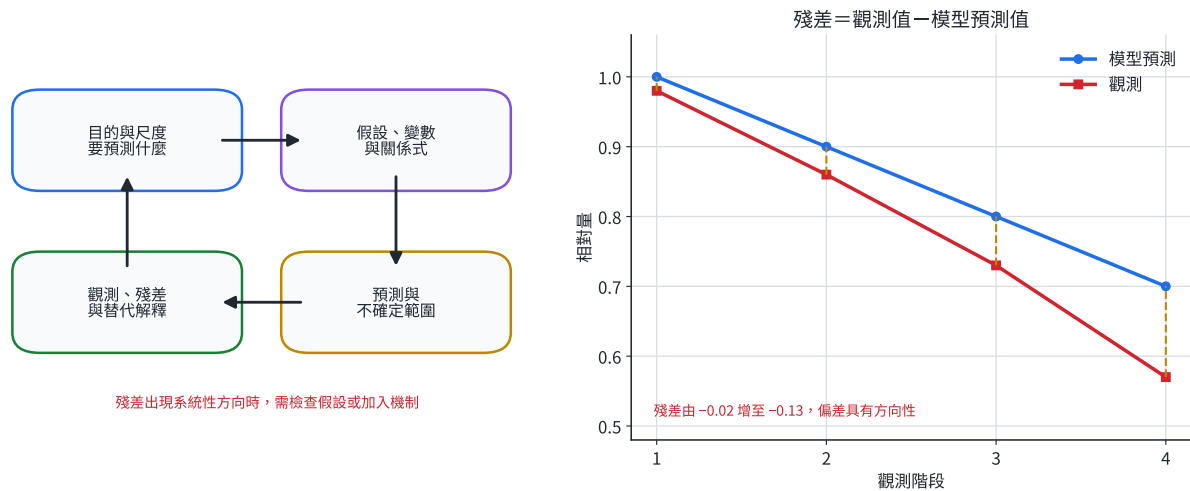
圖 2 | 左圖依序連結目的、假設、預測與觀測；右圖用逐步增大的殘差指出模型需要修正。
