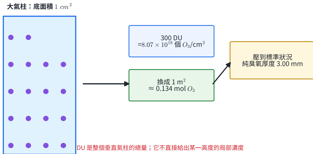
圖 4 | 把 300 DU 依序換成每平方公分分子數、每平方公尺莫耳數與標準狀況厚度。
