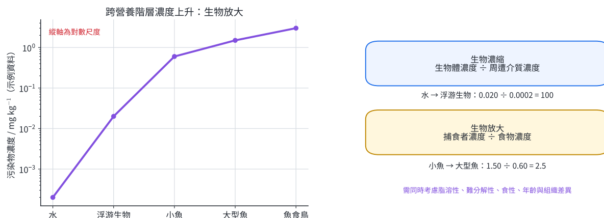
圖 7 | 左圖以對數尺度呈現跨五個介質／營養階層的濃度；右圖分別計算濃縮與放大倍數。
