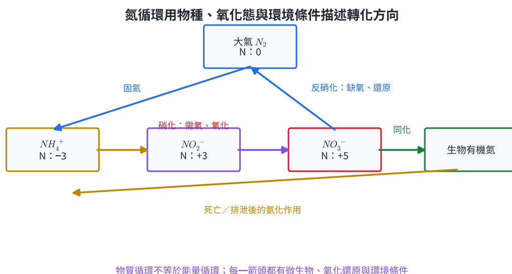
圖 11 | 每個氮庫標出化學物種與 N 氧化數；箭頭同時標出固氮、硝化、同化、氨化與反硝化。
