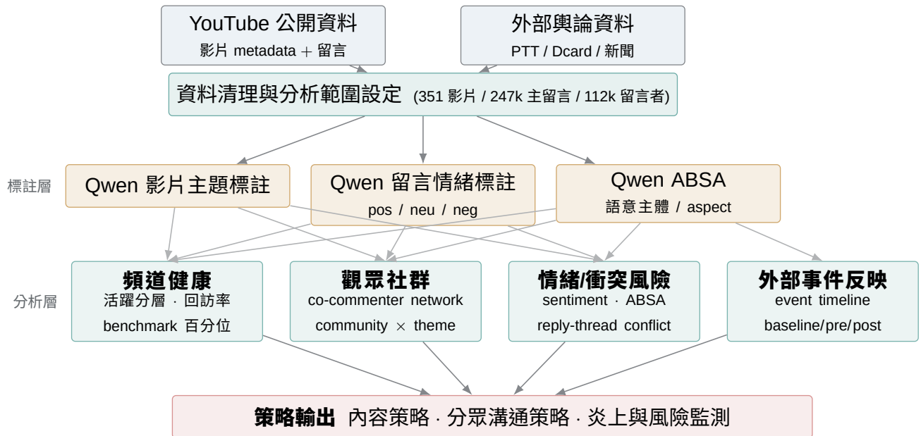
Figure 1: 研究分析架構與資料流。資料層整合 YouTube 公開留言與外部輿論資料，經清理後由 Qwen 進行影片主題、留言情緒與 ABSA 語意主體標註；分析層包含頻道健康、觀眾社群、情緒／衝突風險與外部事件反映四個模組，最終轉化為內容、分眾溝通與風險監測策略。
