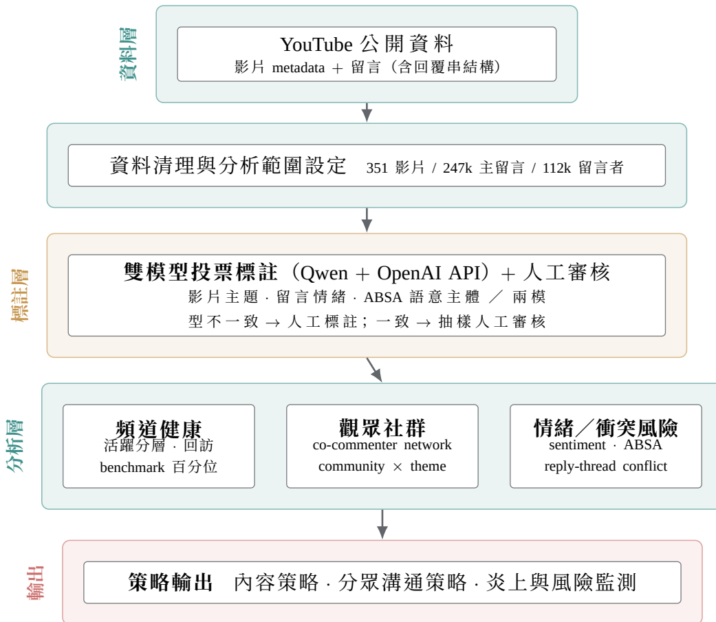
Figure 1: 研究分析架構與資料流（由上而下分為五層）。YouTube 公開留言經前處理後，由標註層以雙模型投票（Qwen 與 OpenAI API）加人工審核產生影片主題、留言情緒與 ABSA 語意主體標註；分析層包含頻道健康、觀眾社群與情緒／衝突風險三個模組，最終於輸出層轉化為內容、分眾溝通與風險監測策略。
