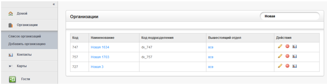
Рисунок 12 Результат поиска.
