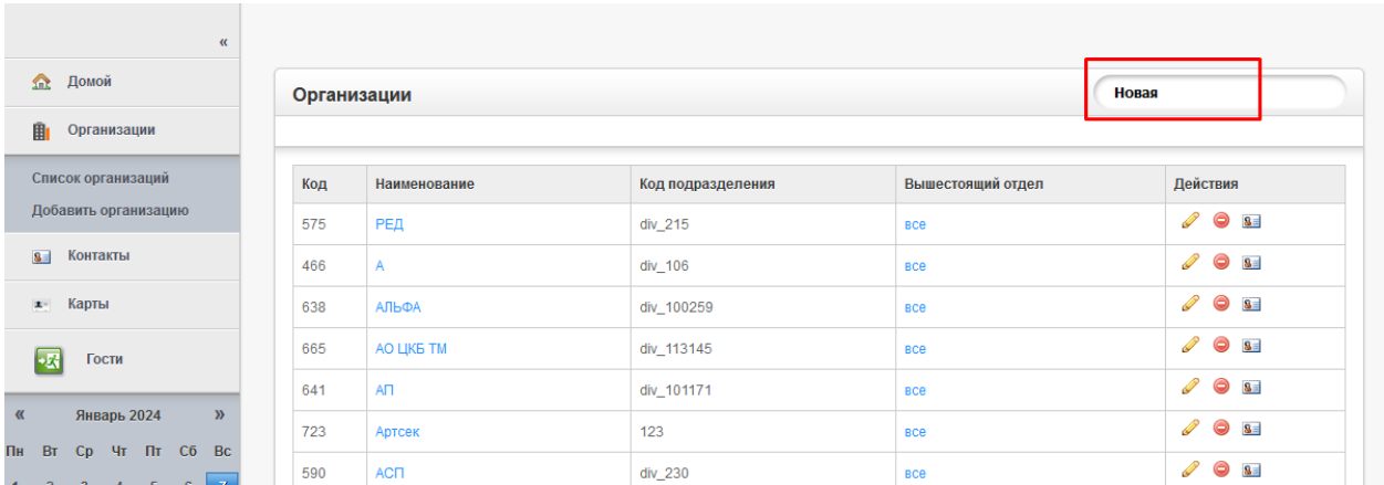
Рисунок 11 Поиск организации.
