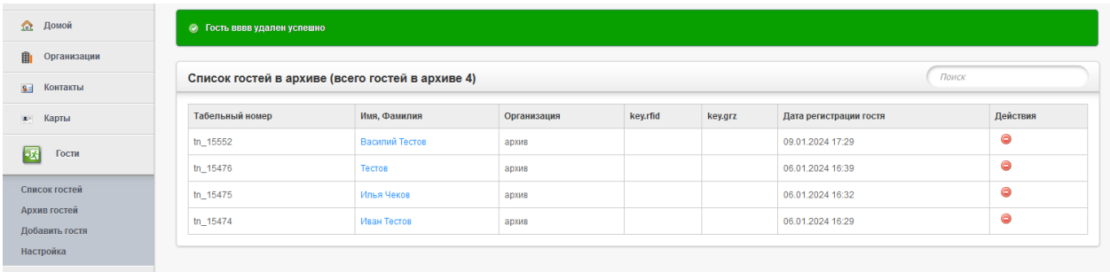
Рисунок 5 Архив гостей.
