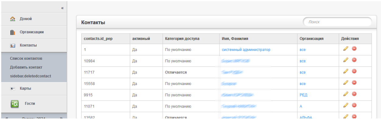
Рисунок 16 Список контактов
