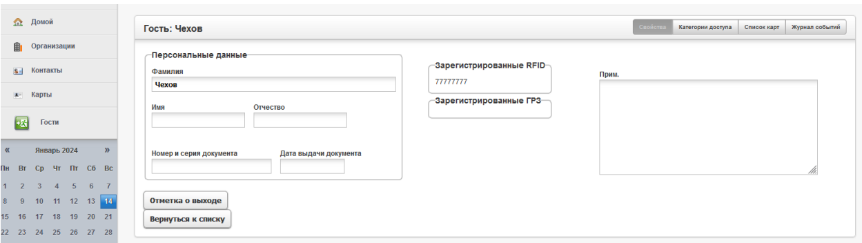
Рисунок 4 Свойства гостя.
