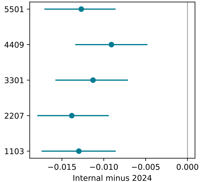
Macro-F1 gap
