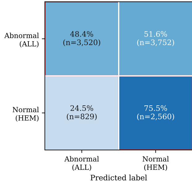
True label
