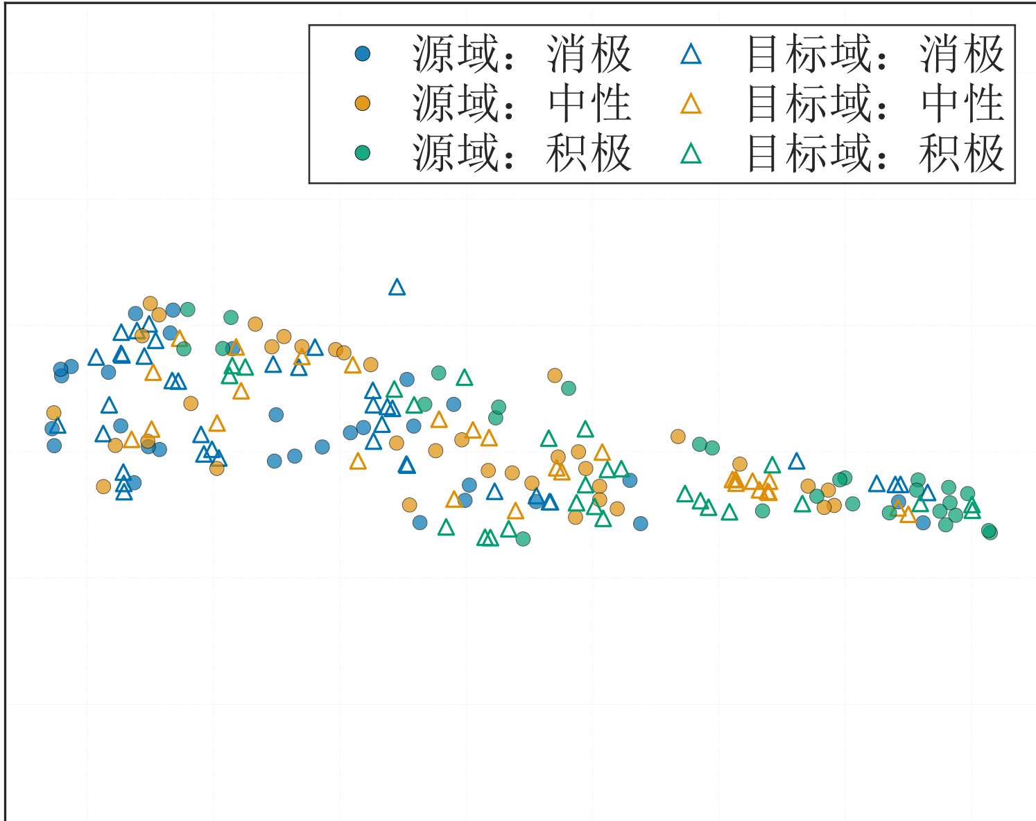
t-SNE 成分 1
