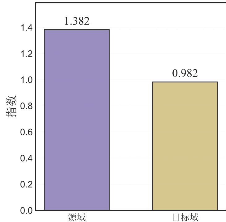
可分性指数
