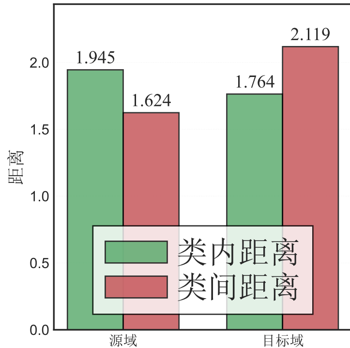
距离度量
