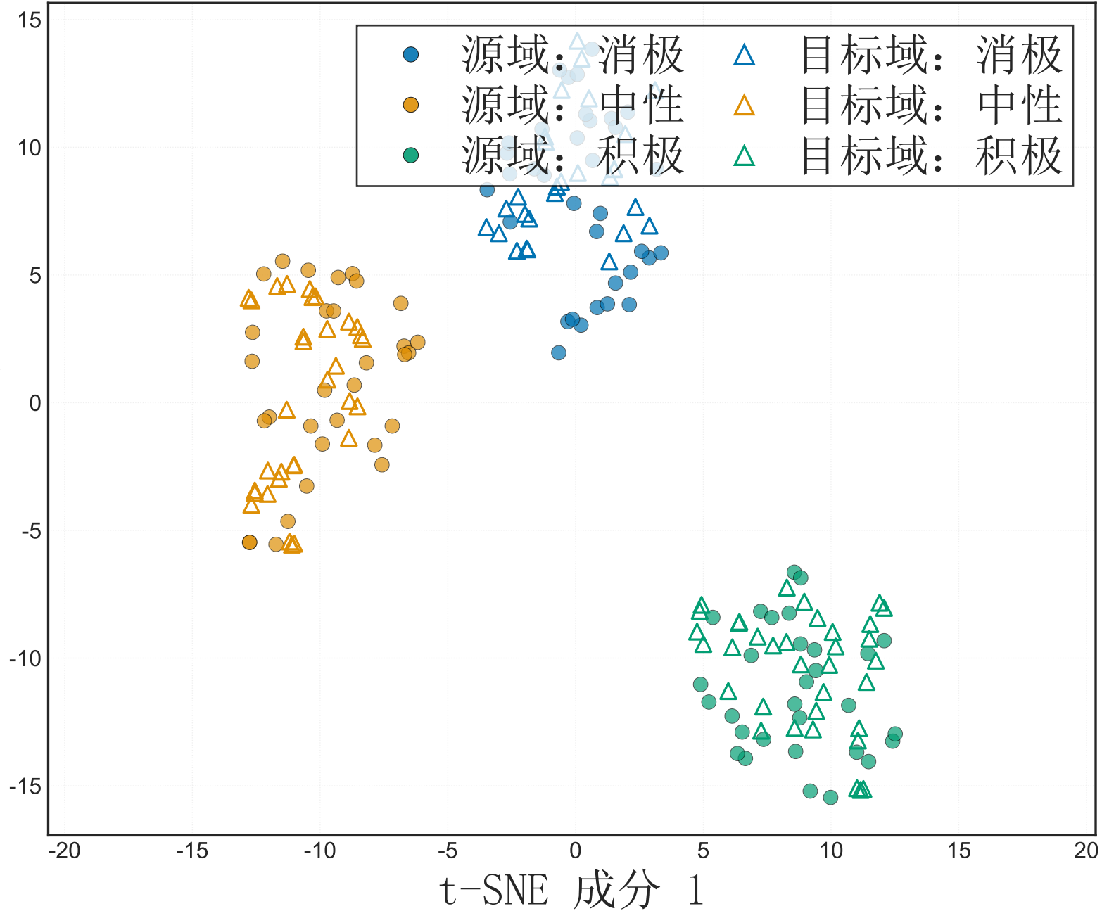
t-SNE 成分 2
