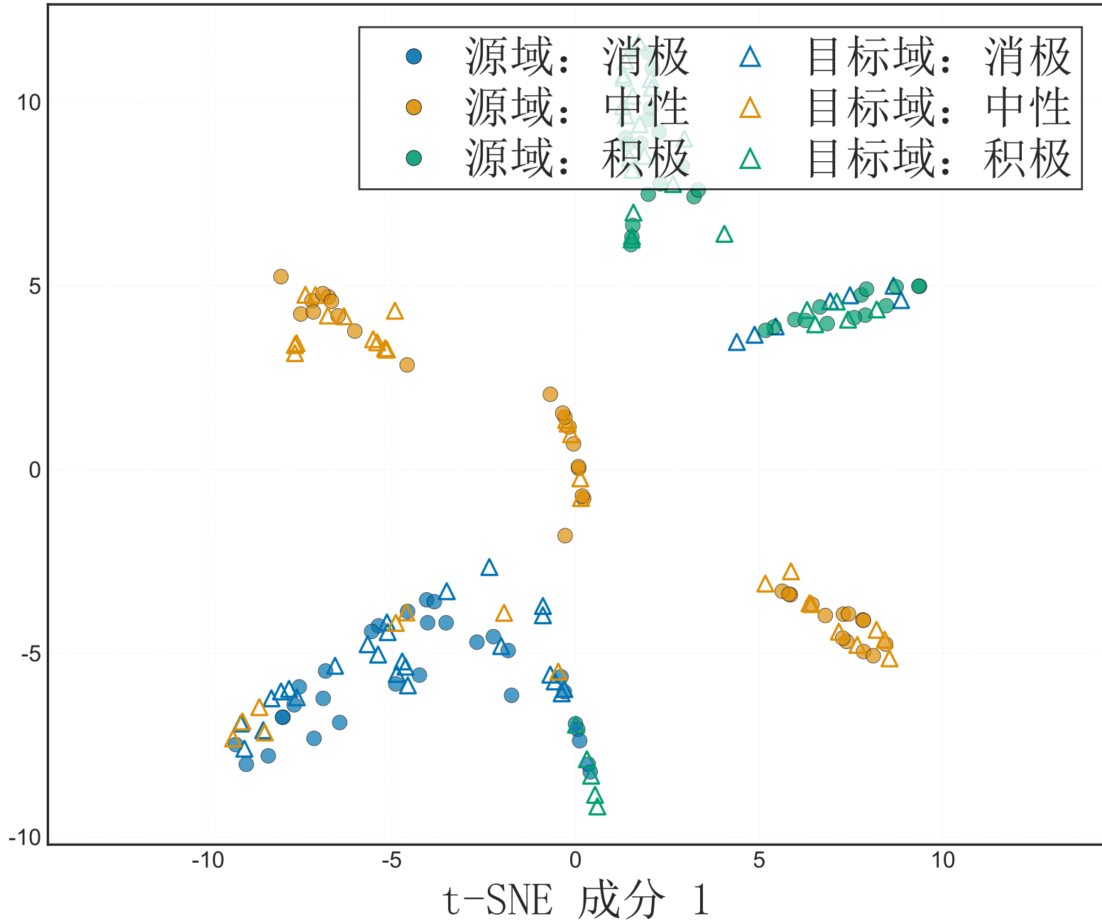
t-SNE 成分 2
