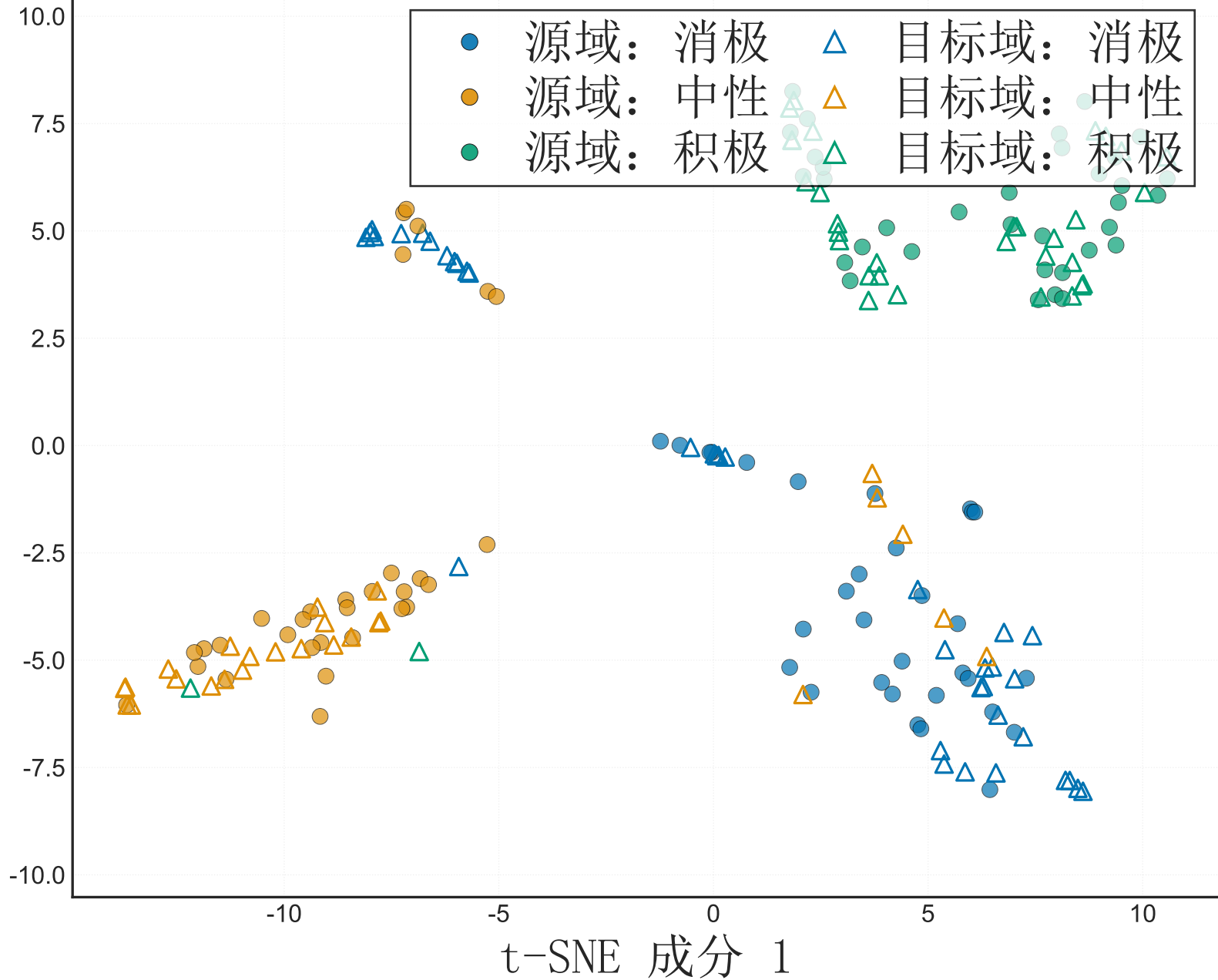
t-SNE 成分 2
