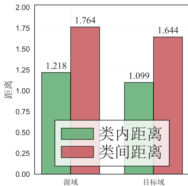
距离度量
