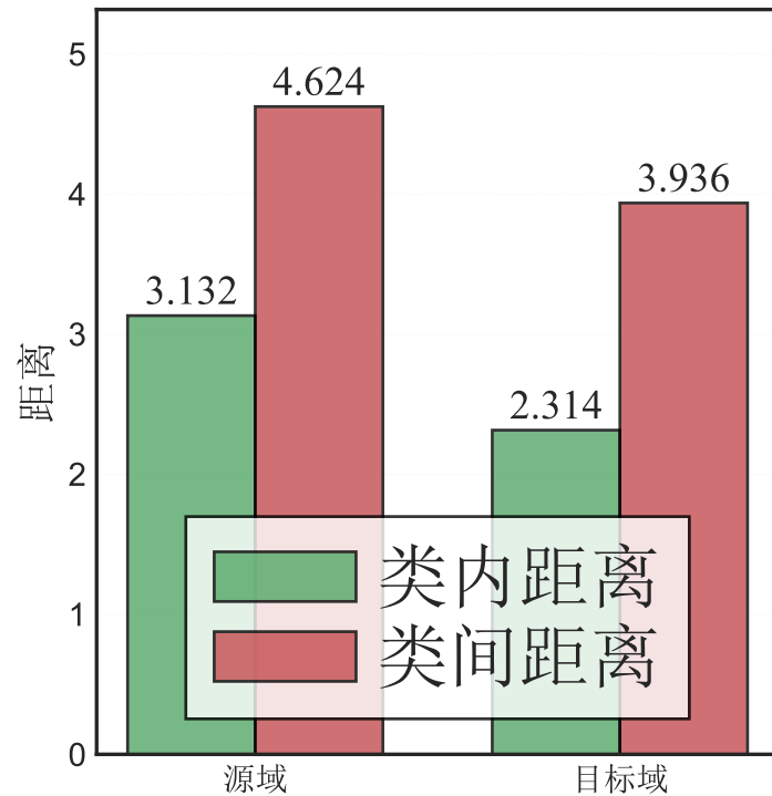
距离度量
