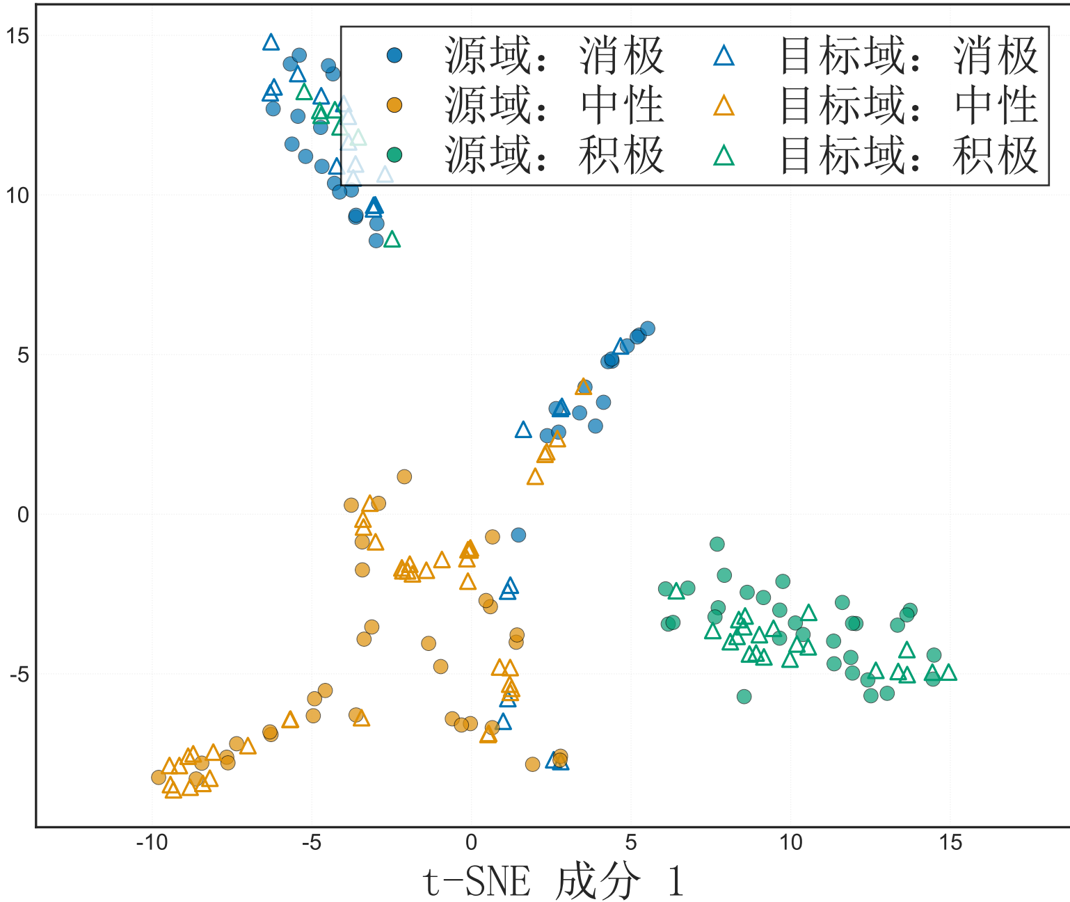
t-SNE 成分 2
