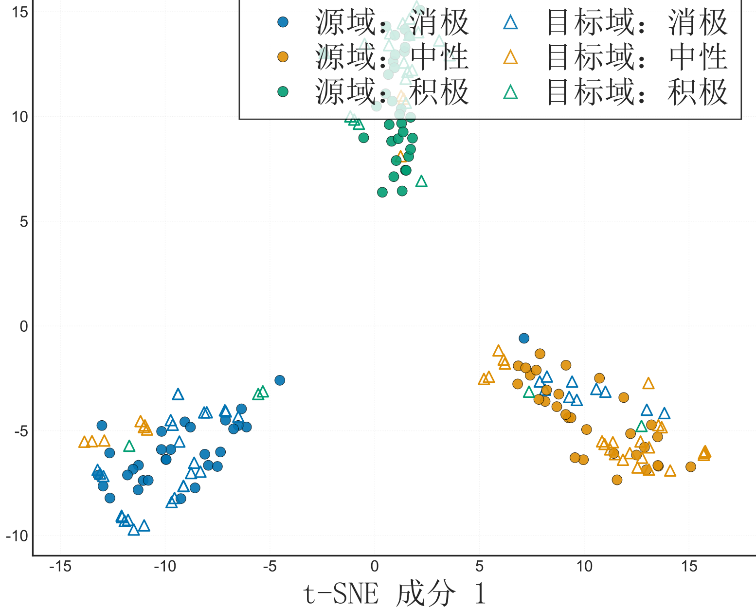
t-SNE 成分 2
