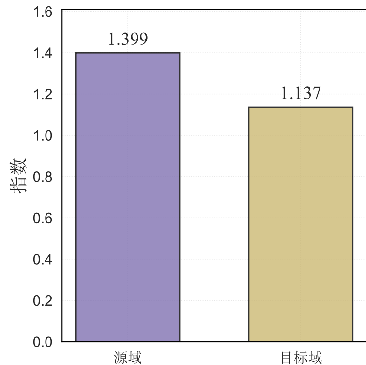
可分性指数
