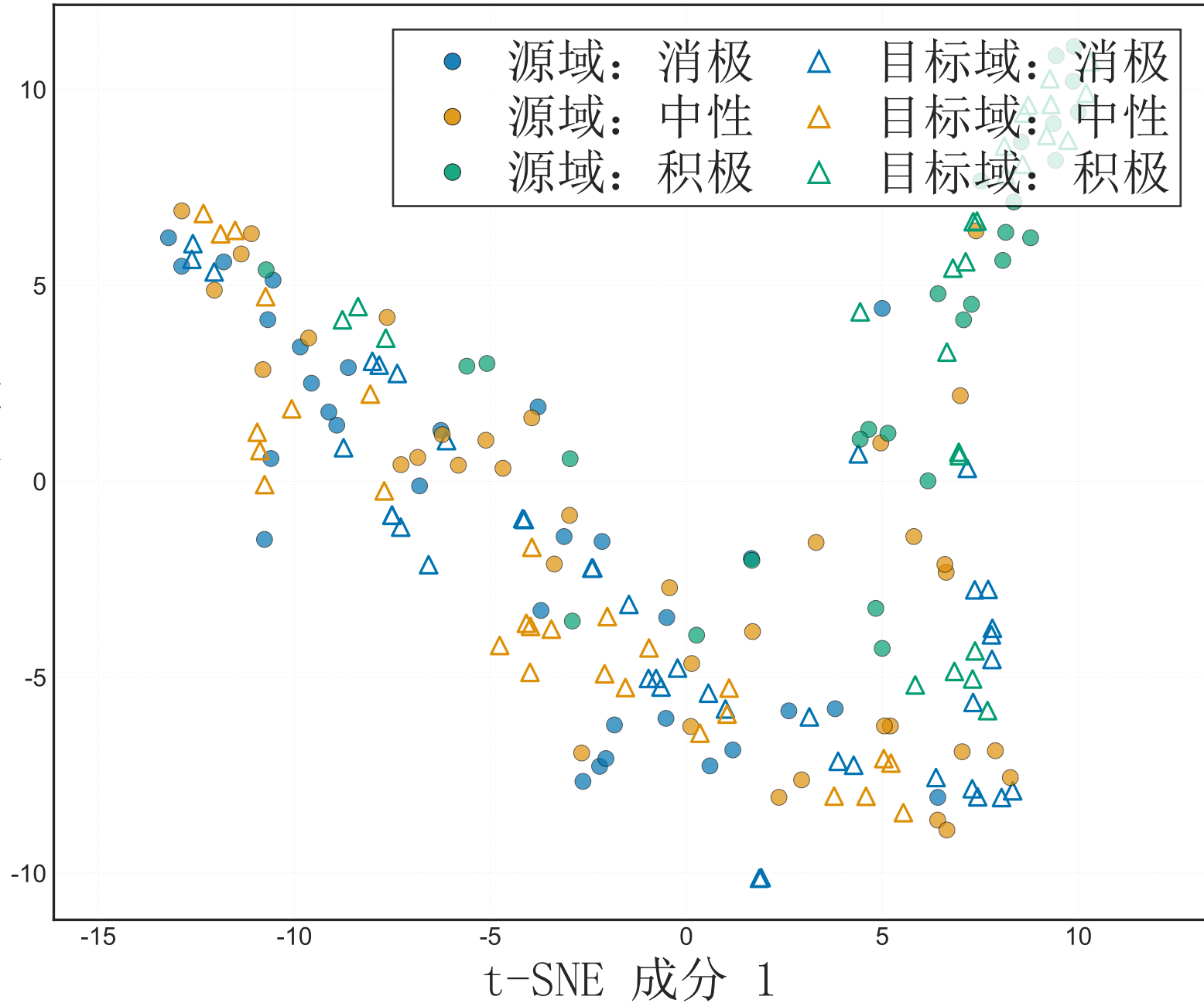
t-SNE 成分 2
