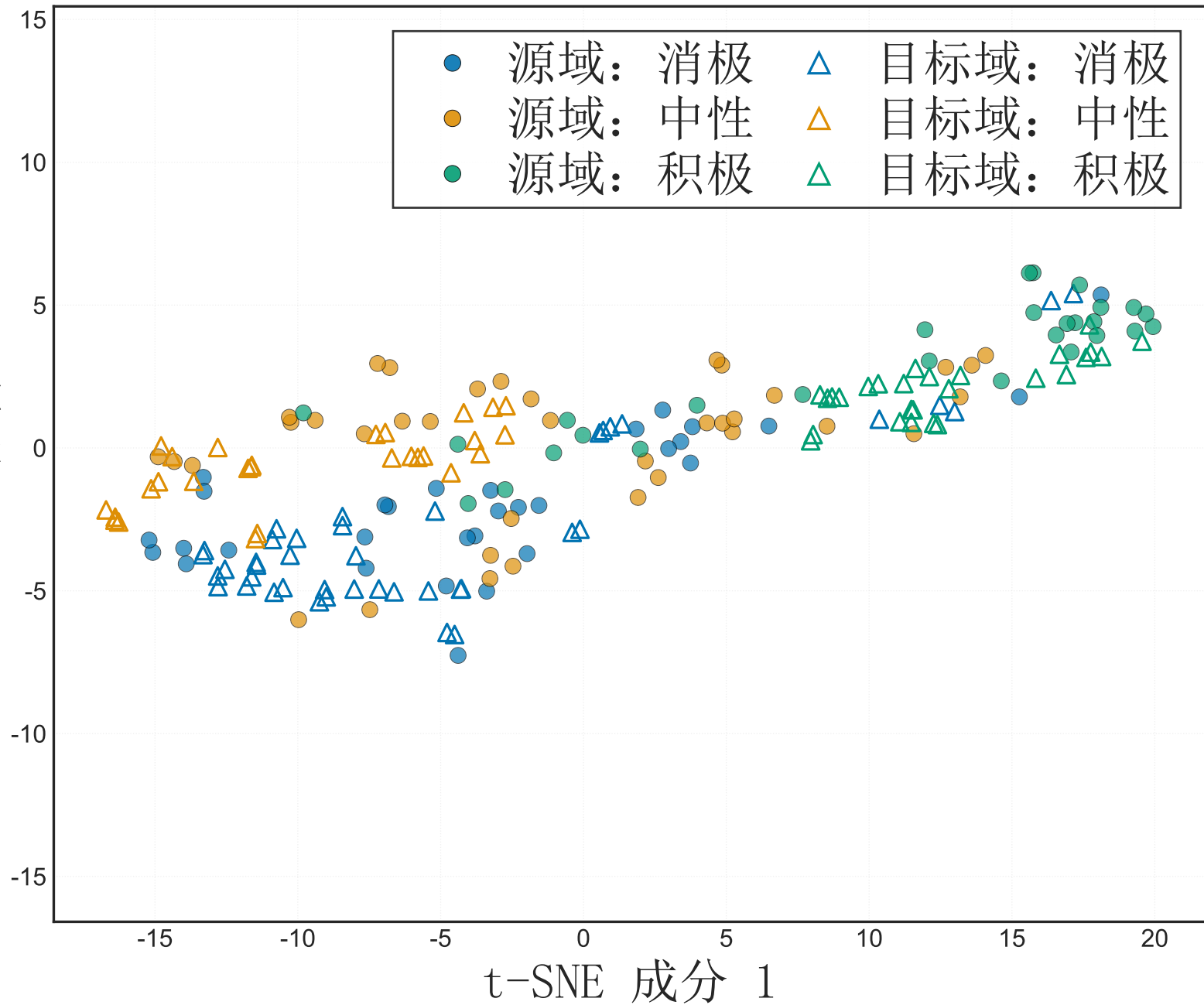
t-SNE 成分 2
