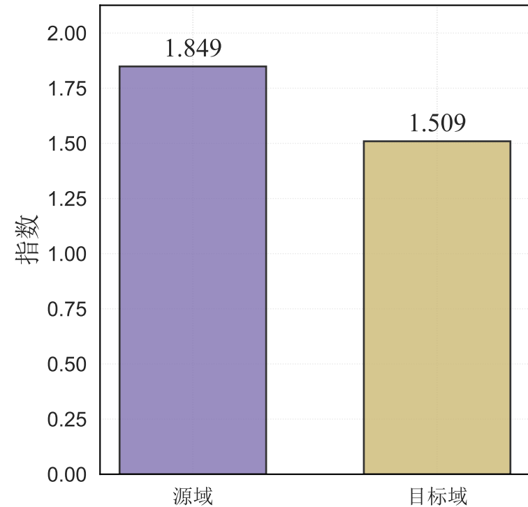
可分性指数
