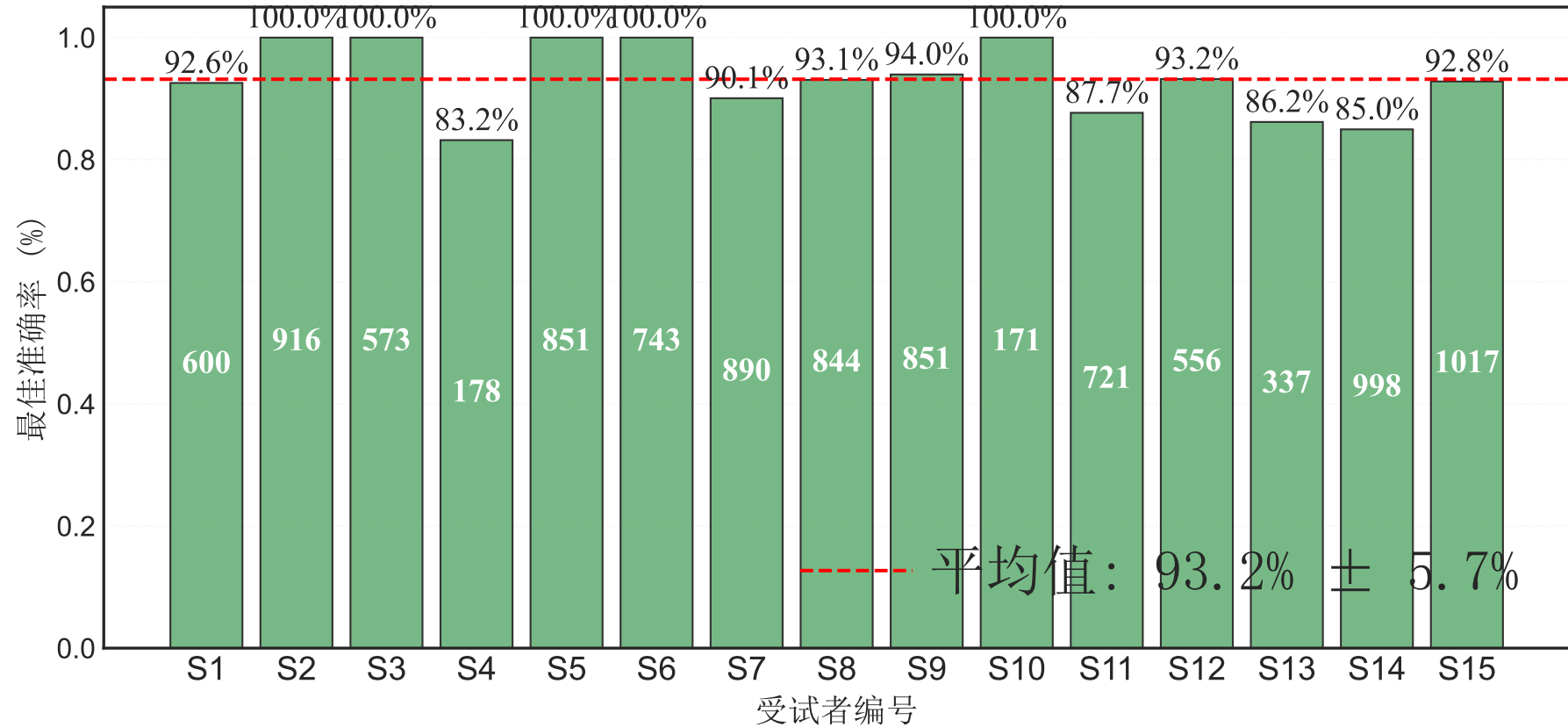
性能分析 - 会话 1 受试者最佳性能和最优轮次
