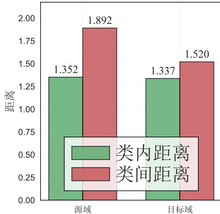
距离度量
