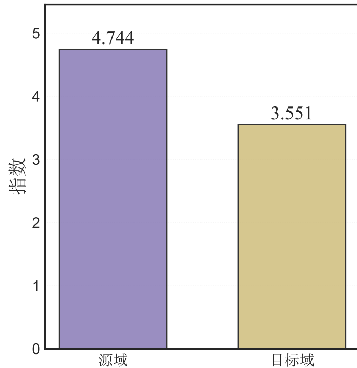
可分性指数
