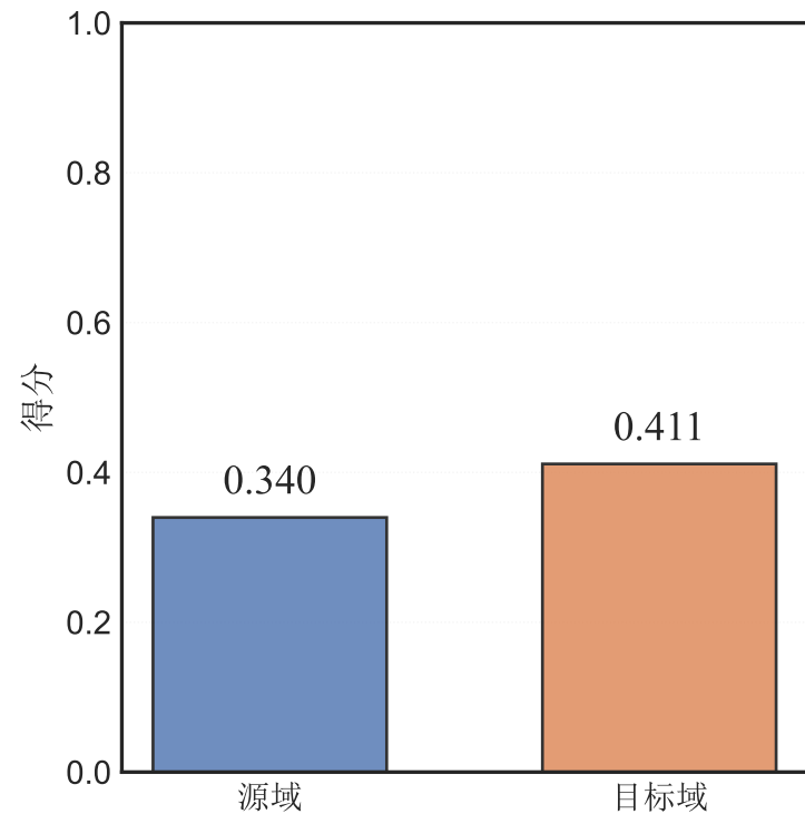
轮廓系数
