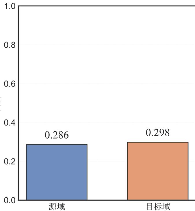
轮廓系数
