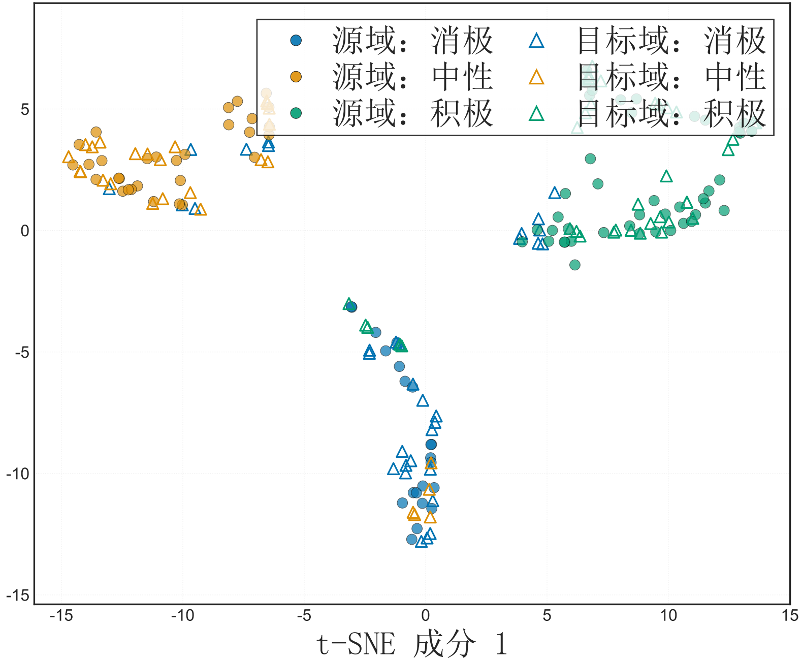
t-SNE 成分 2
