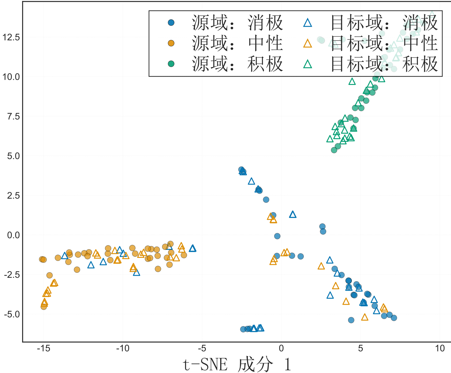
t-SNE 成分 2
