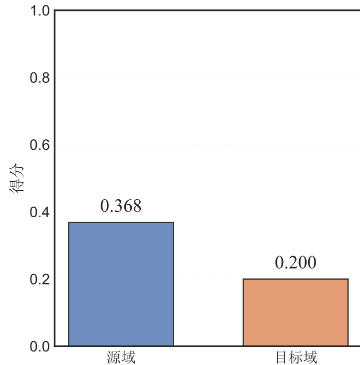
轮廓系数
