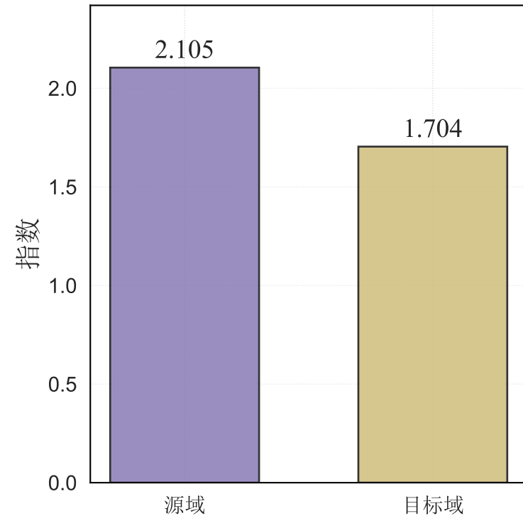
可分性指数
