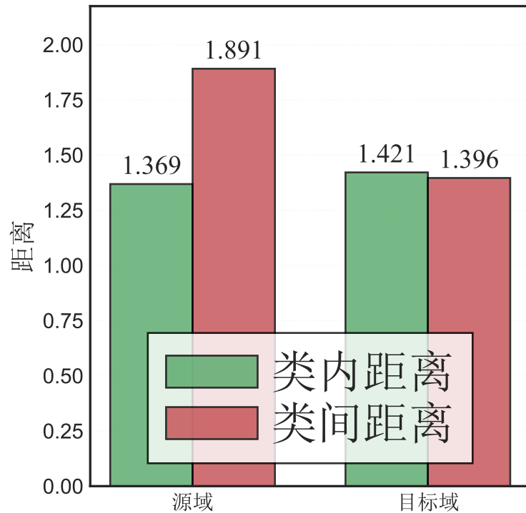
距离度量
