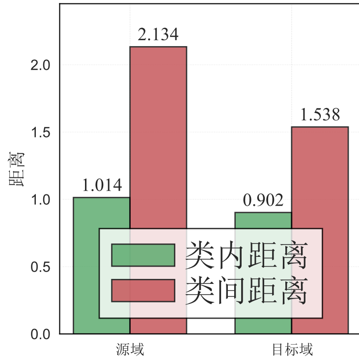
距离度量
