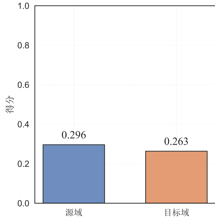
轮廓系数
