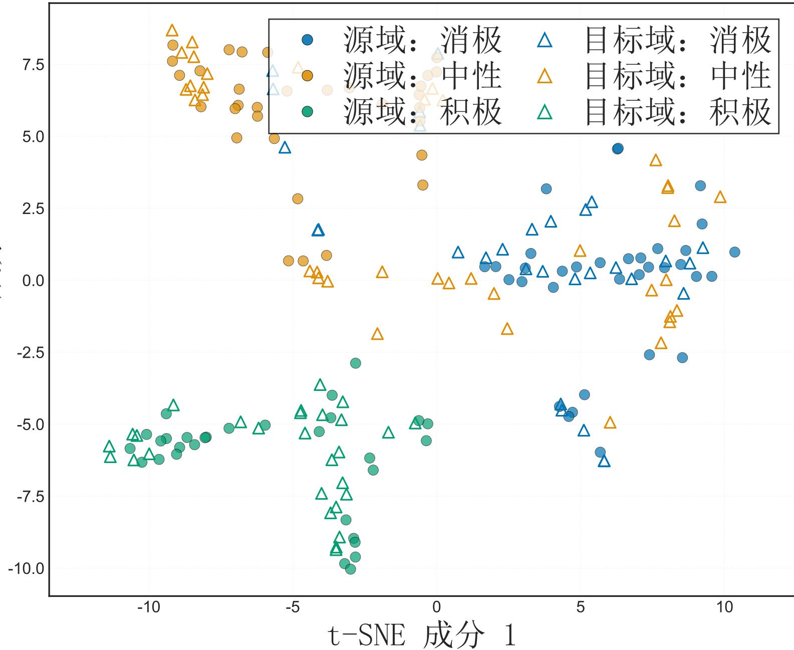
t-SNE 成分 2
