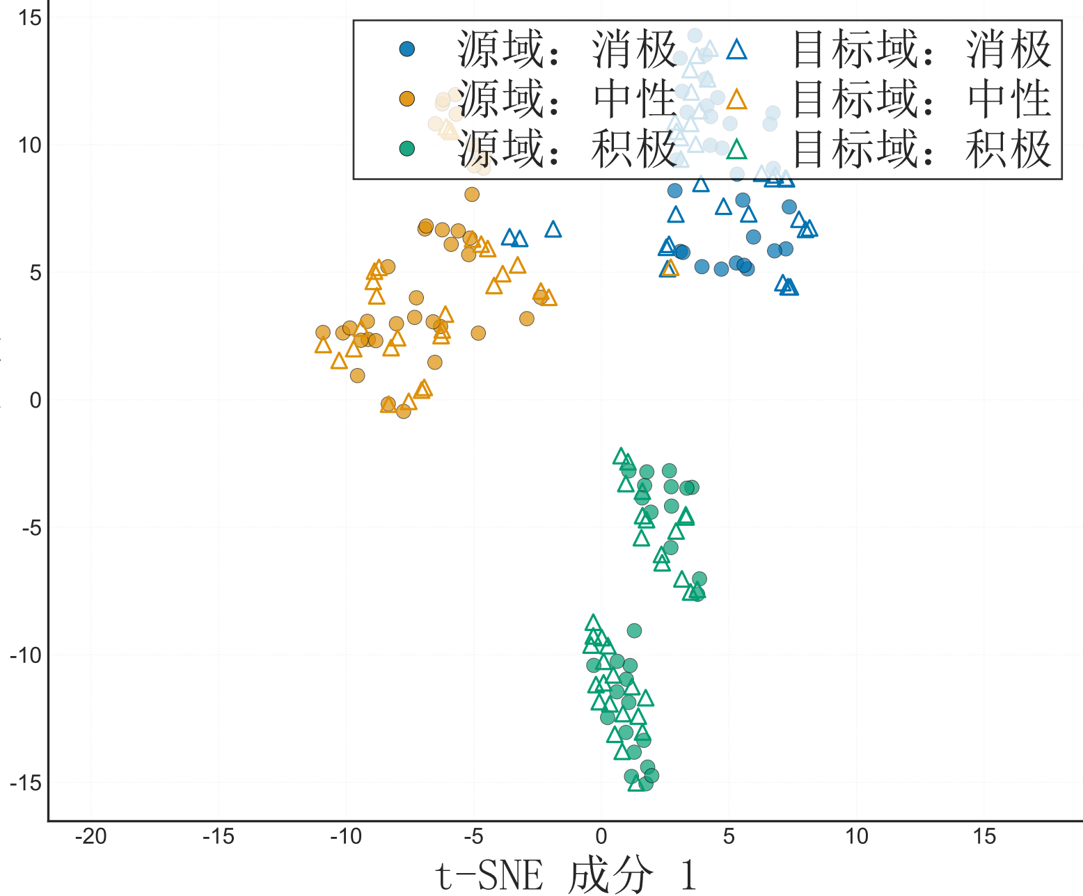
t-SNE 成分 2
