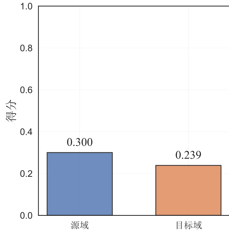
轮廓系数
