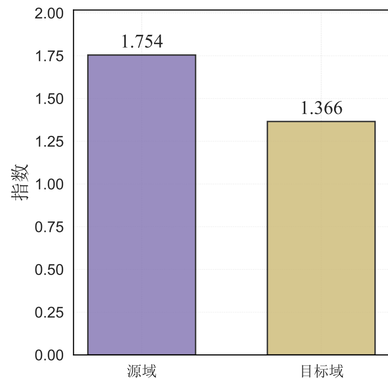
可分性指数
