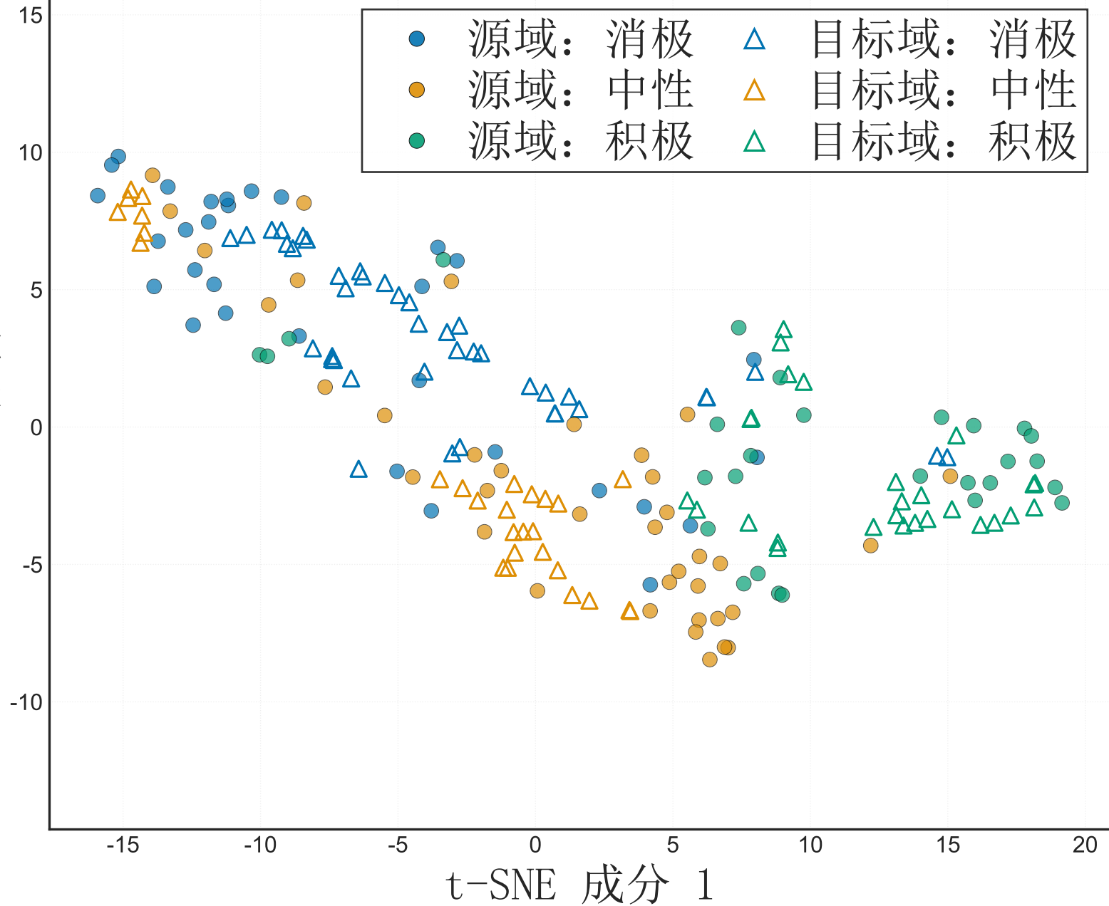
t-SNE 成分 2
