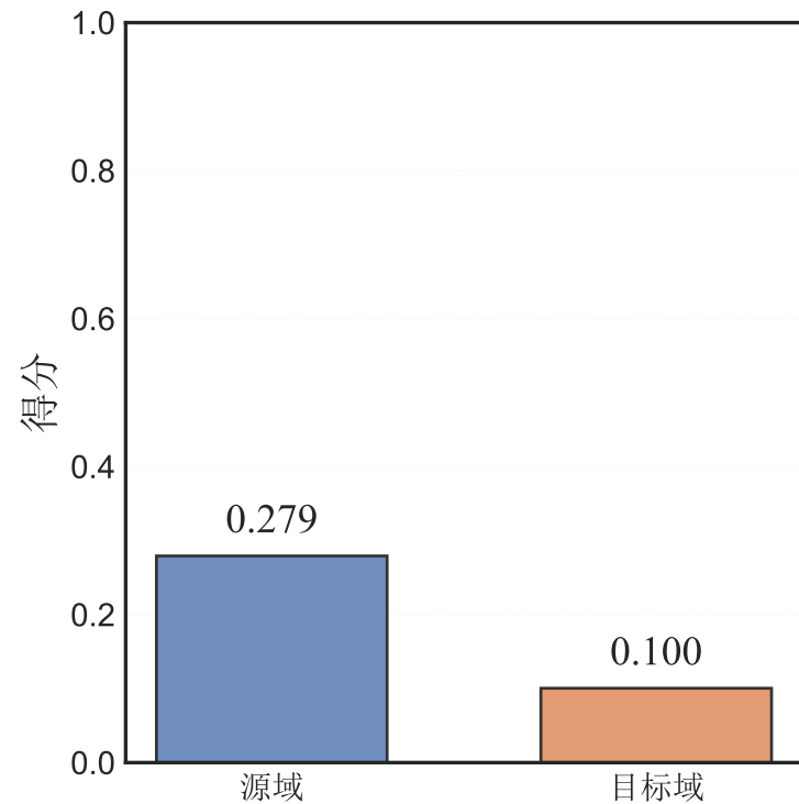
轮廓系数
