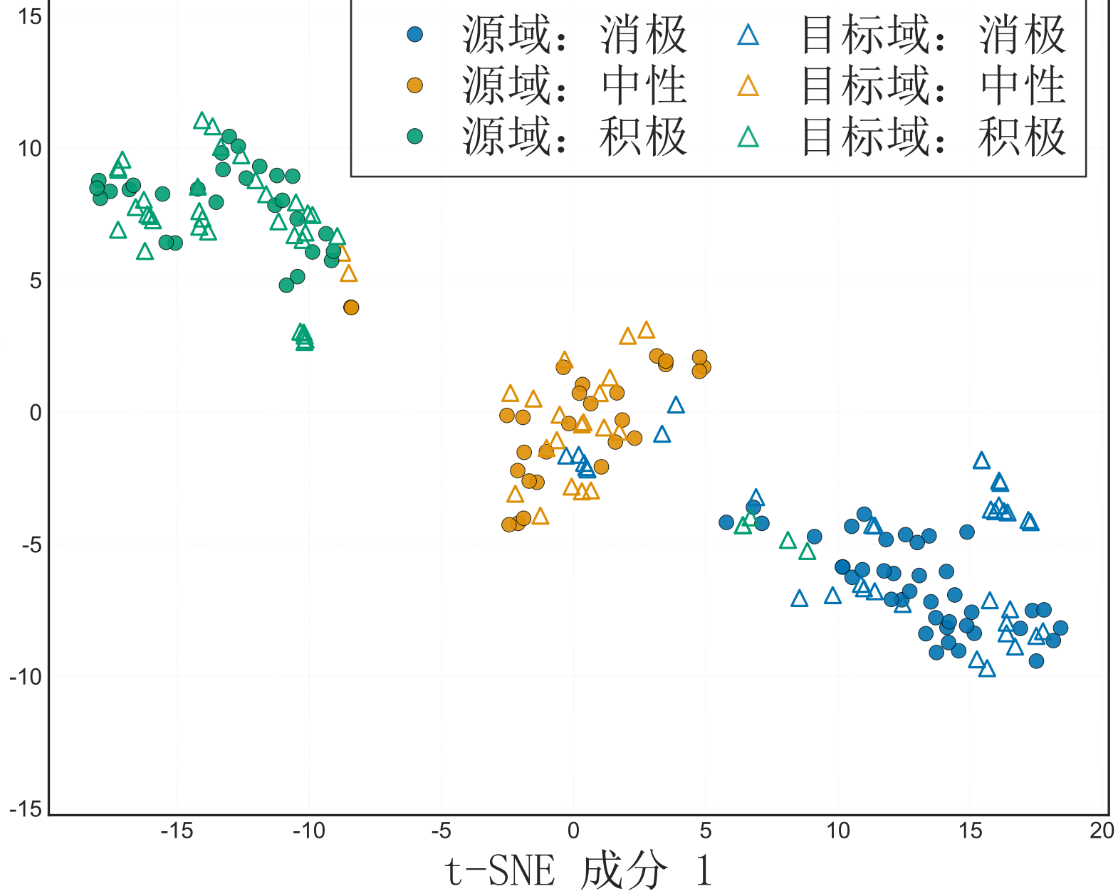
t-SNE 成分 2
