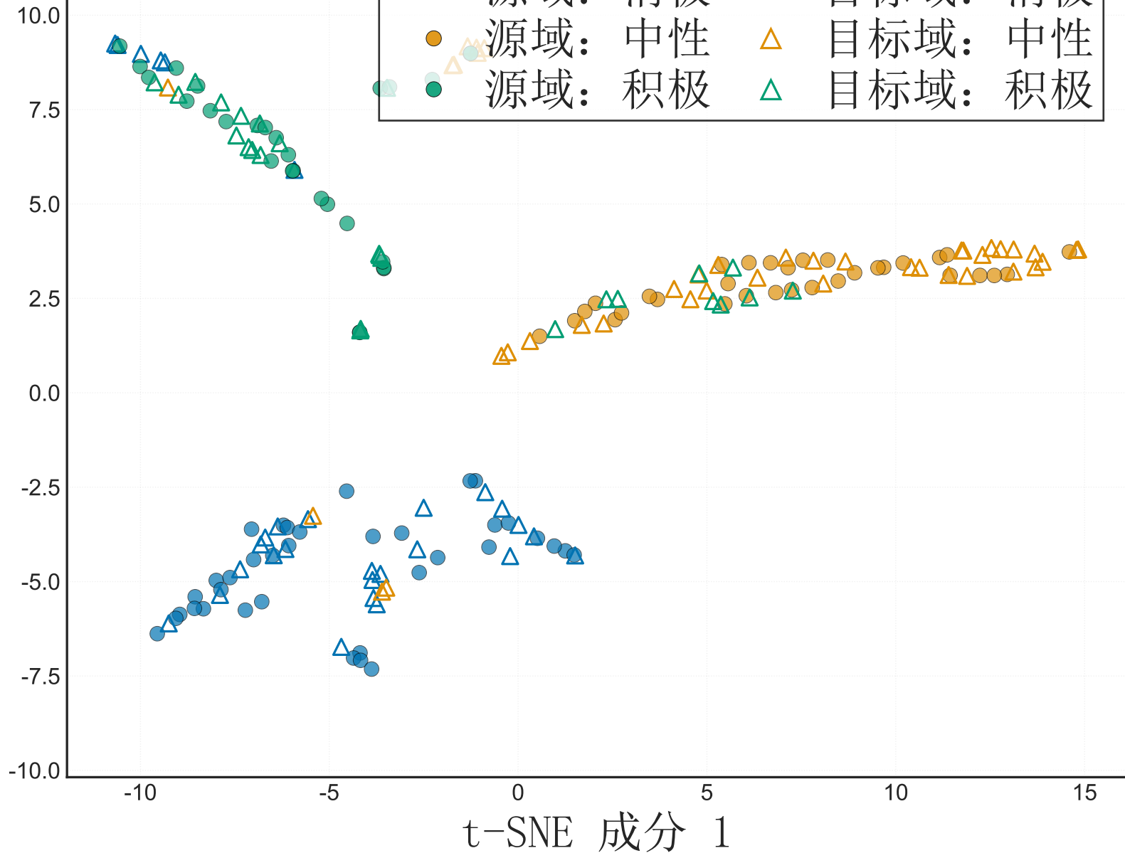
t-SNE 成分 2
