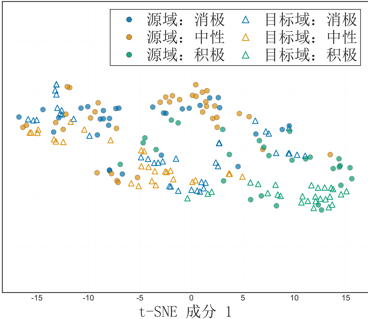
t-SNE 成分 2
