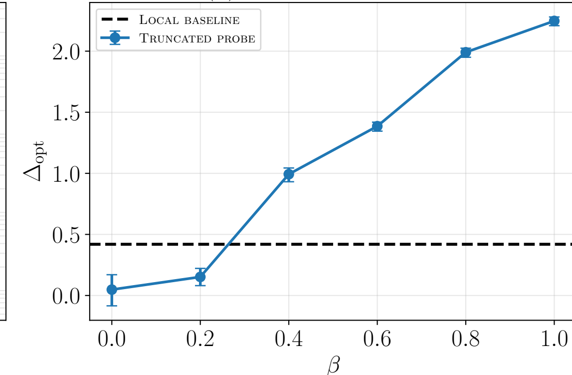
(d) Truncated : \alpha = 0.5
