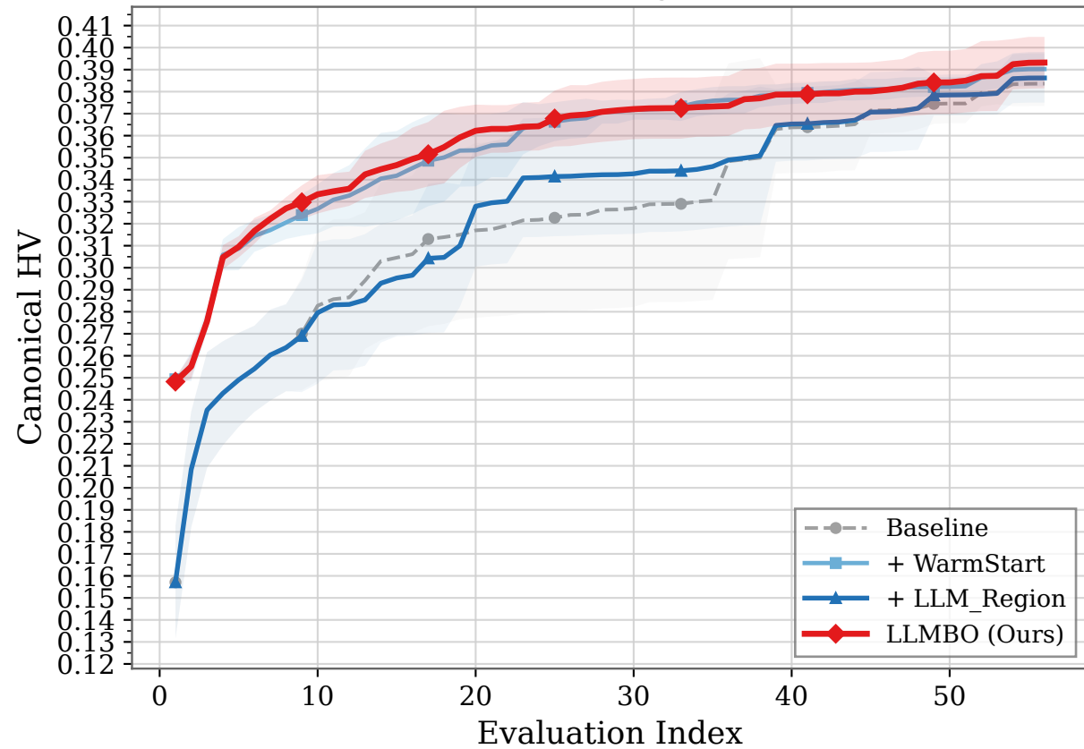
HV Convergence
