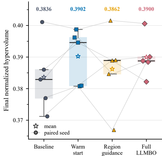
(b) Final-NHV distribution
