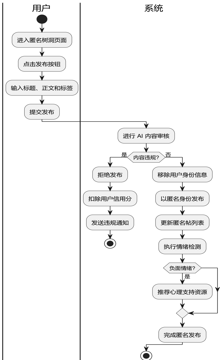
泳道图：匿名树洞流程
