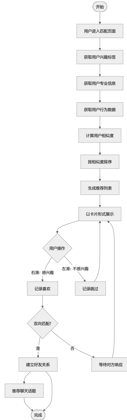
活动图：匹配交友流程
