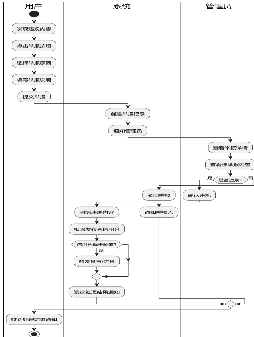
泳道图：举报与审核流程
