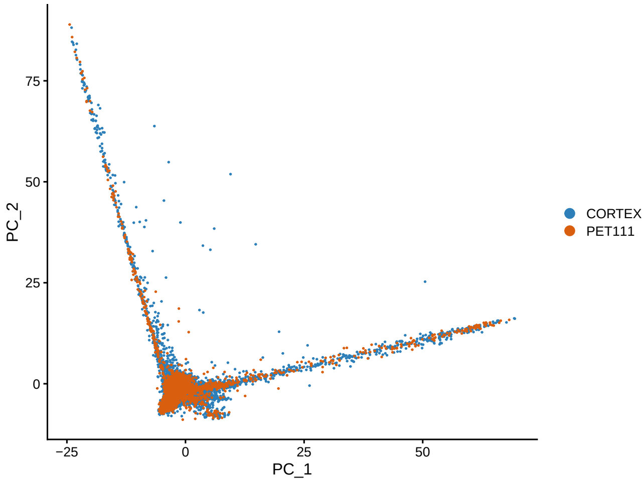
PCA (PC1 vs PC2)
