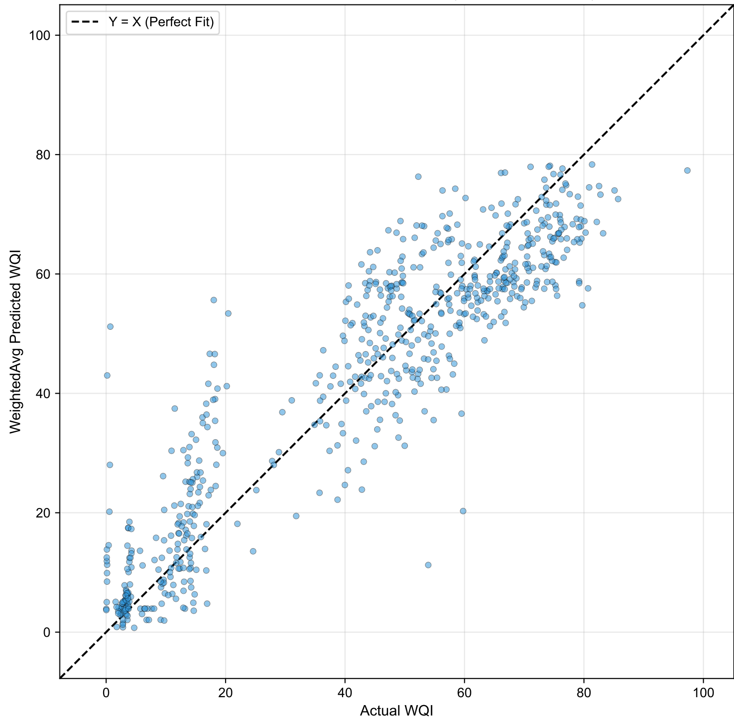
Ensemble Prediction vs Actual WQI (AKH, 657 Samples)
