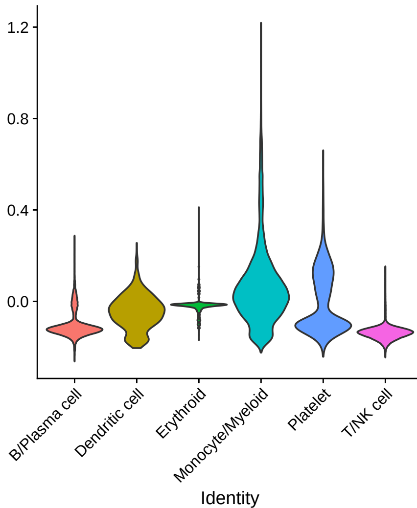
NestedRecurrent_score
