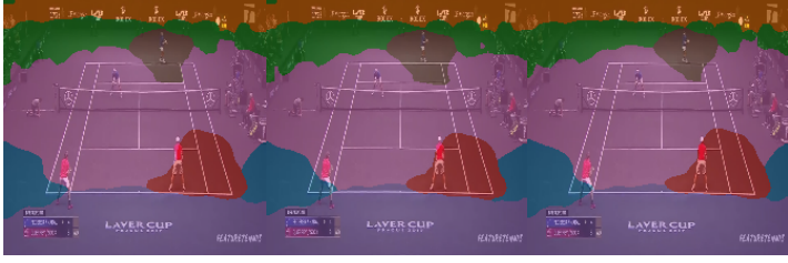
SlotContrast
