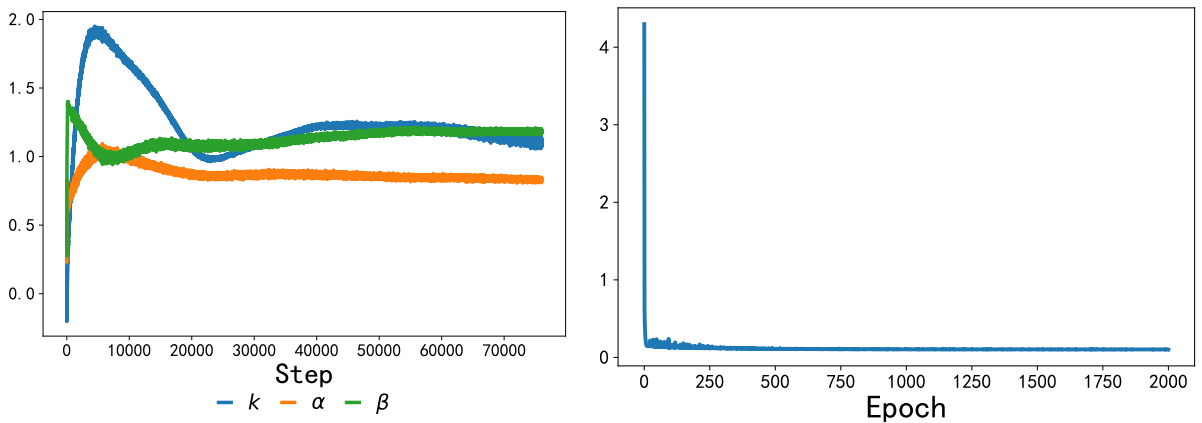
图 5.21 用 NAdam 求解经验模型 \text{LMSE}_{SDR} 时参数值（左）和损失函数值（右）变化趋势
