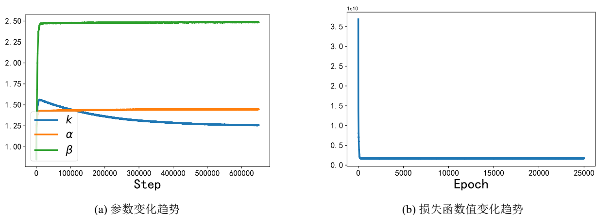
图 5.10 使用 NAdam 求解 SE 方程过程
