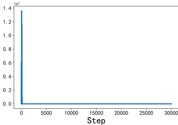
(a) PSO 求解减法模型 1
