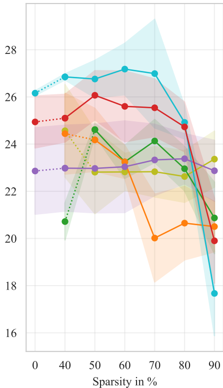
Dark Zurich
