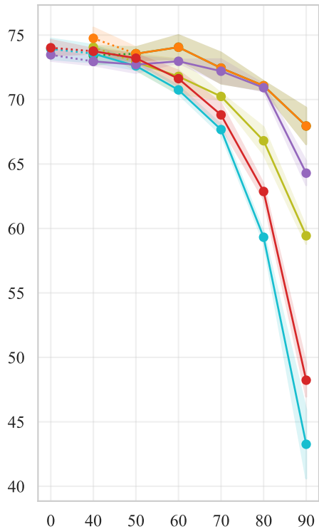
Cityscapes
