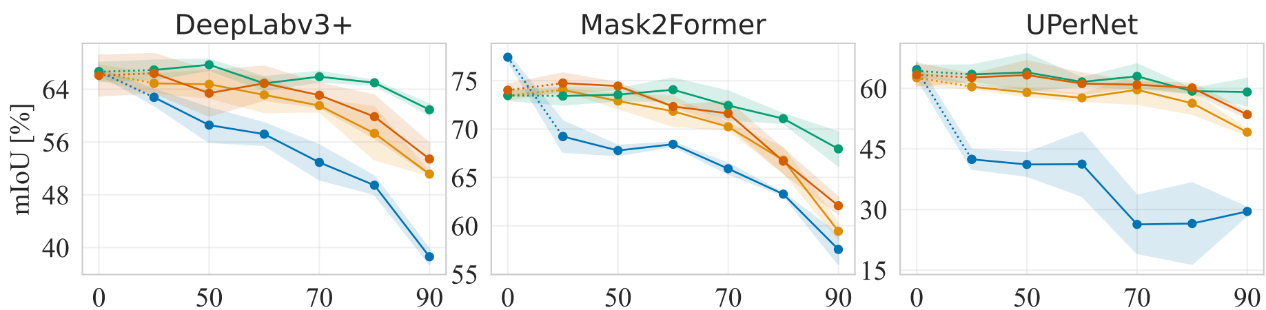
Cityscapes
