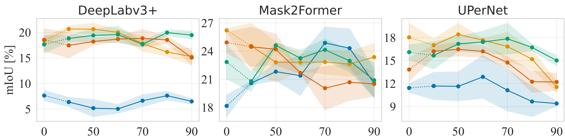
Dark Zurich
