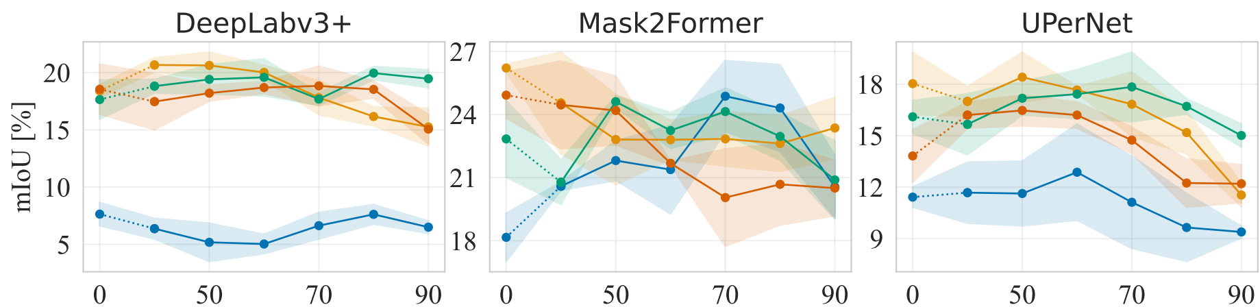
Dark Zurich
