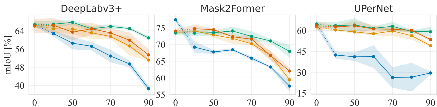
Cityscapes
