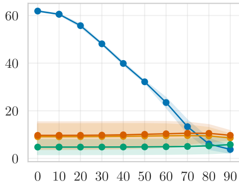
UPerNet
