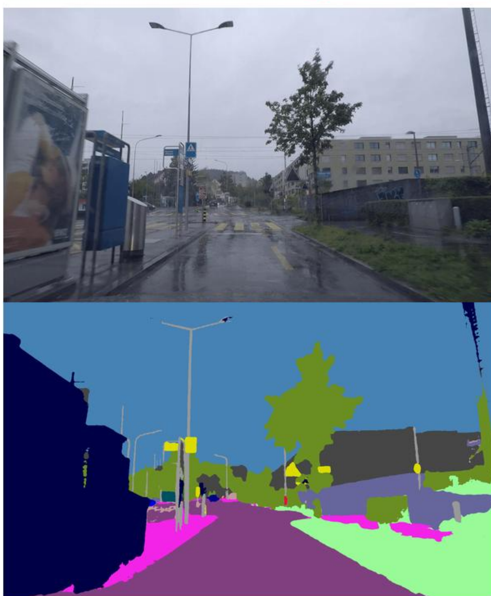
ACDC Rain
