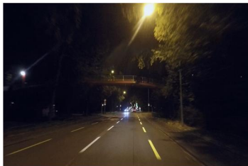
Dark Zurich
