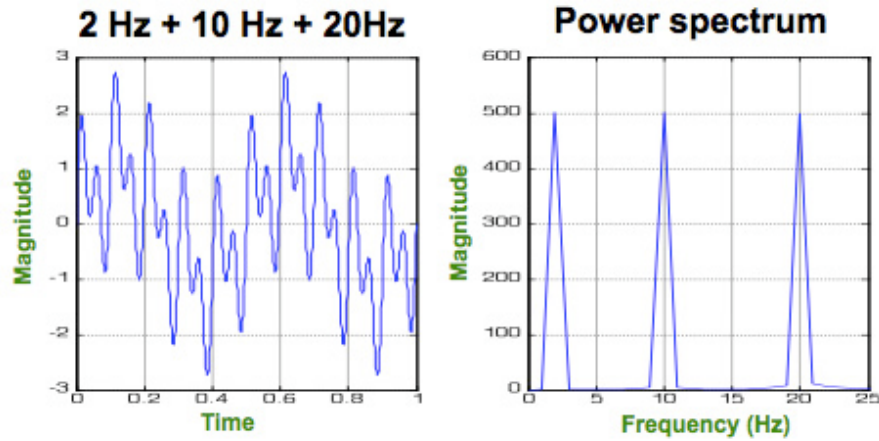
Figura 5.3: Ejemplo de señal en dominio temporal y frecuencial. Fuente: [61].
