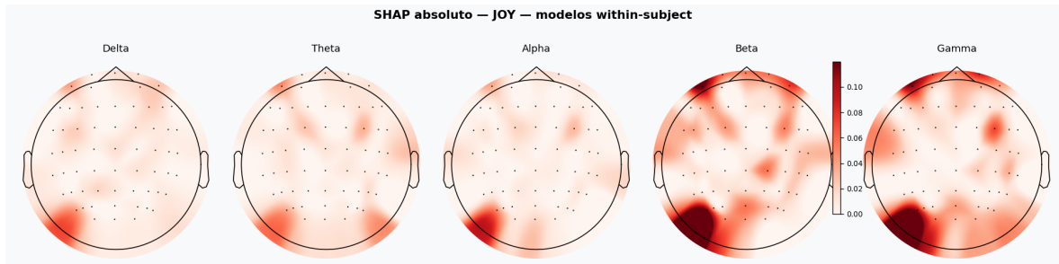
Figura 3.4: Ejemplo de topomaps por banda espectral para la clase alegría.
