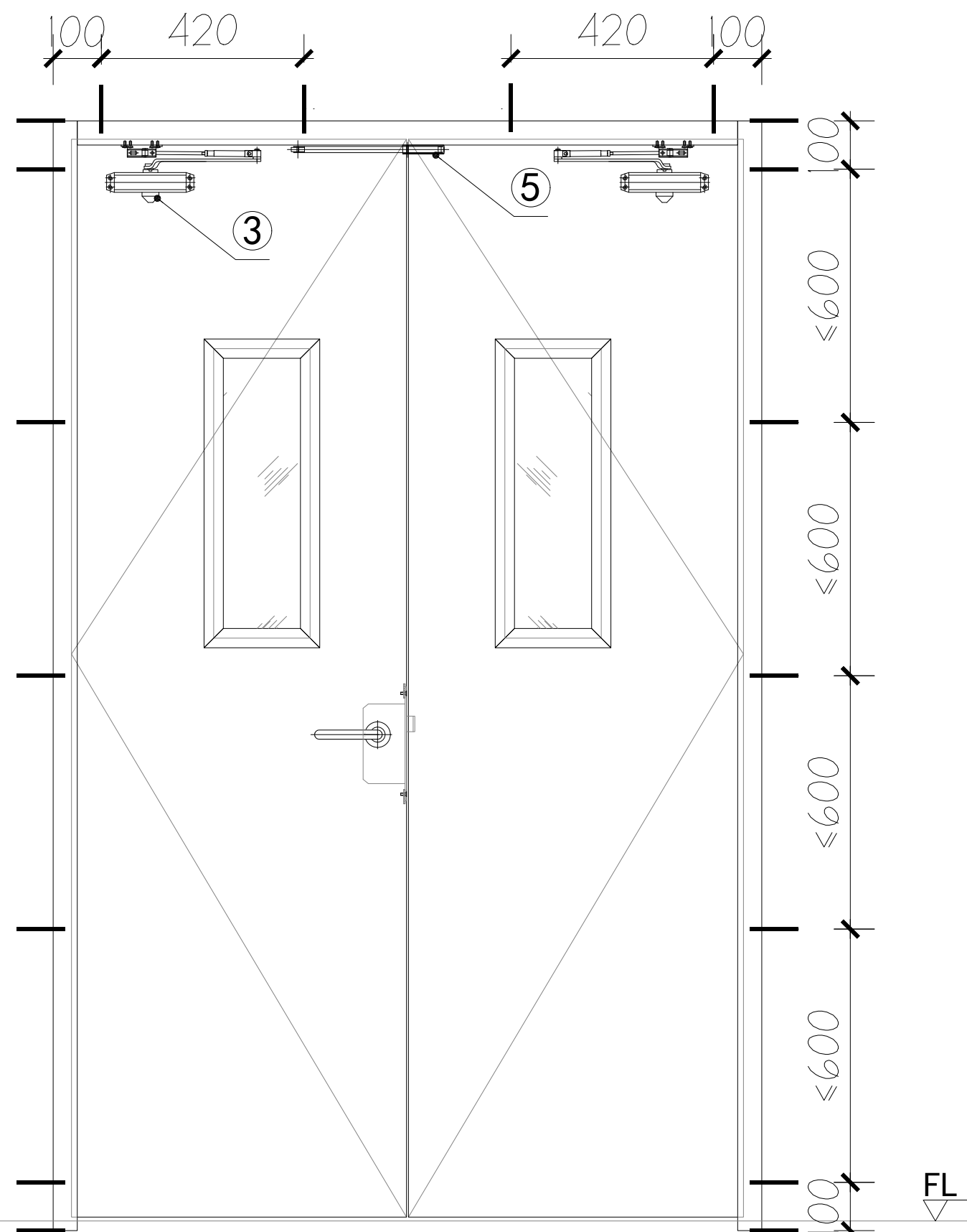
02 门体立面图（推侧） 1:20
