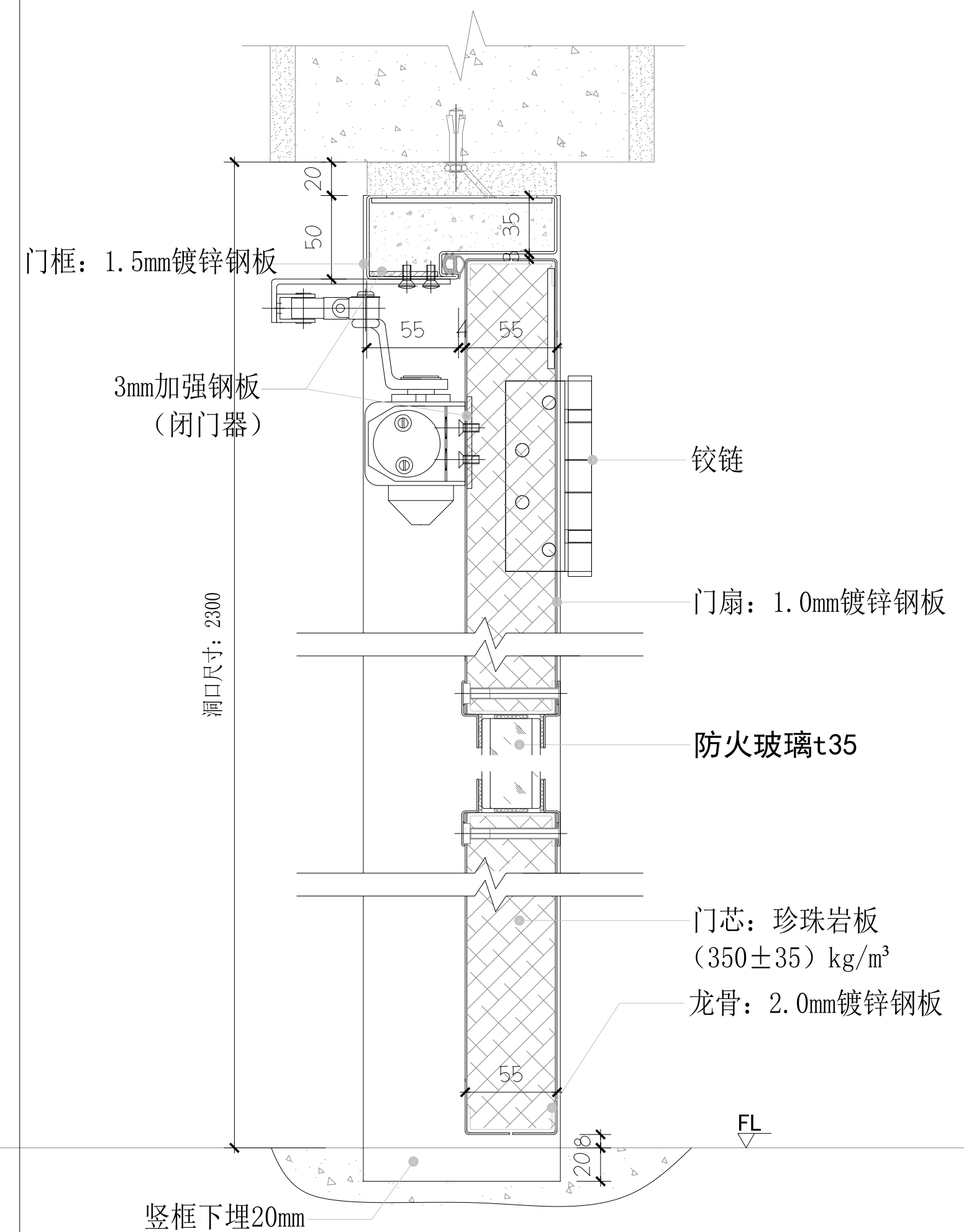
03 门体竖剖图 1:5
