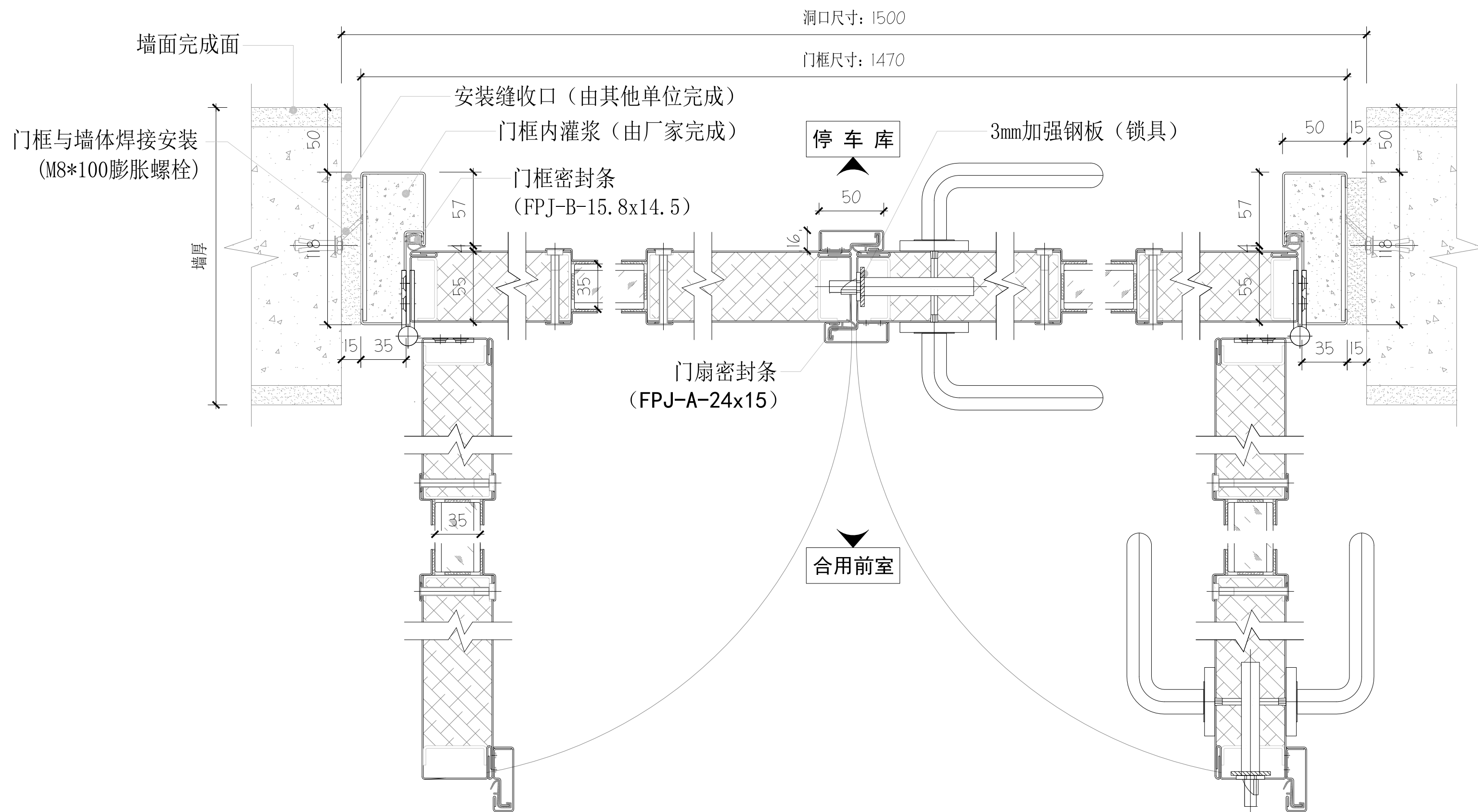
04 门体横剖图 1:5
