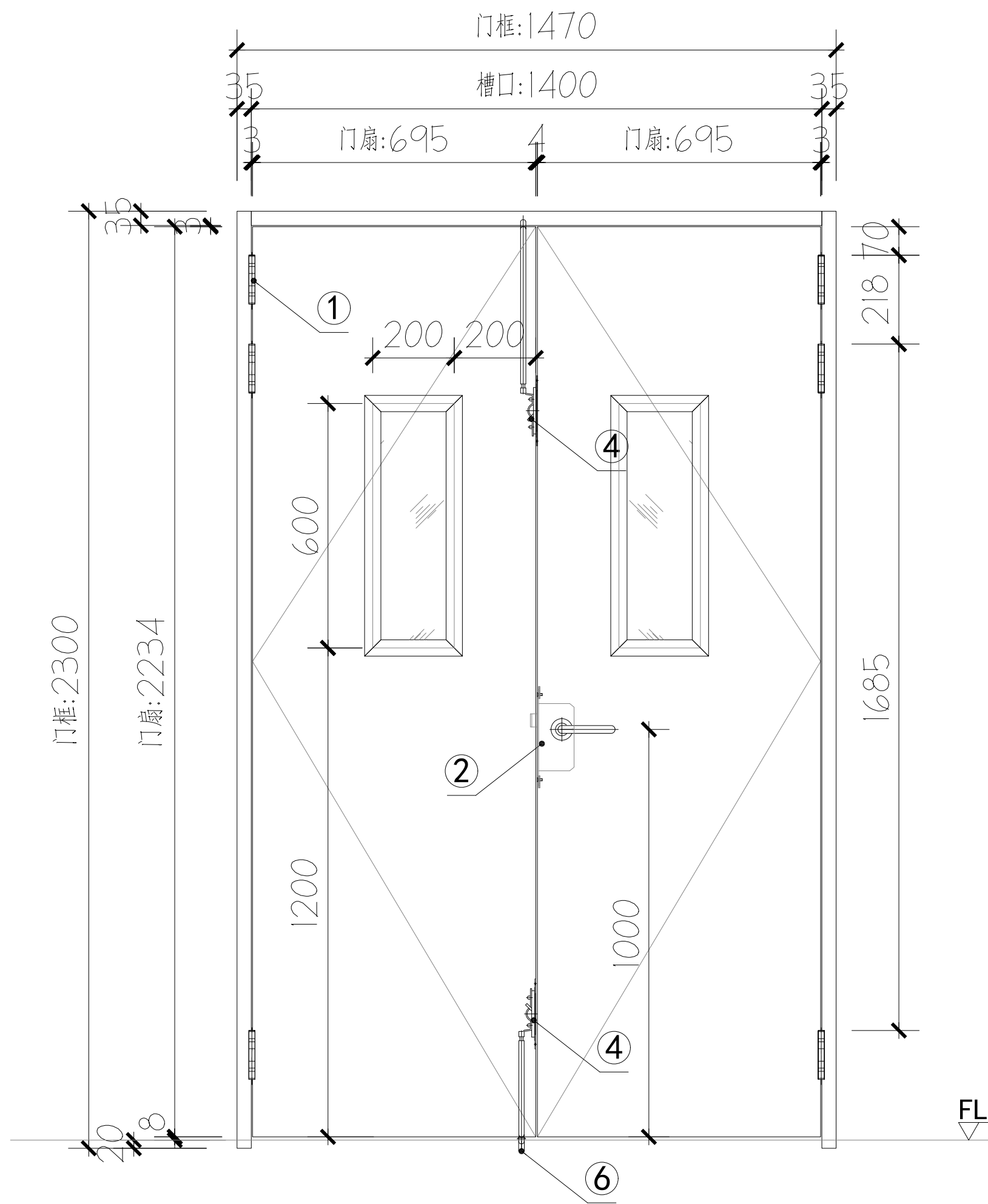
01 门体立面图（拉侧） 1:20
