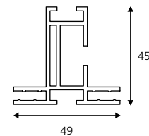
Profilquerschnitt
