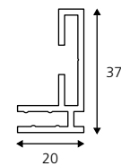
Profilquerschnitt
