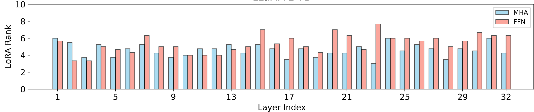
LLaMA-2-7B
