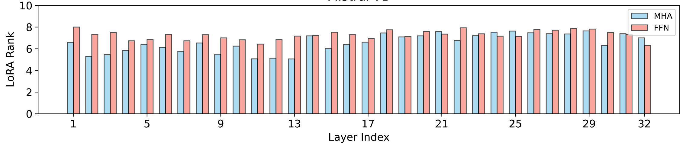
Mistral-7B
