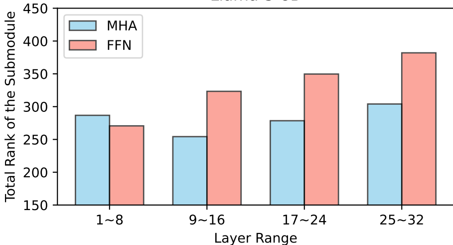
Llama-3-8B
