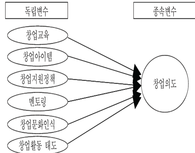
〈그림 1〉 연구모형
