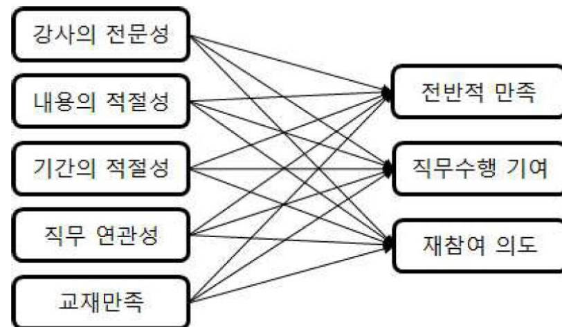
[그림 1] 연구모형
