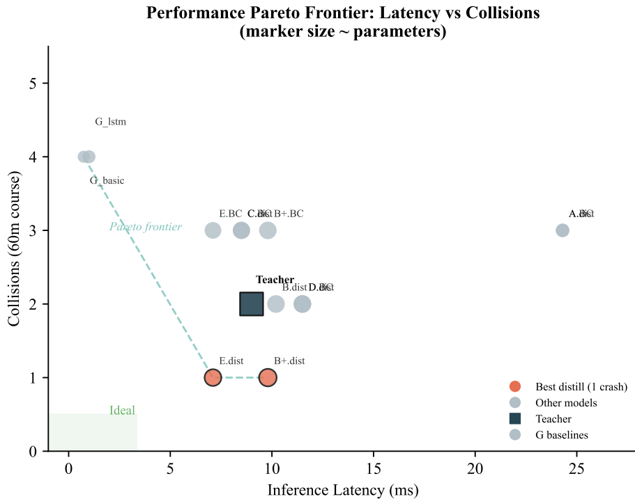
Figure 4.4 性能帕累托前沿：推理延迟与碰撞次数。标记面积为参数量比例。E.dist 和 B+.dist 以 1 次碰撞位于帕累托前沿，G_basic 以极低延迟（0.74ms）但 4 次碰撞位于前沿的另一端。实心标记 = 蒸馏模型。
