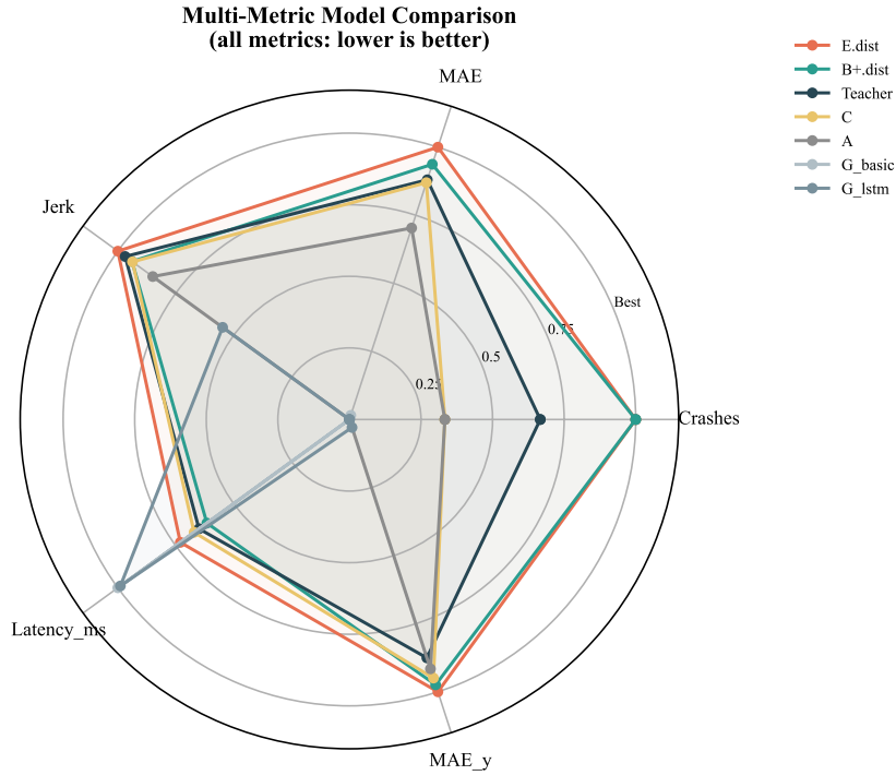
Figure 4.2 多维度模型性能雷达图。所有指标均归一化至 [0,1] 区间（外圈 = 最优），涵盖碰撞次数、速度追踪误差（MAE）、控制平滑度（jerk）、推理延迟和横向偏差五个维度。E.dist 在除推理延迟外的所有维度上均处于外圈区域。
