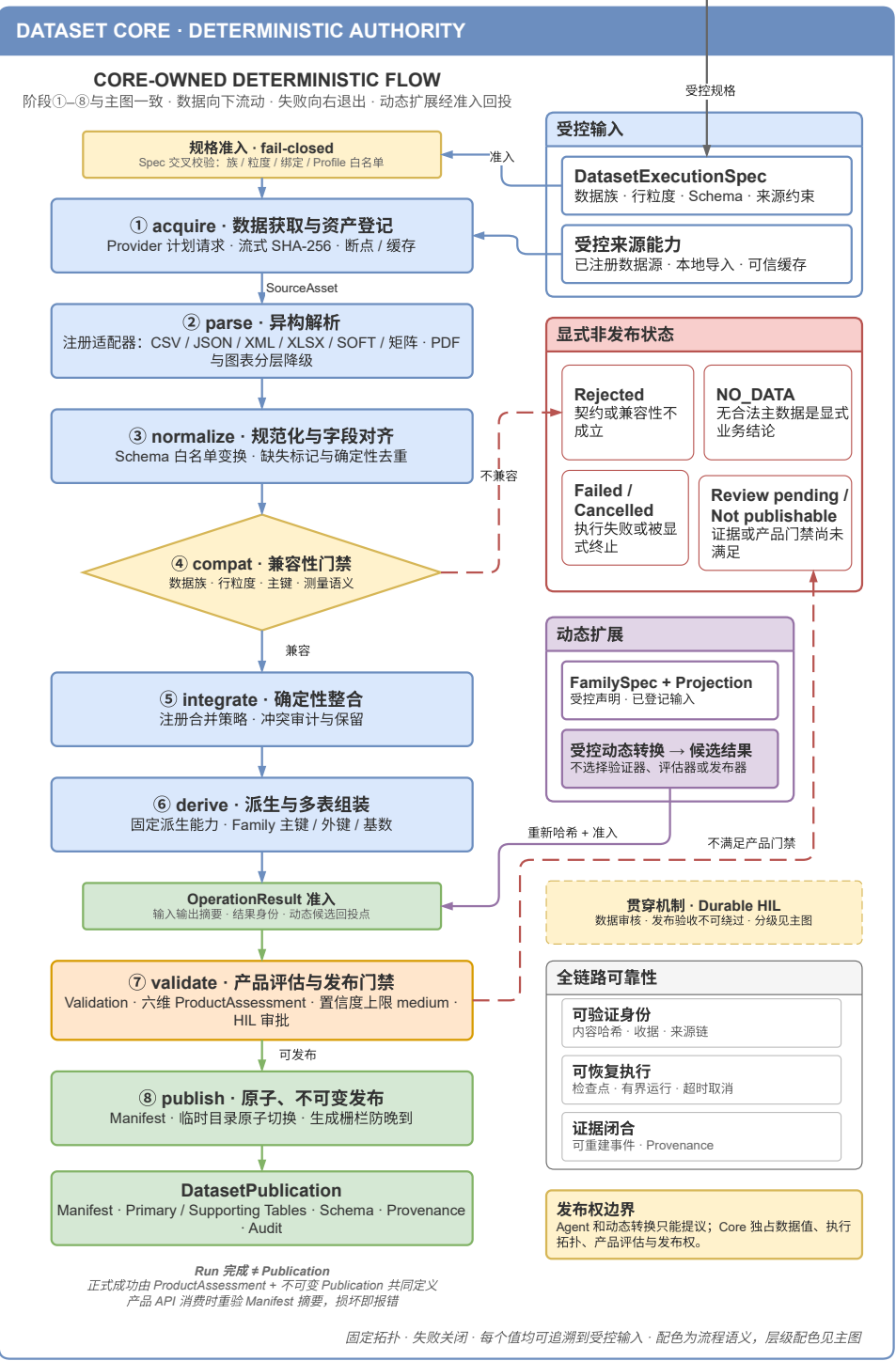
图 4.1: Dataset Core 确定性数据流详图
