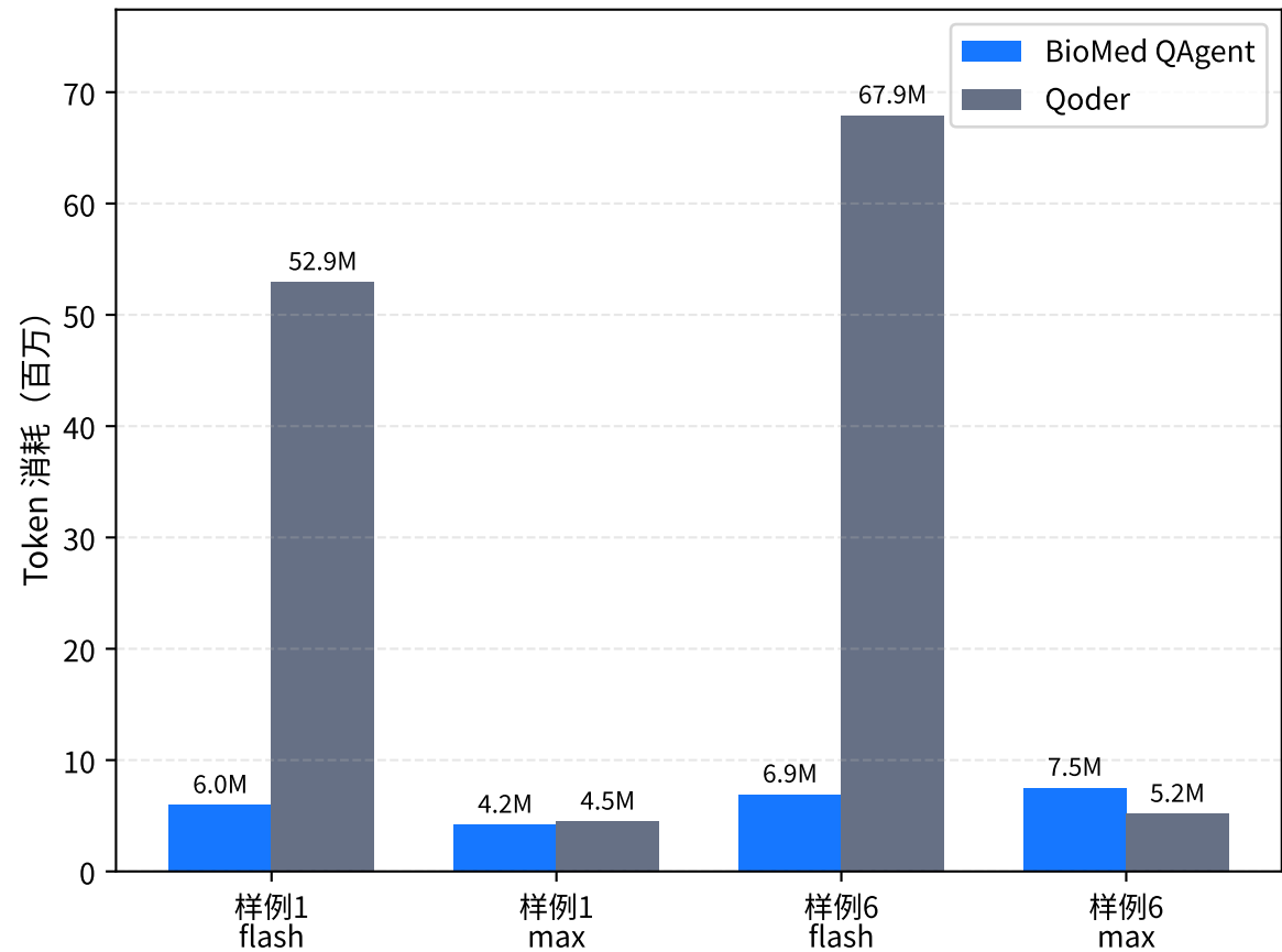
Token 消耗（样例1 / 样例6）
