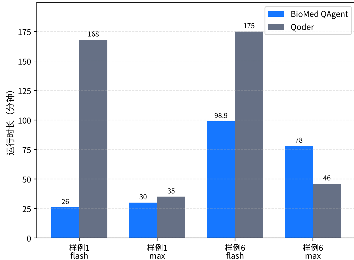
运行时长（样例1 / 样例6）
