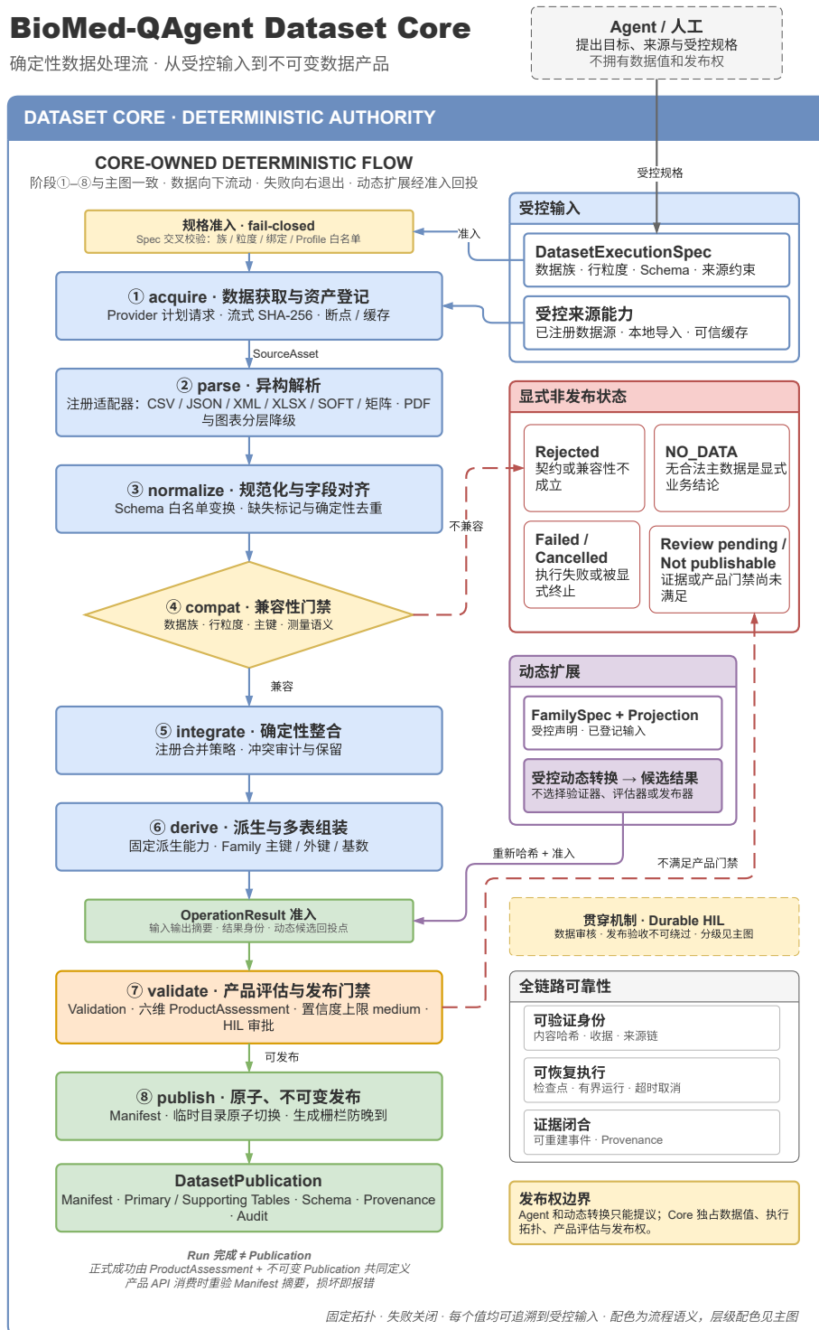
图 4.1: Dataset Core 确定性数据流详图
