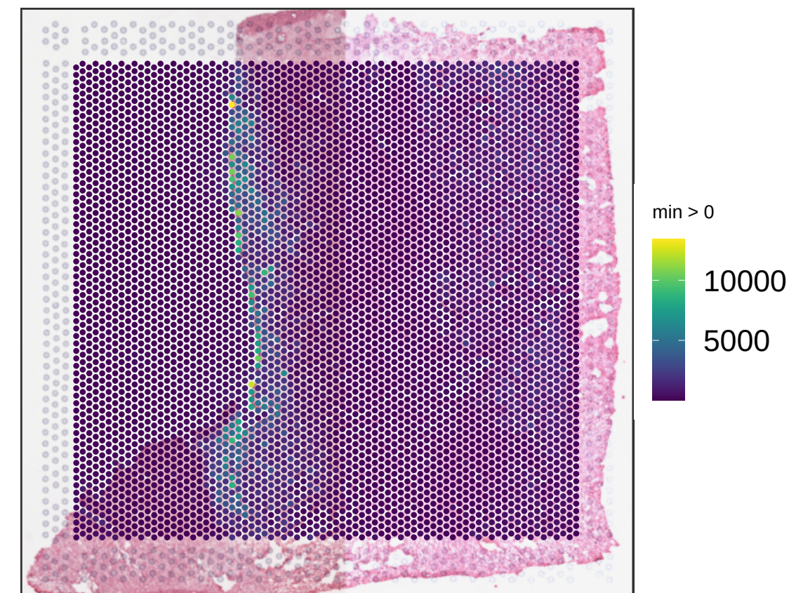
V13B23-280_D1 sum_umi
