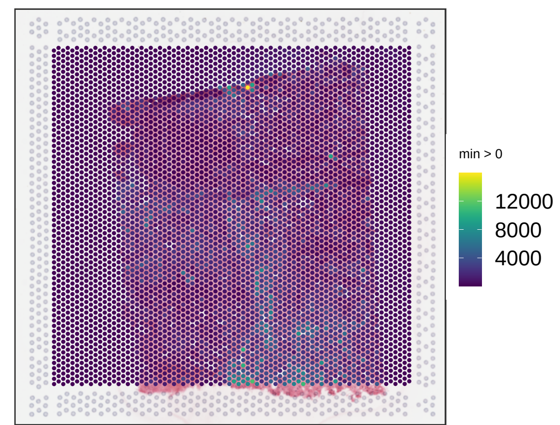
V13B23-281_D1 sum_umi
