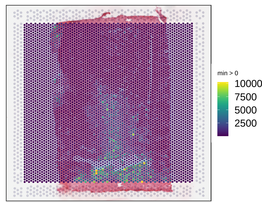
V13B23-281_C1 sum_umi
