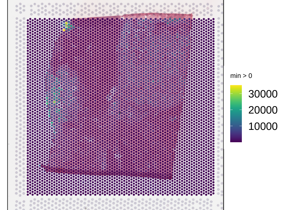
V13B23-285_D1 sum_umi
