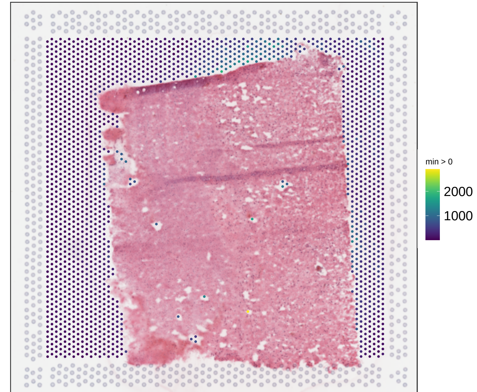
V13B23-281_D1 sum_umi
