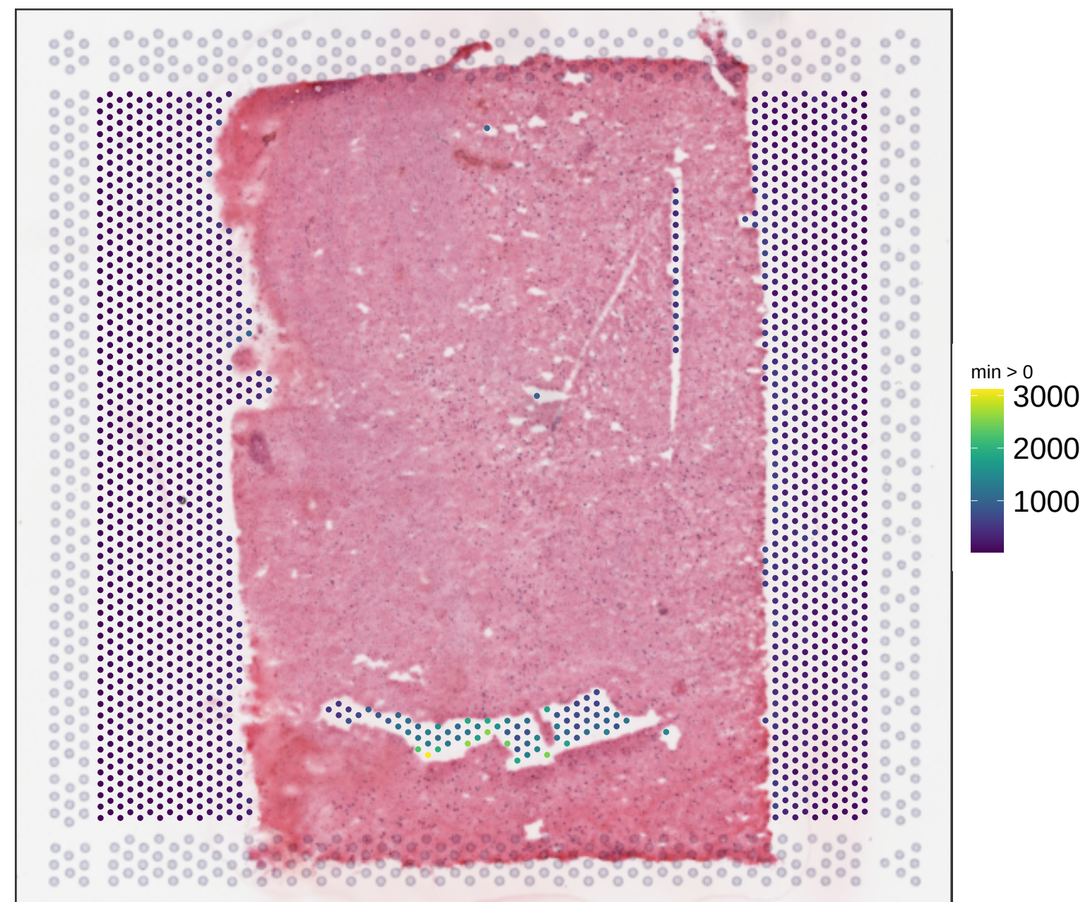
V13B23-281_C1 sum_umi
