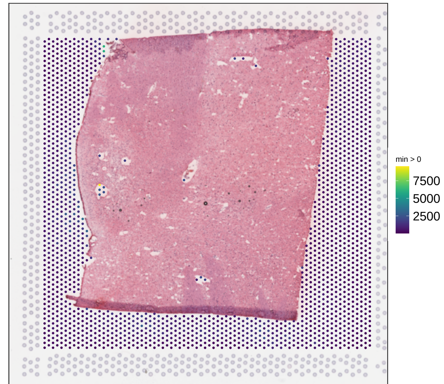
V13B23-285_D1 sum_umi
