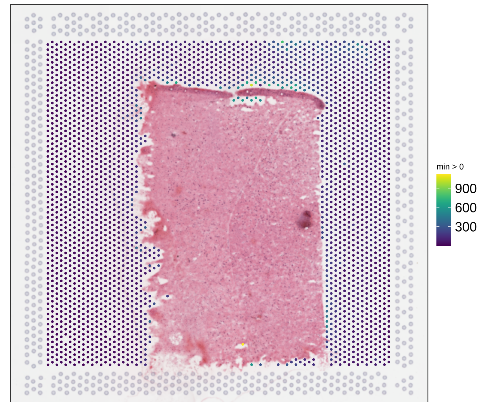
V13B23-281_A1 sum_umi
