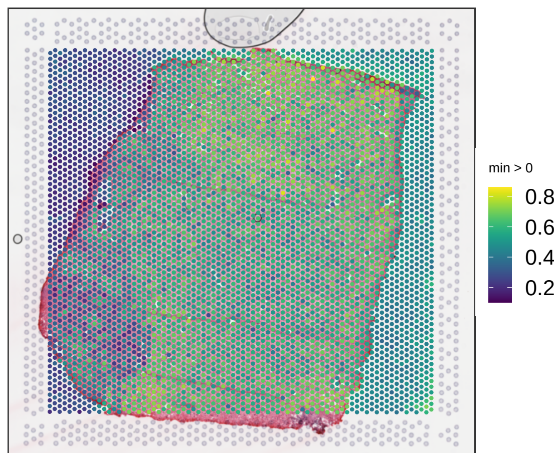
V13B23-285_A1 expr_chrm_ratio
