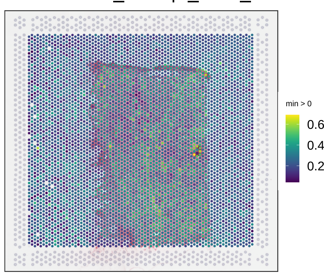
V13B23-281_A1 expr_chrm_ratio
