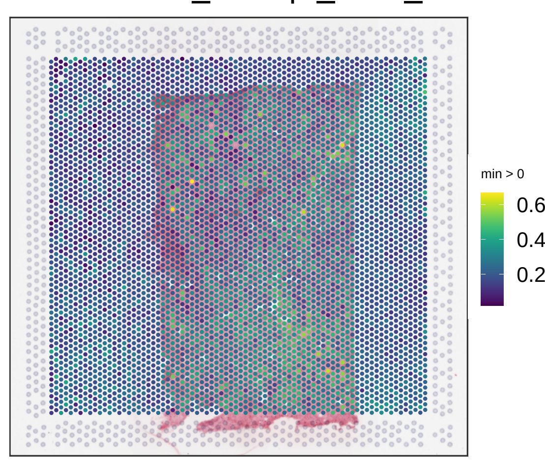
V13B23-281_B1 expr_chrm_ratio
