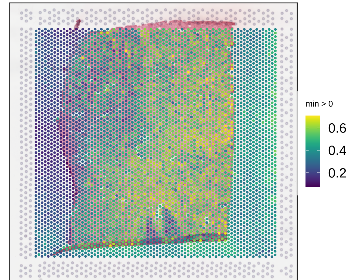
V13B23-285_C1 expr_chrm_ratio
