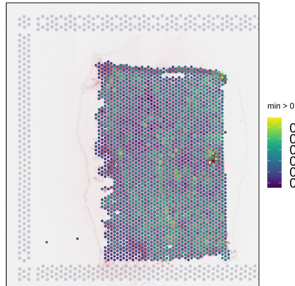
V13B23-281_A1 expr_chrm_ratio
