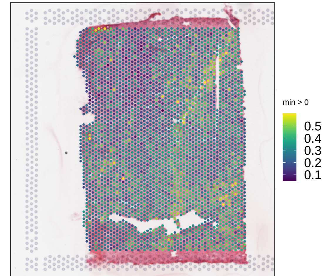
V13B23-281_C1 expr_chrm_ratio
