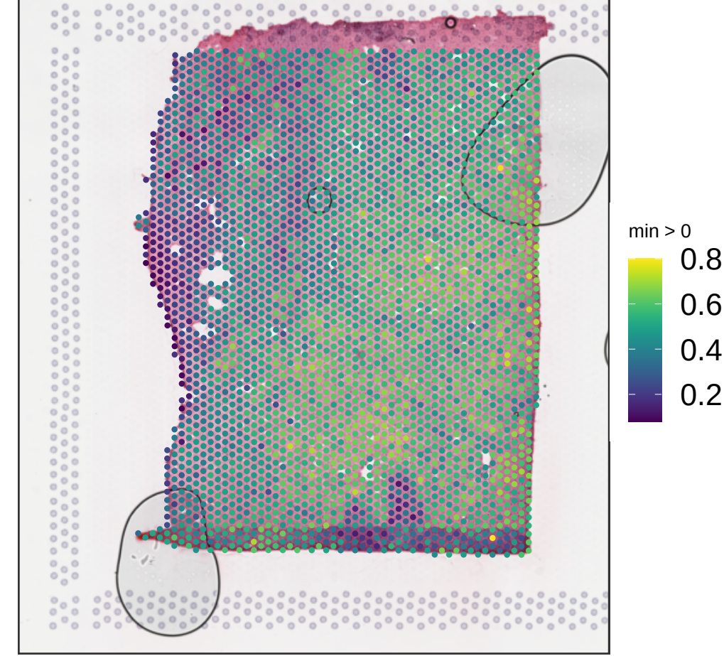
V13B23-285_B1 expr_chrm_ratio
