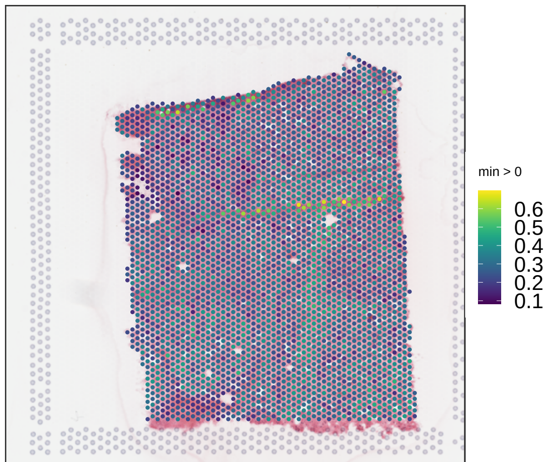
V13B23-281_D1 expr_chrm_ratio
