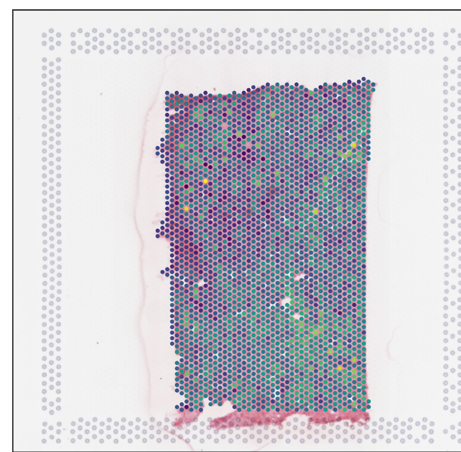
V13B23-281_B1 expr_chrm_ratio
