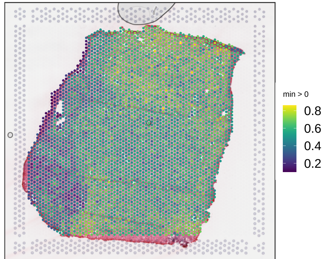
V13B23-285_A1 expr_chrm_ratio
