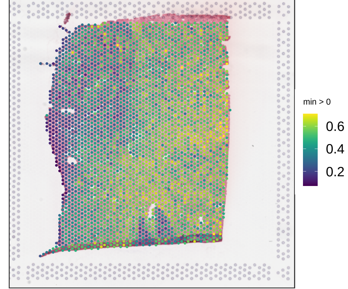
V13B23-285_C1 expr_chrm_ratio
