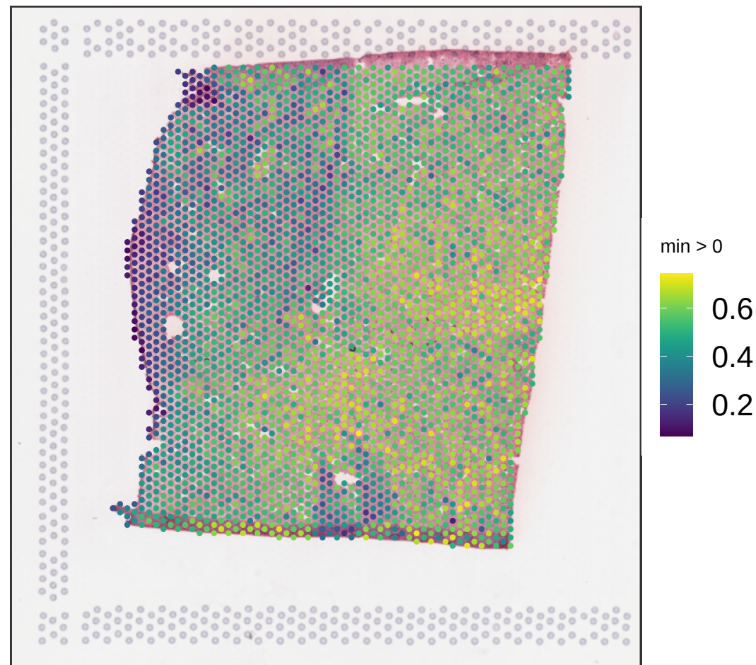
V13B23-285_D1 expr_chrm_ratio
