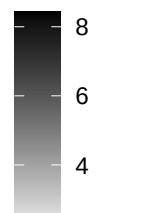
sum_gene_log
