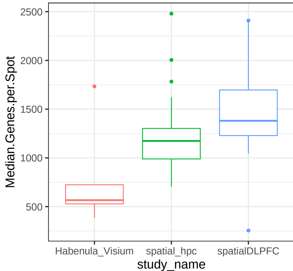
Median.Genes.per.Spot
