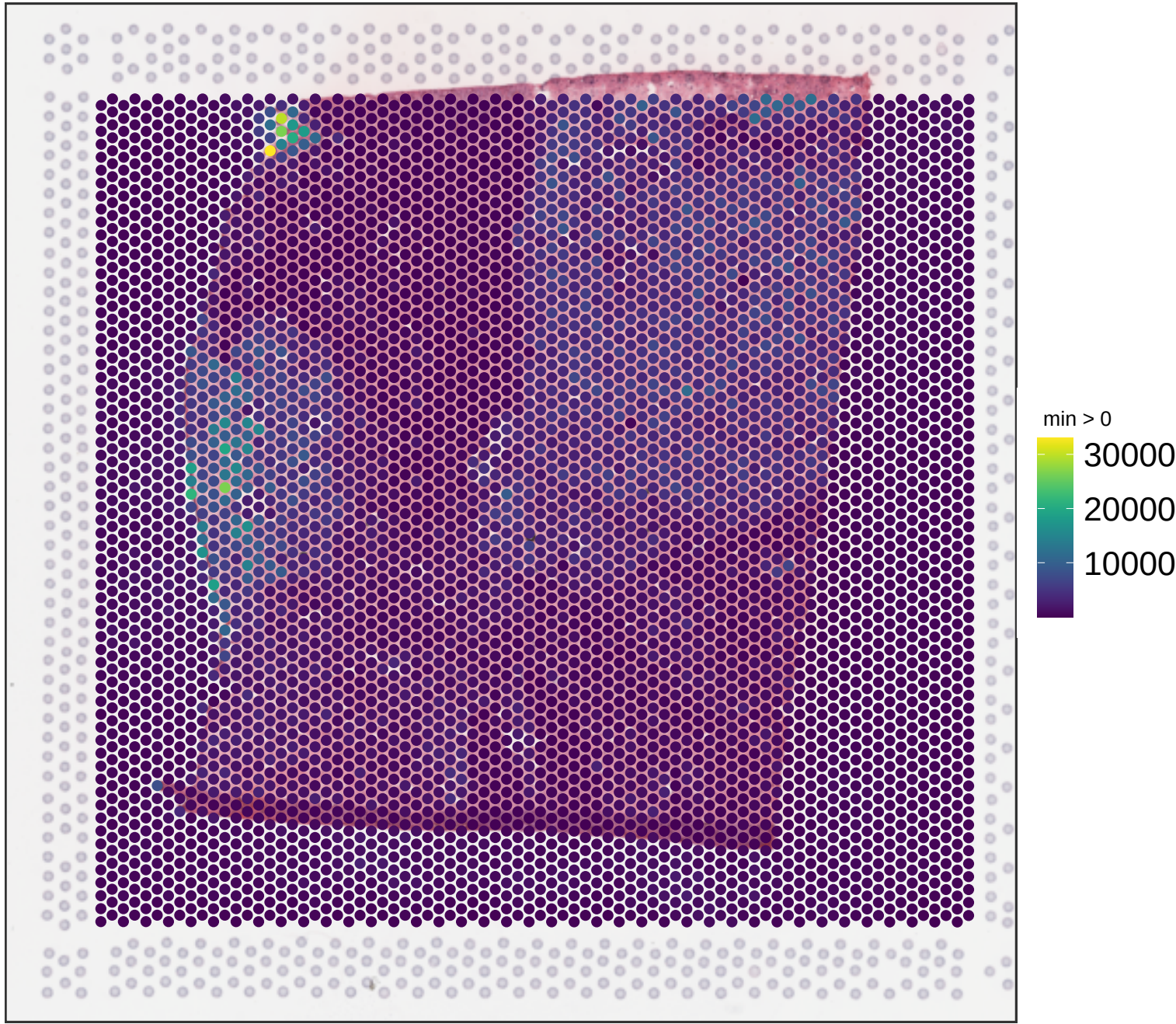
V13B23-285_D1 sum_umi
