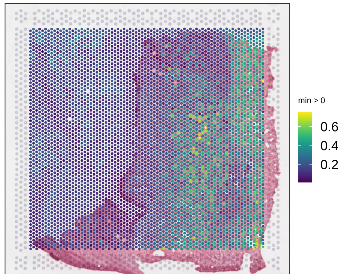
V13B23-280_B1 expr_chrM_ratio
