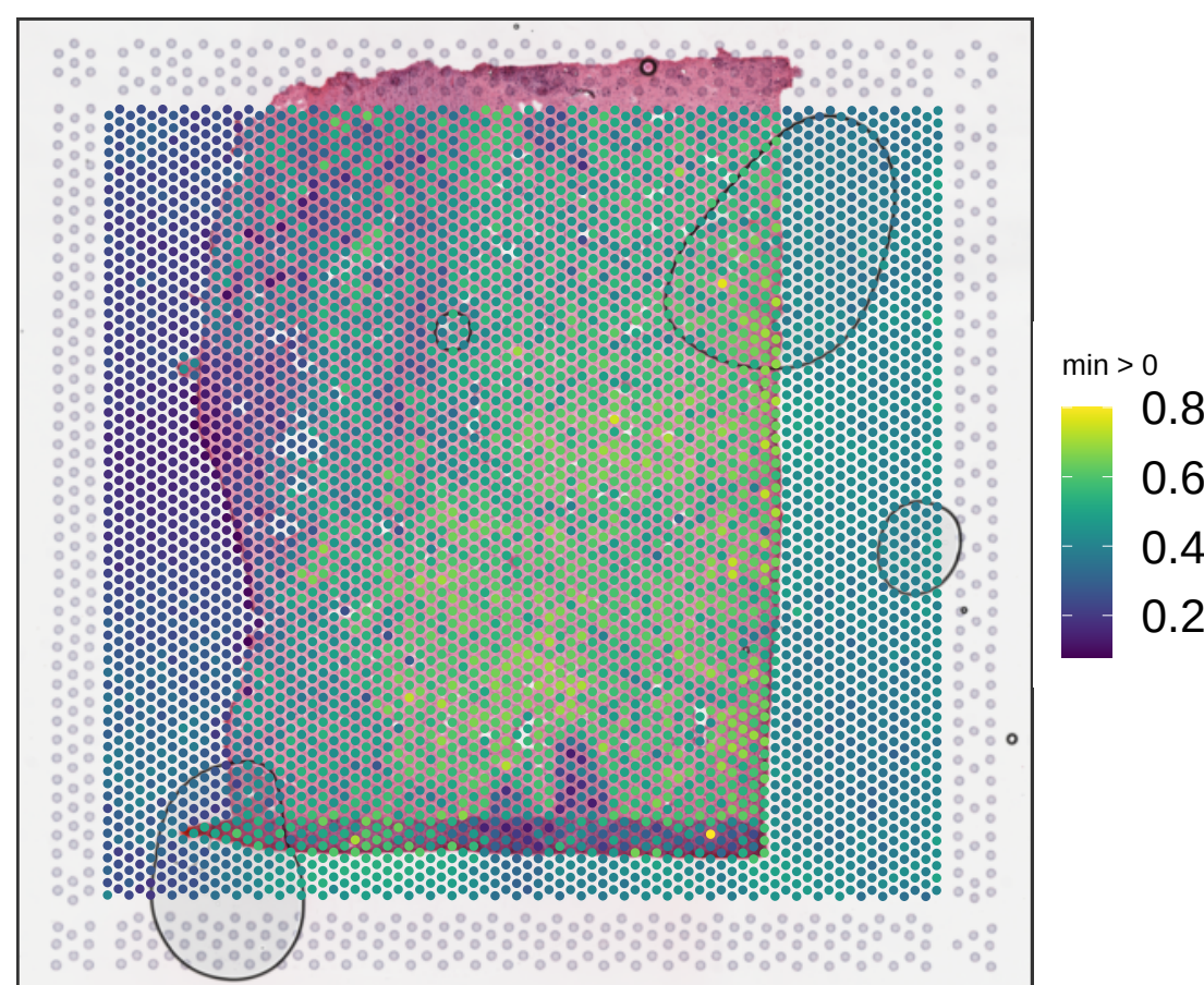
V13B23-285_B1 expr_chrM_ratio
