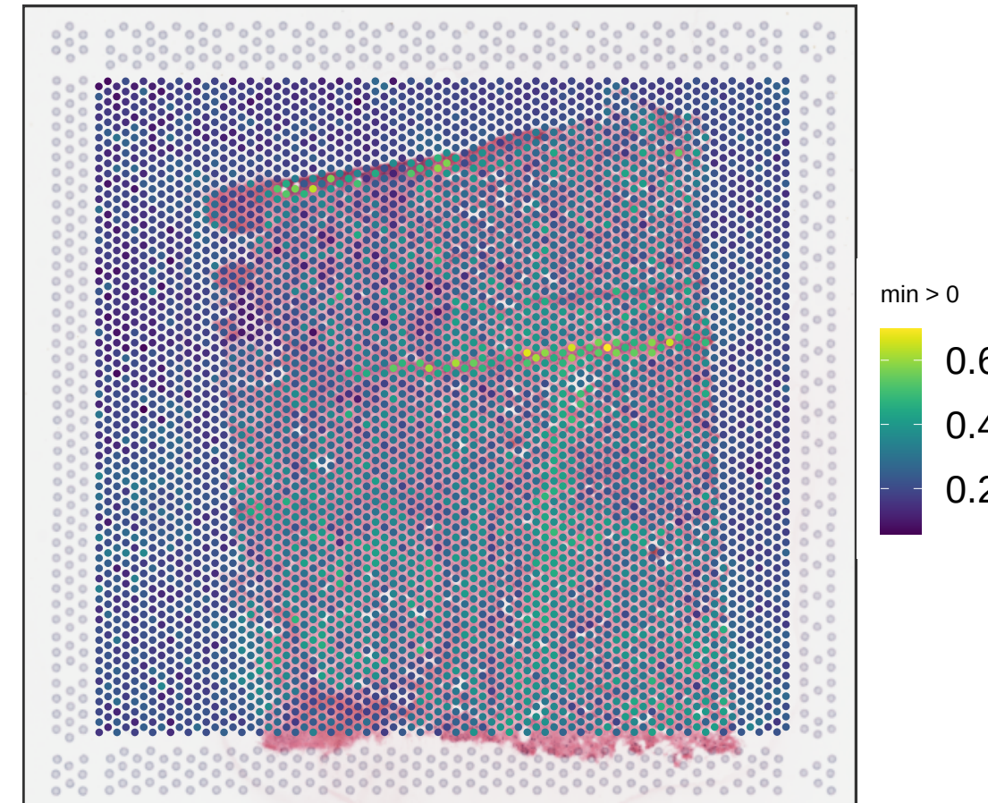
V13B23-281_D1 expr_chrM_ratio
