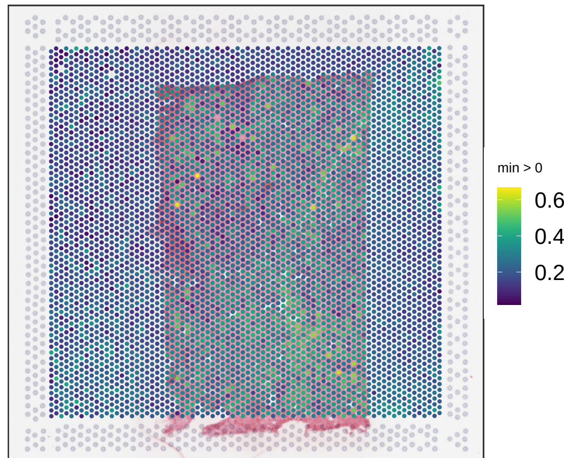
V13B23-281_B1 expr_chrM_ratio
