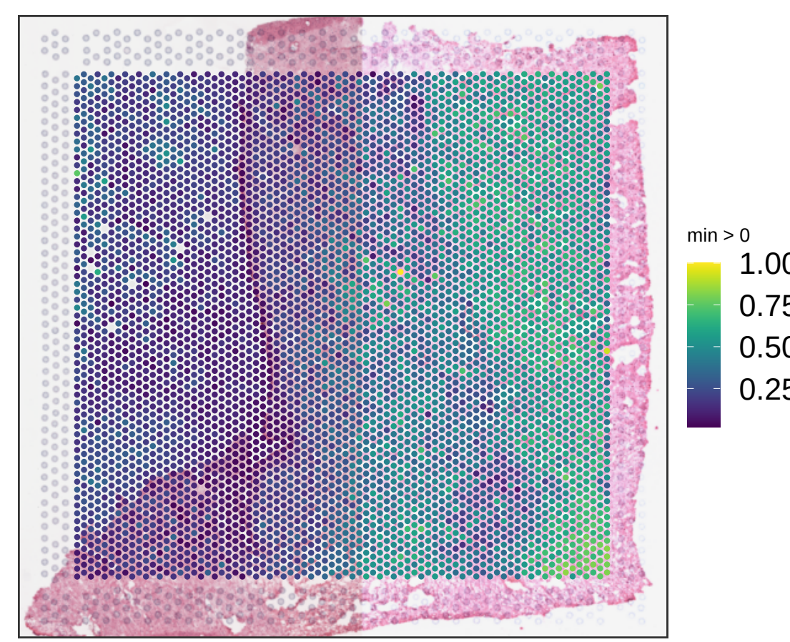
V13B23-280 D1 expr chrM ratio
