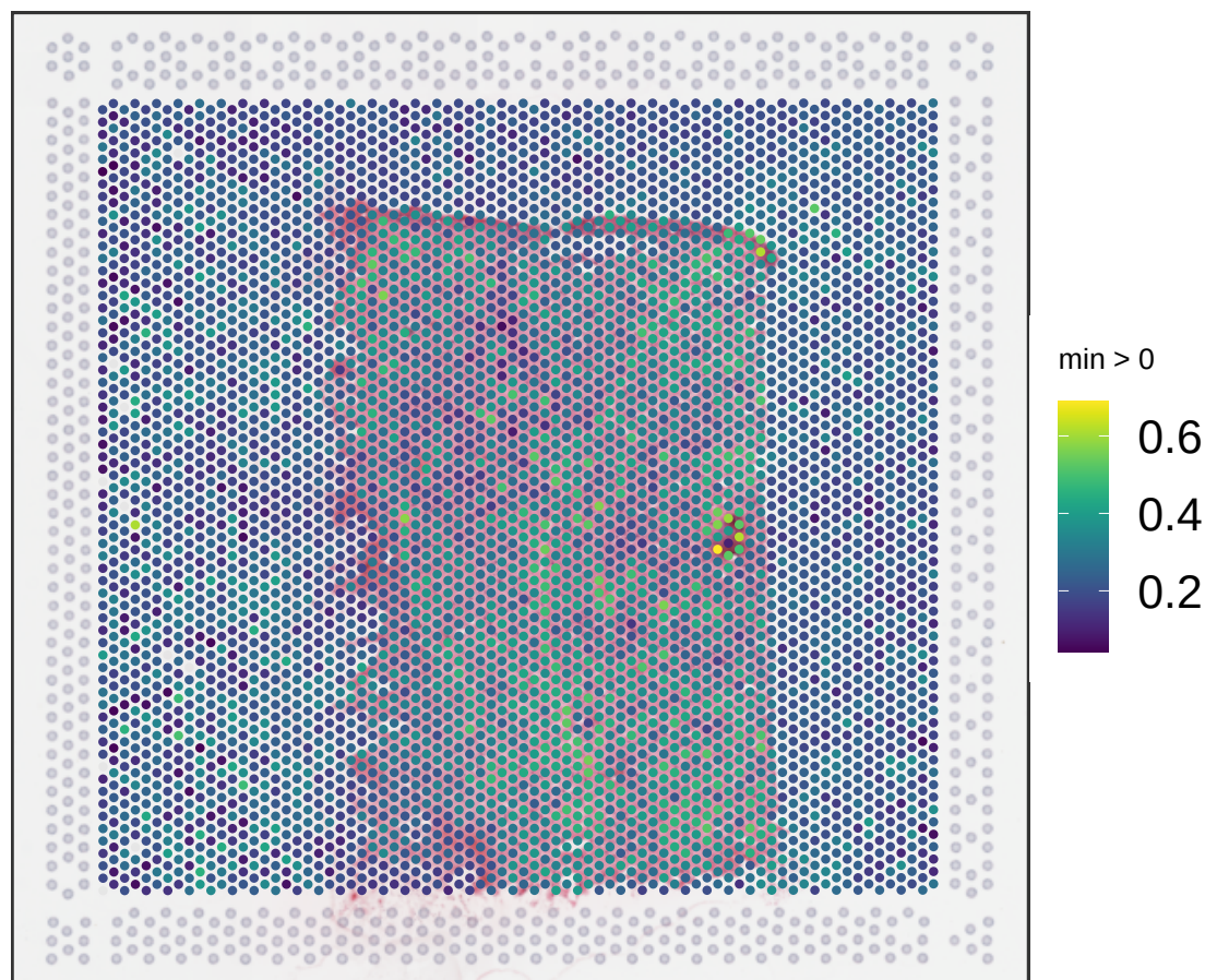
V13B23-281_A1 expr_chrM_ratio
