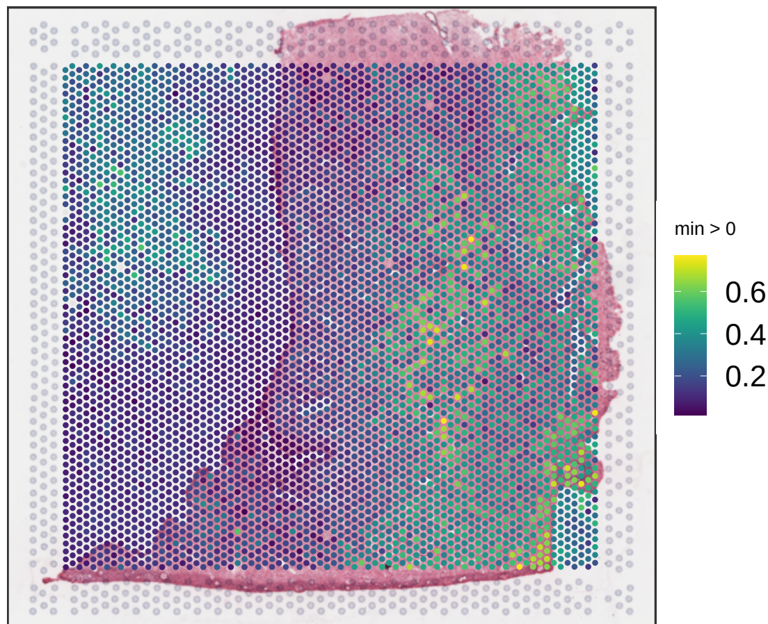
V13B23-280_A1 expr_chrM_ratio
