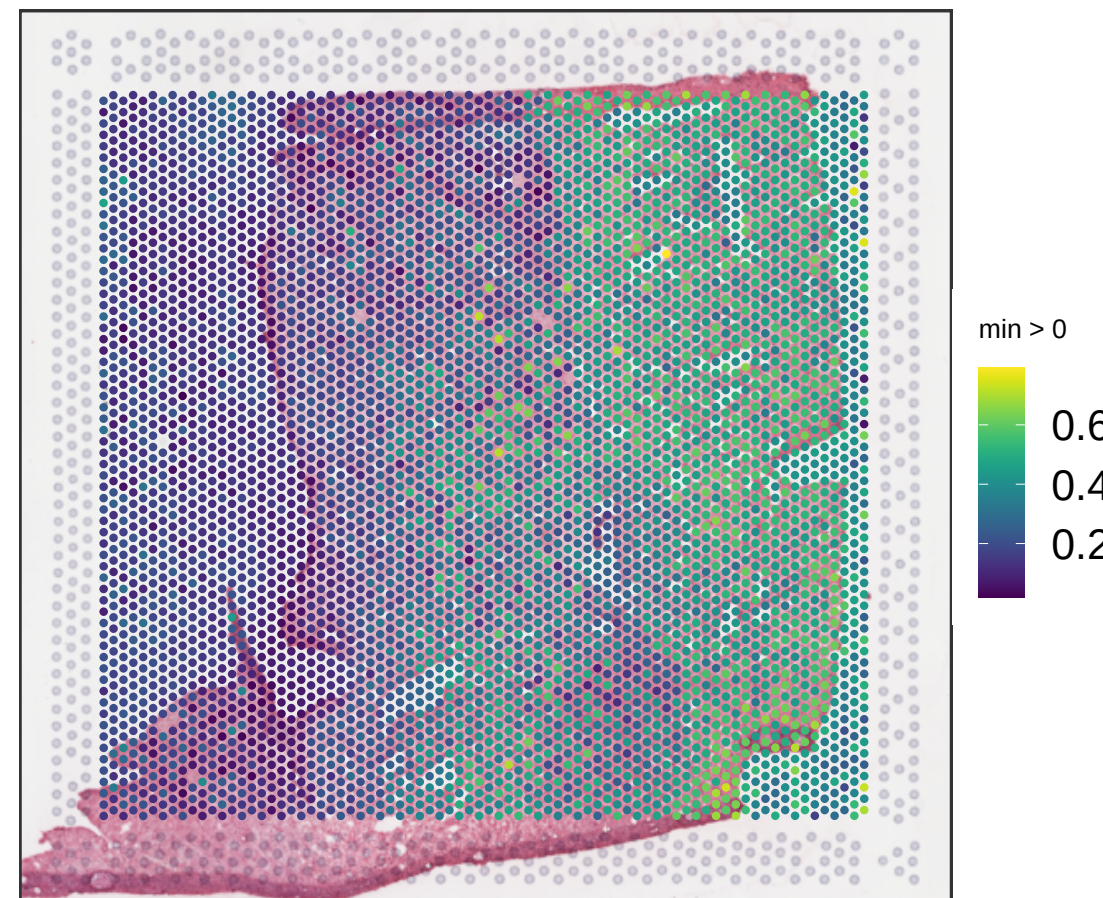
V13B23-280_C1 expr_chrM_ratio
