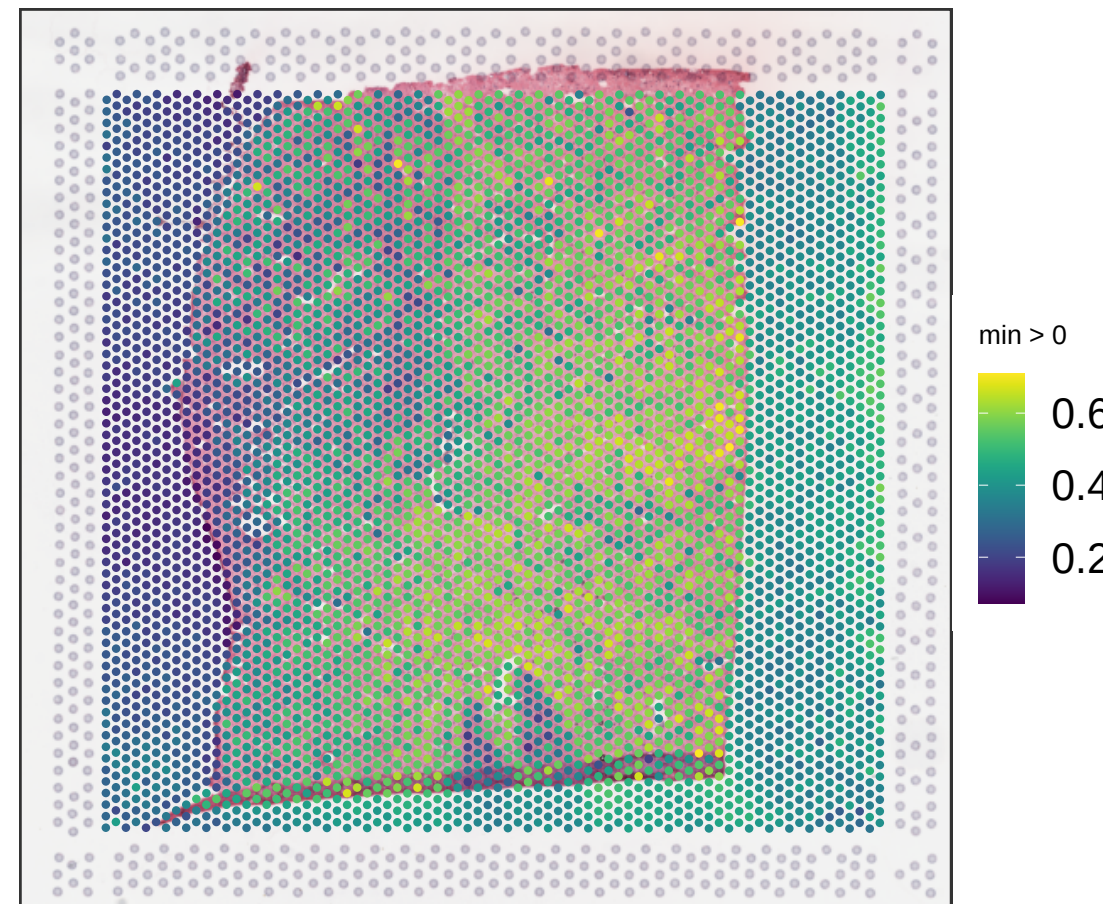
V13B23-285_C1 expr_chrM_ratio
