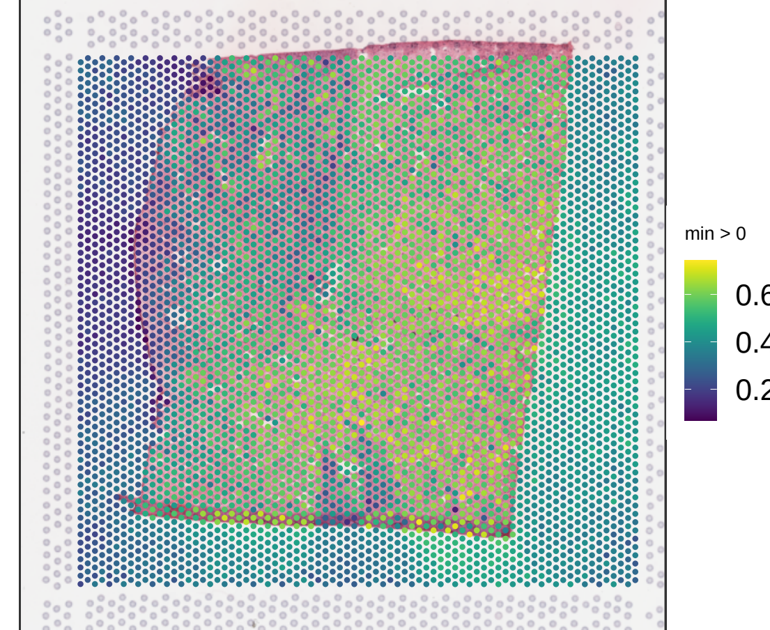
V13B23-285_D1 expr_chrM_ratio
