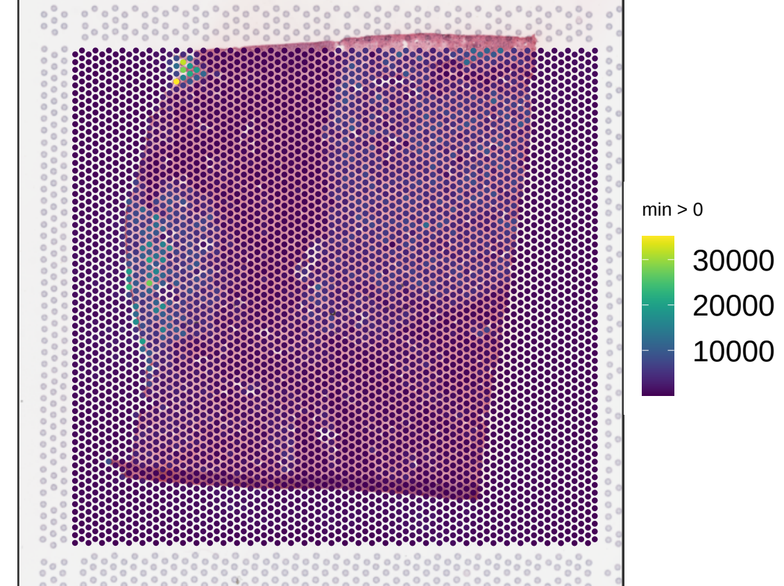
V13B23-285_D1 sum_umi
