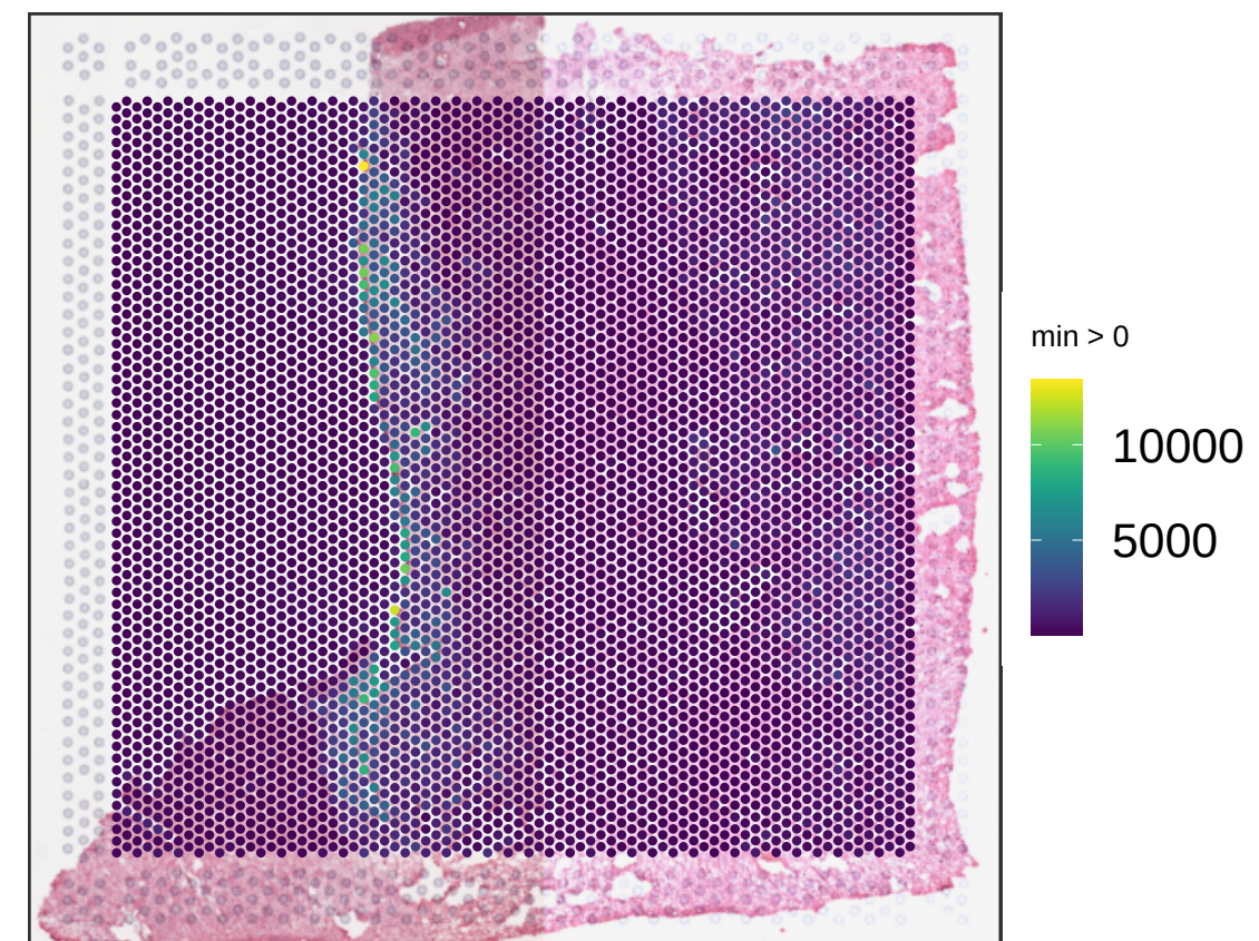
V13B23-280_D1 sum_umi
