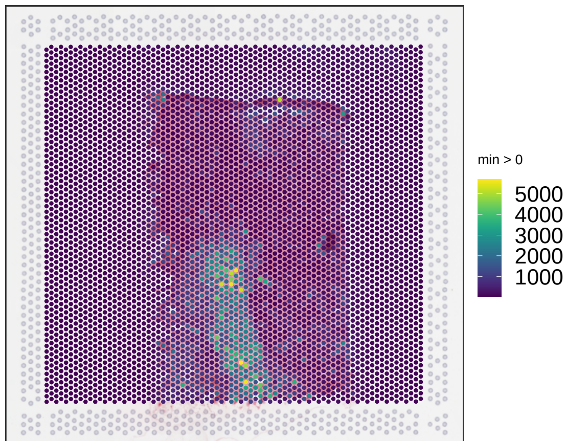
V13B23-281_A1 sum_umi
