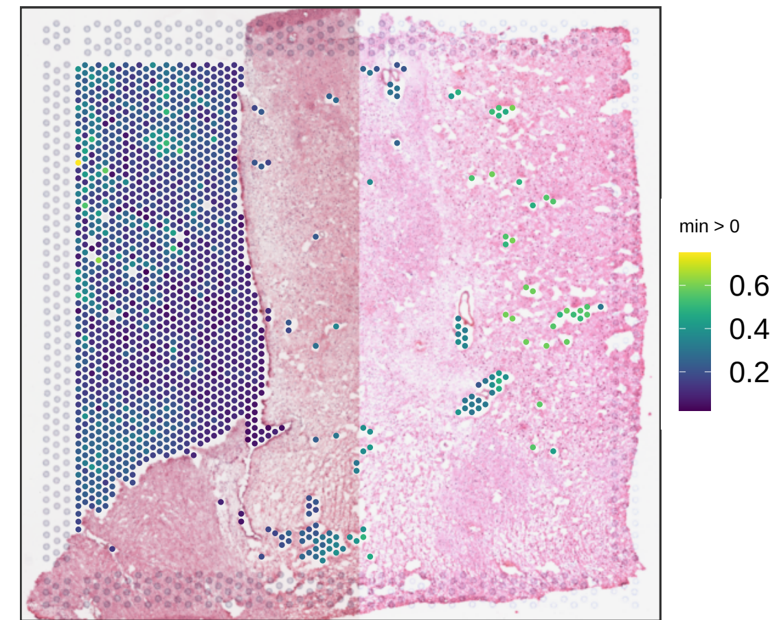
V13B23-280_D1 expr_chrM_ratio
