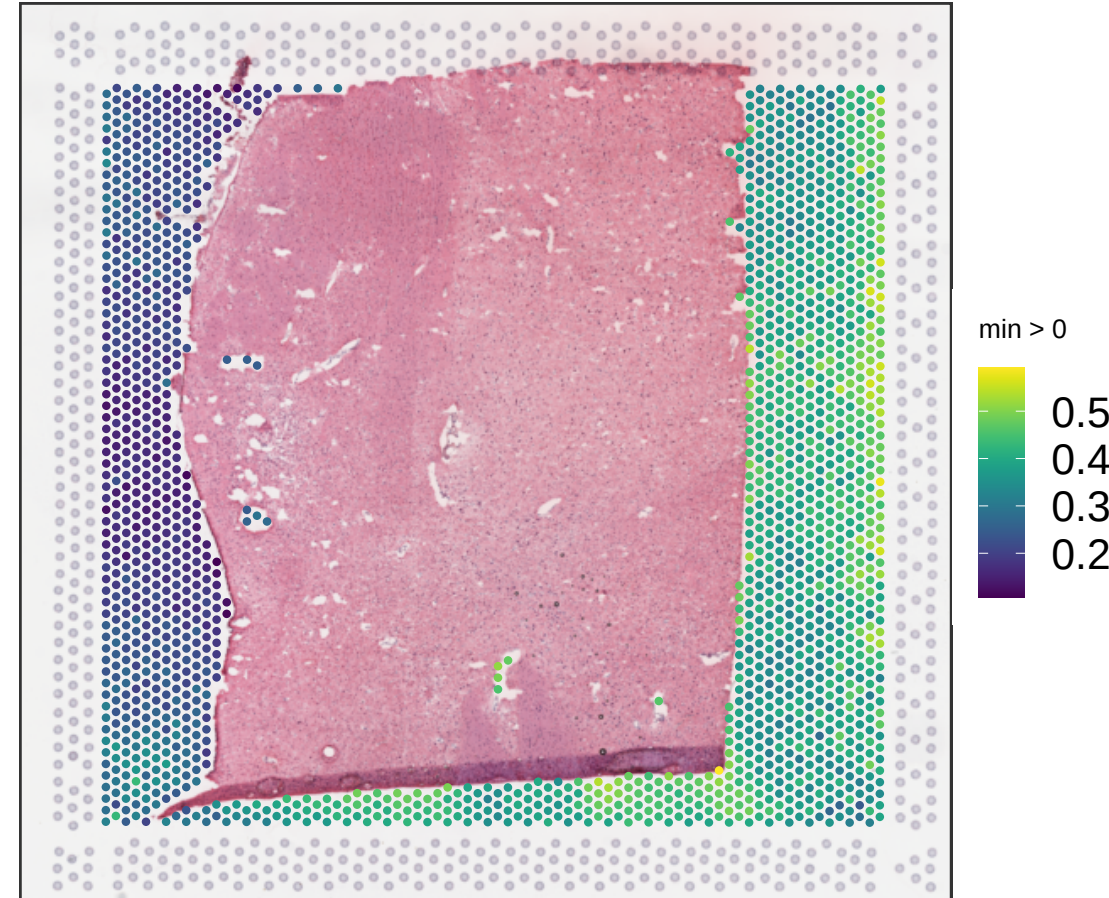
V13B23-285_C1 expr_chrM_ratio
