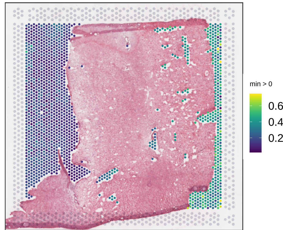
V13B23-280_C1 expr_chrM_ratio
