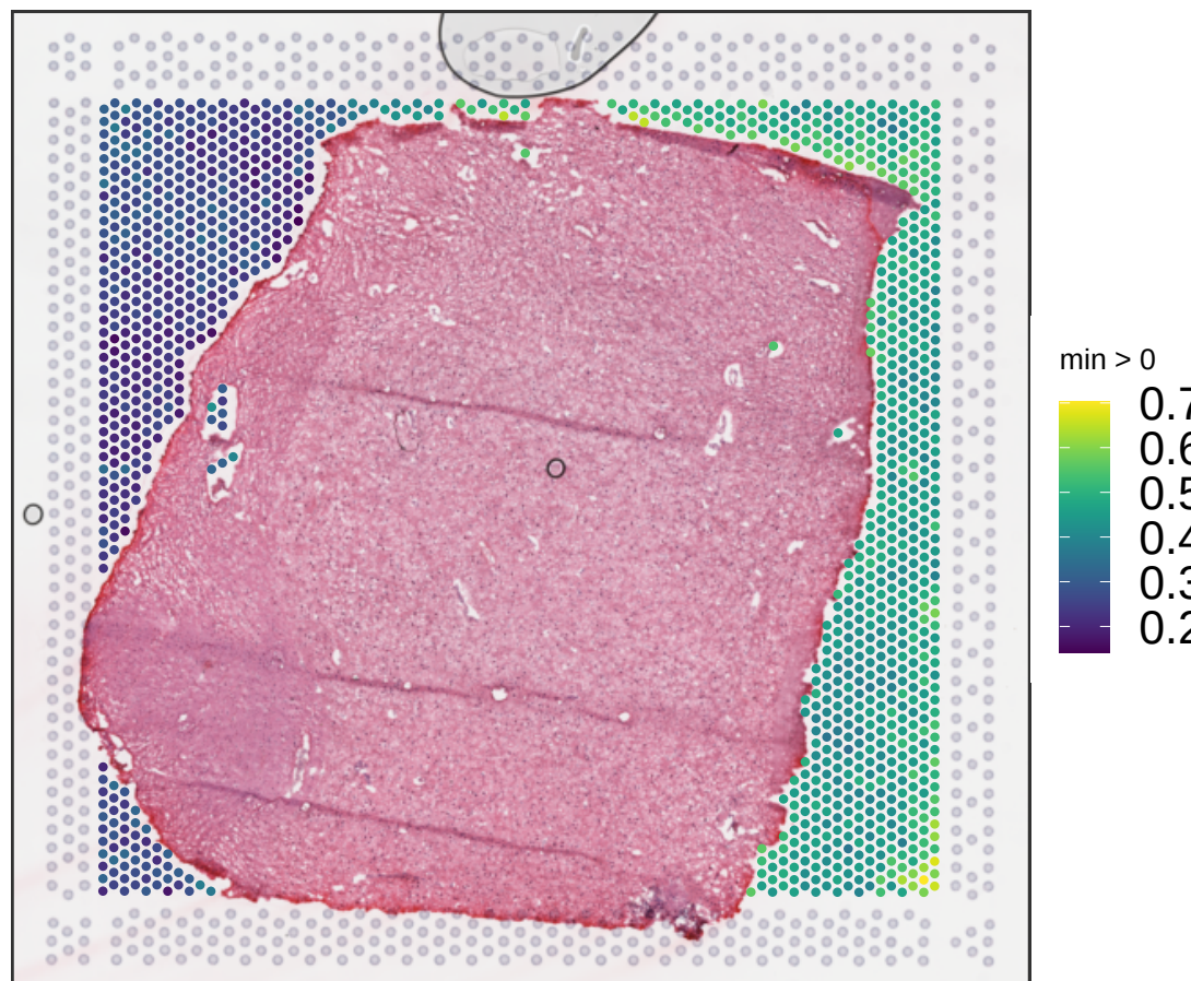
V13B23-285_A1 expr_chrM_ratio
