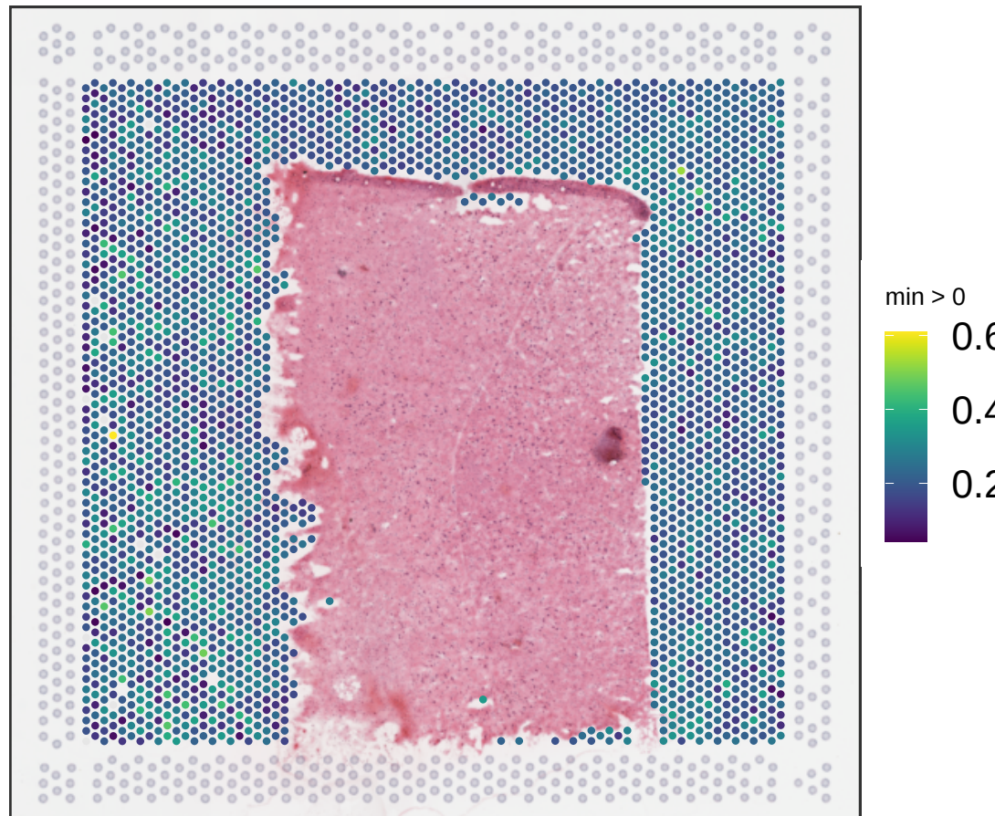
V13B23-281_A1 expr_chrM_ratio
