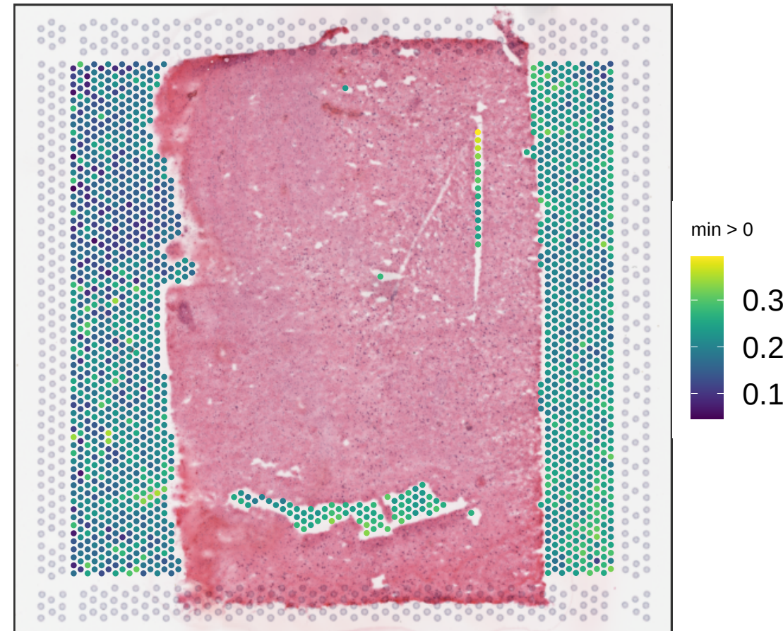
V13B23-281_C1 expr_chrM_ratio
