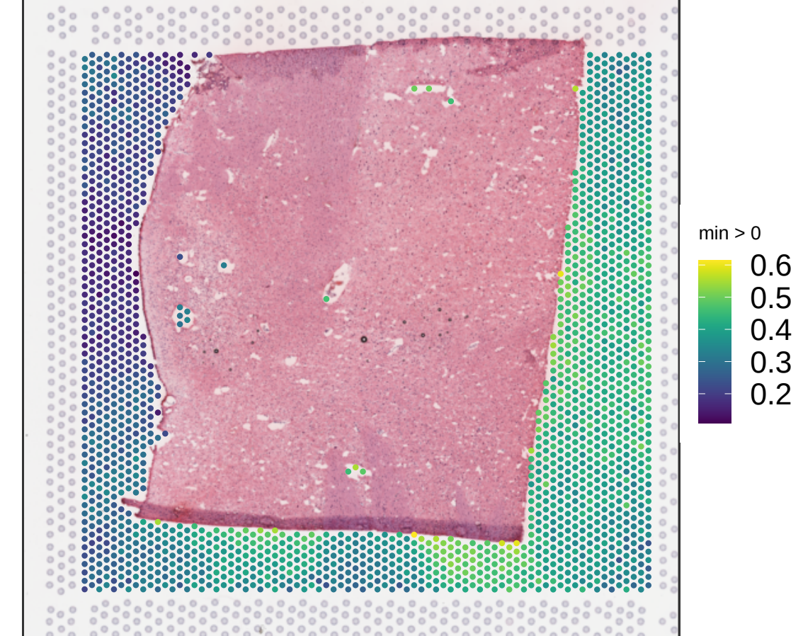
V13B23-285_D1 expr_chrM_ratio
