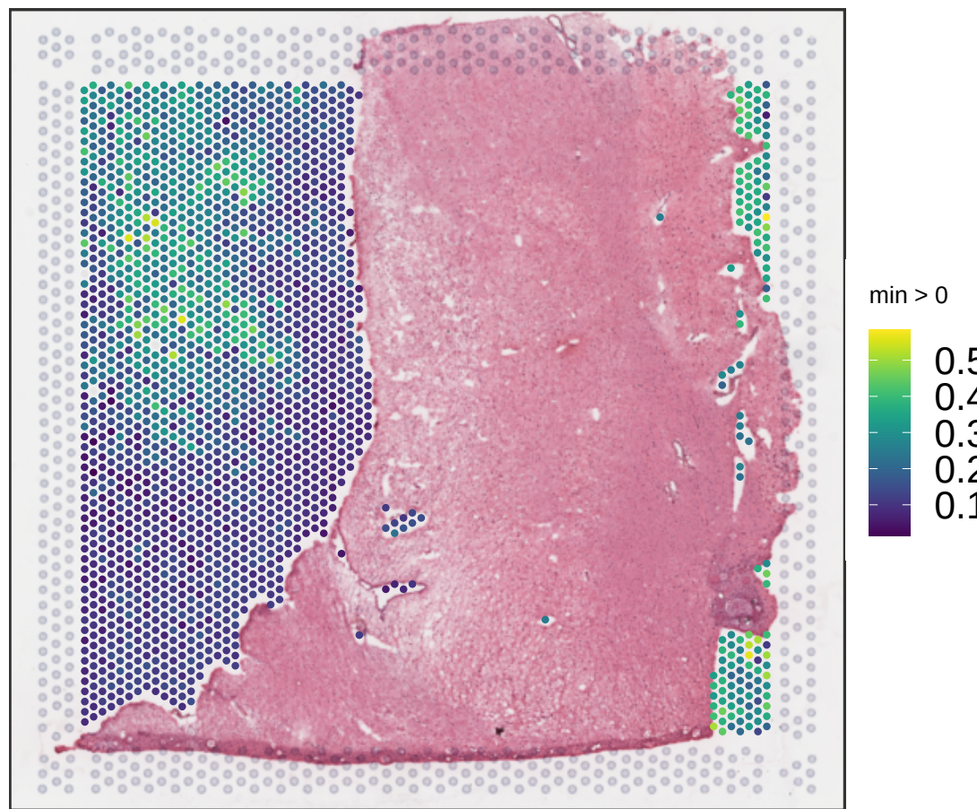
V13B23-280_A1 expr_chrM_ratio
