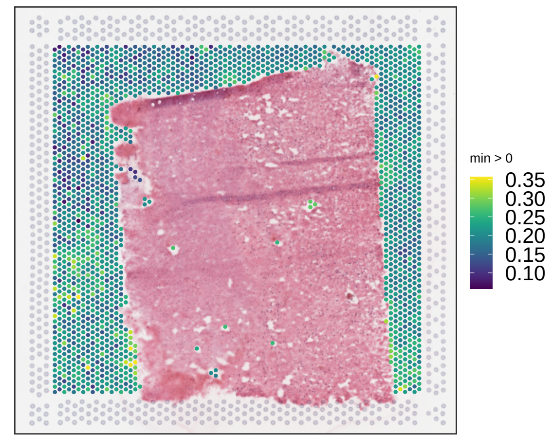
V13B23-281_D1 expr_chrM_ratio
