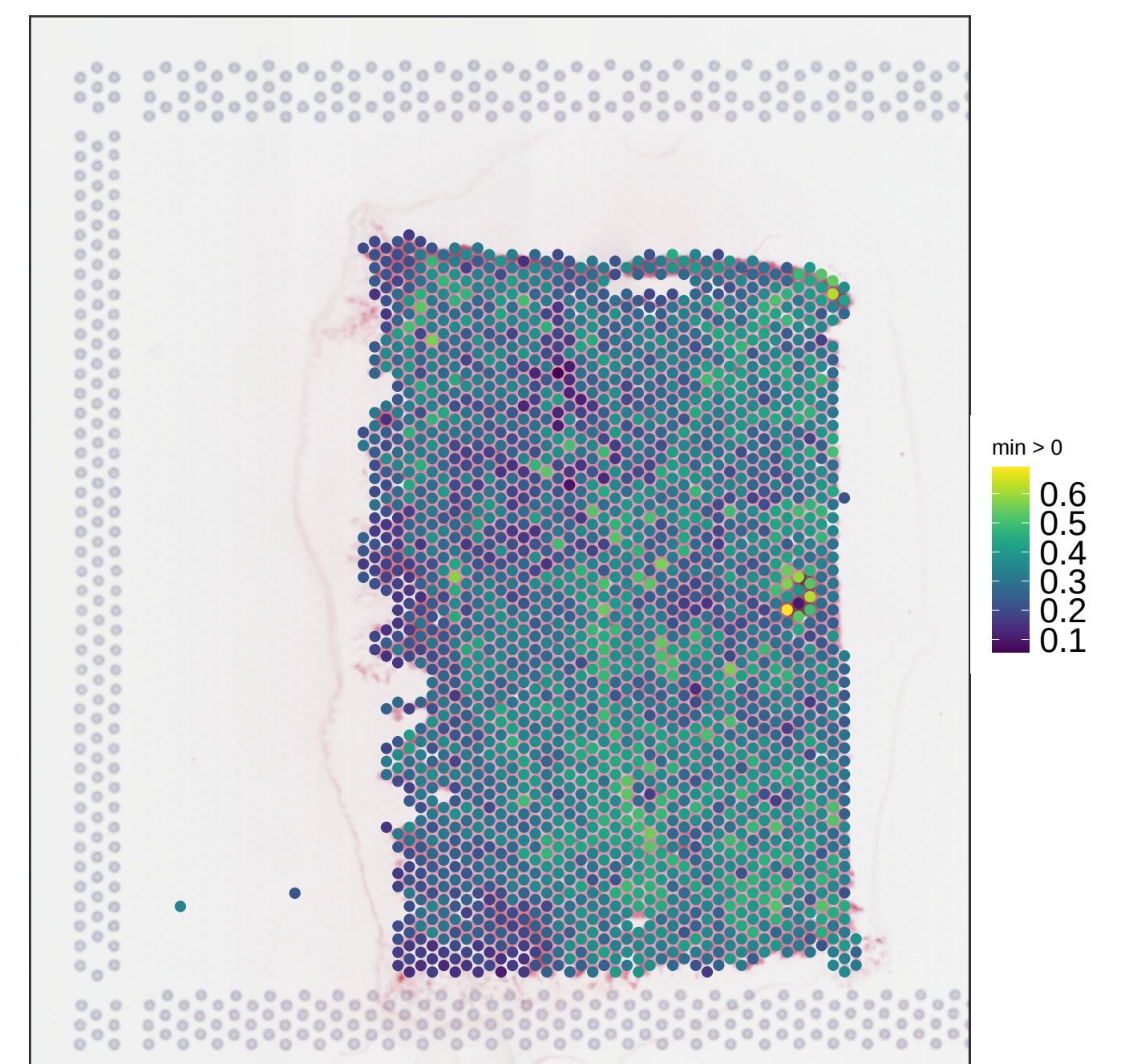
V13B23-281_A1 expr_chrM_ratio
