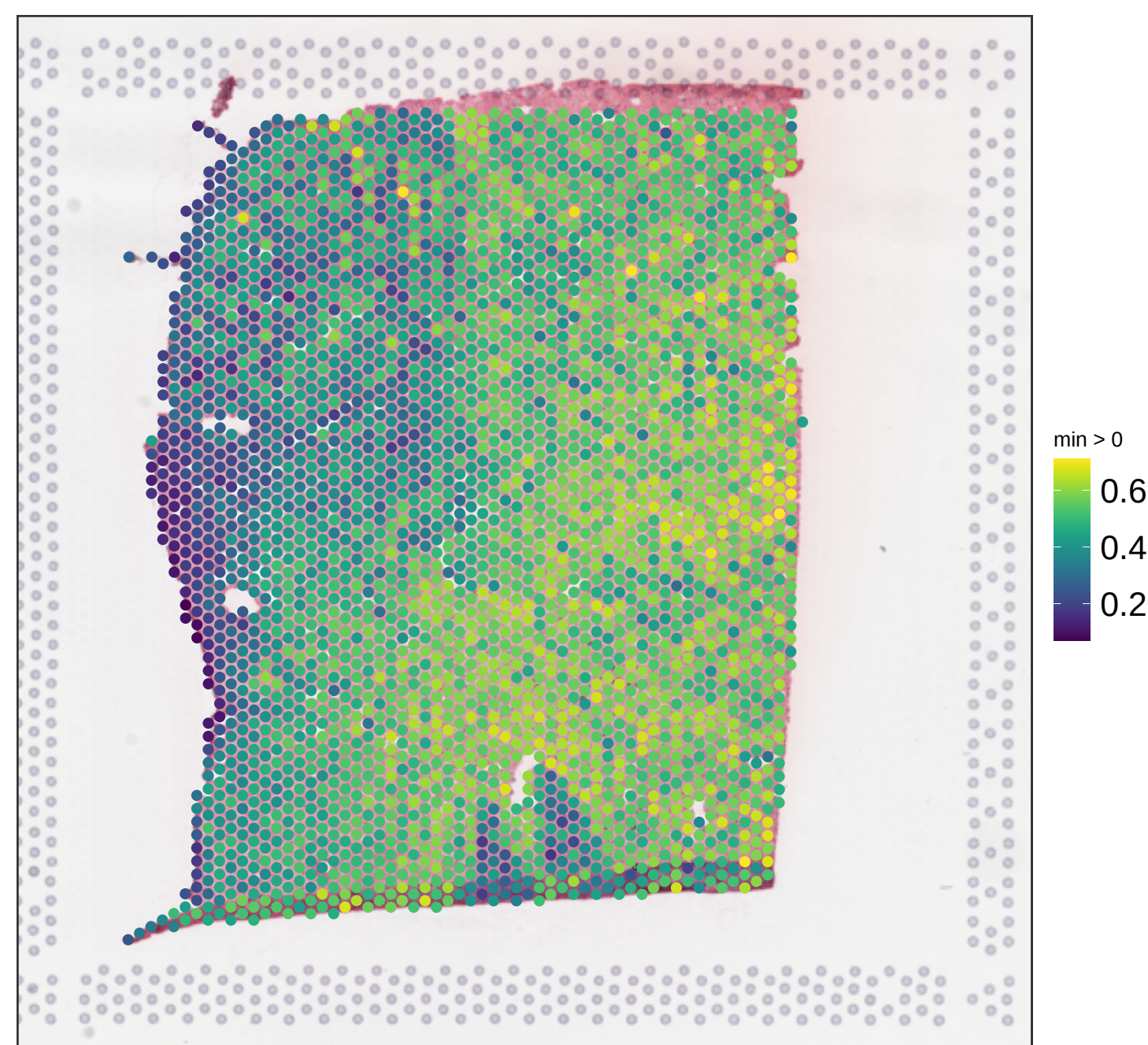
V13B23-285_C1 expr_chrM_ratio
