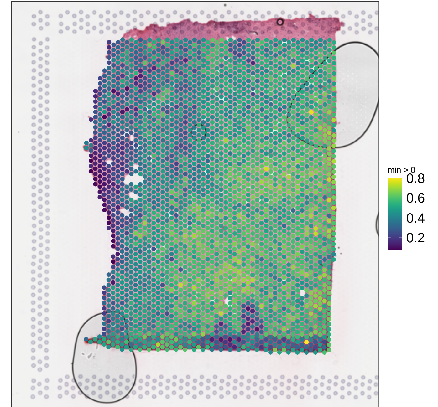
V13B23-285_B1 expr_chrM_ratio
