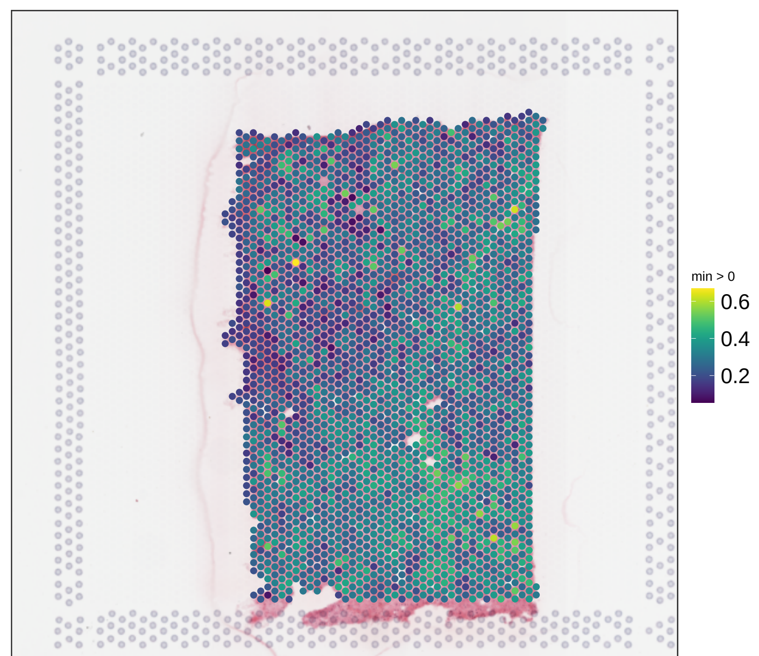
V13B23-281_B1 expr_chrM_ratio
