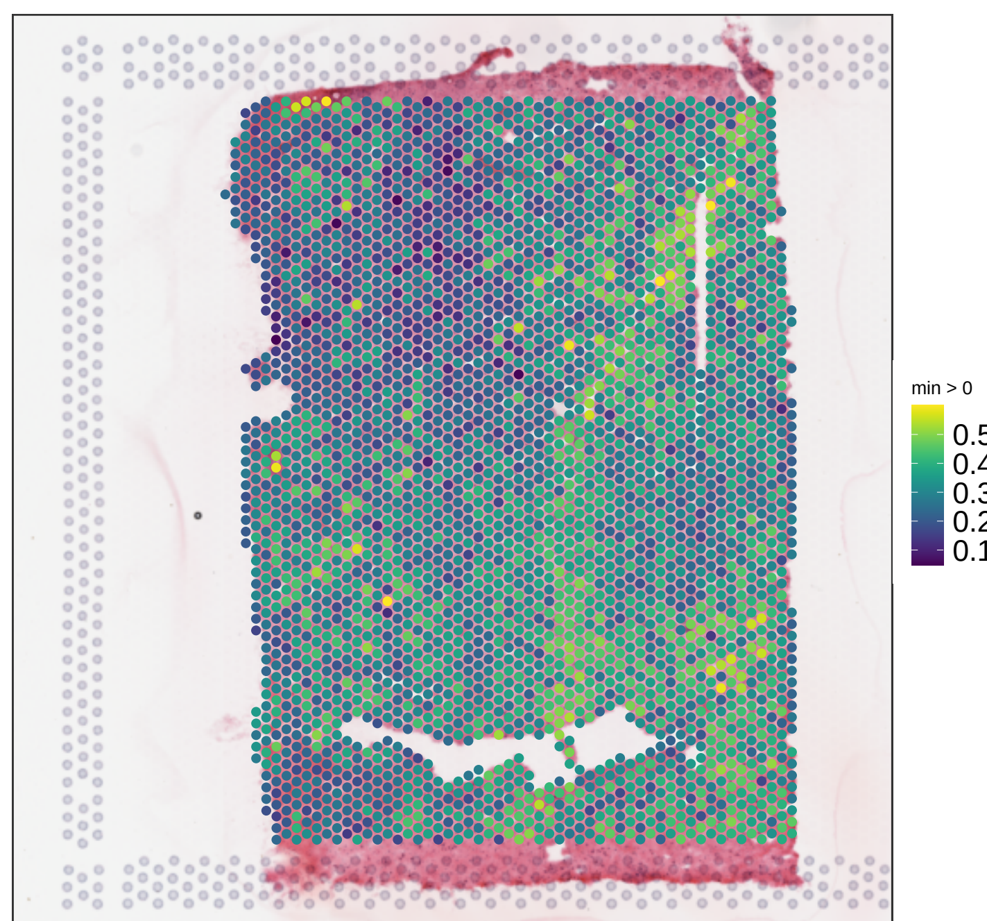
V13B23-281_C1 expr_chrM_ratio
