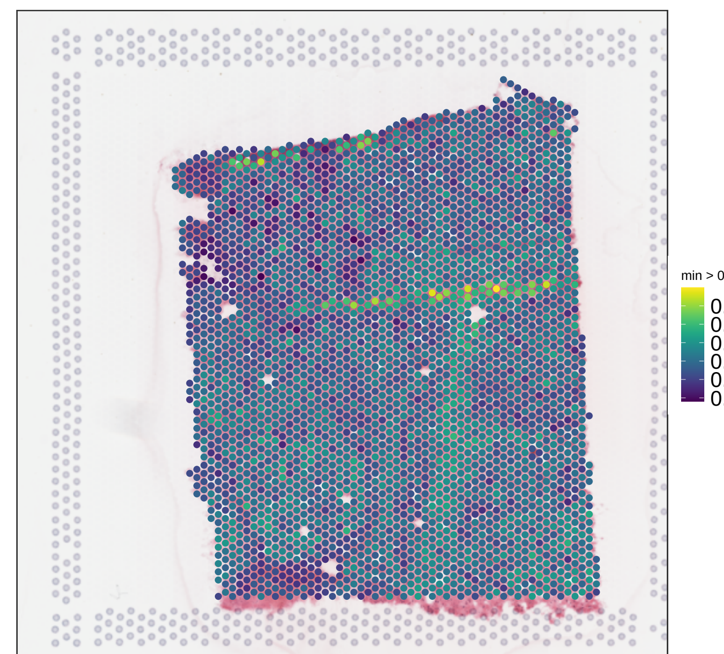
V13B23-281_D1 expr_chrM_ratio
