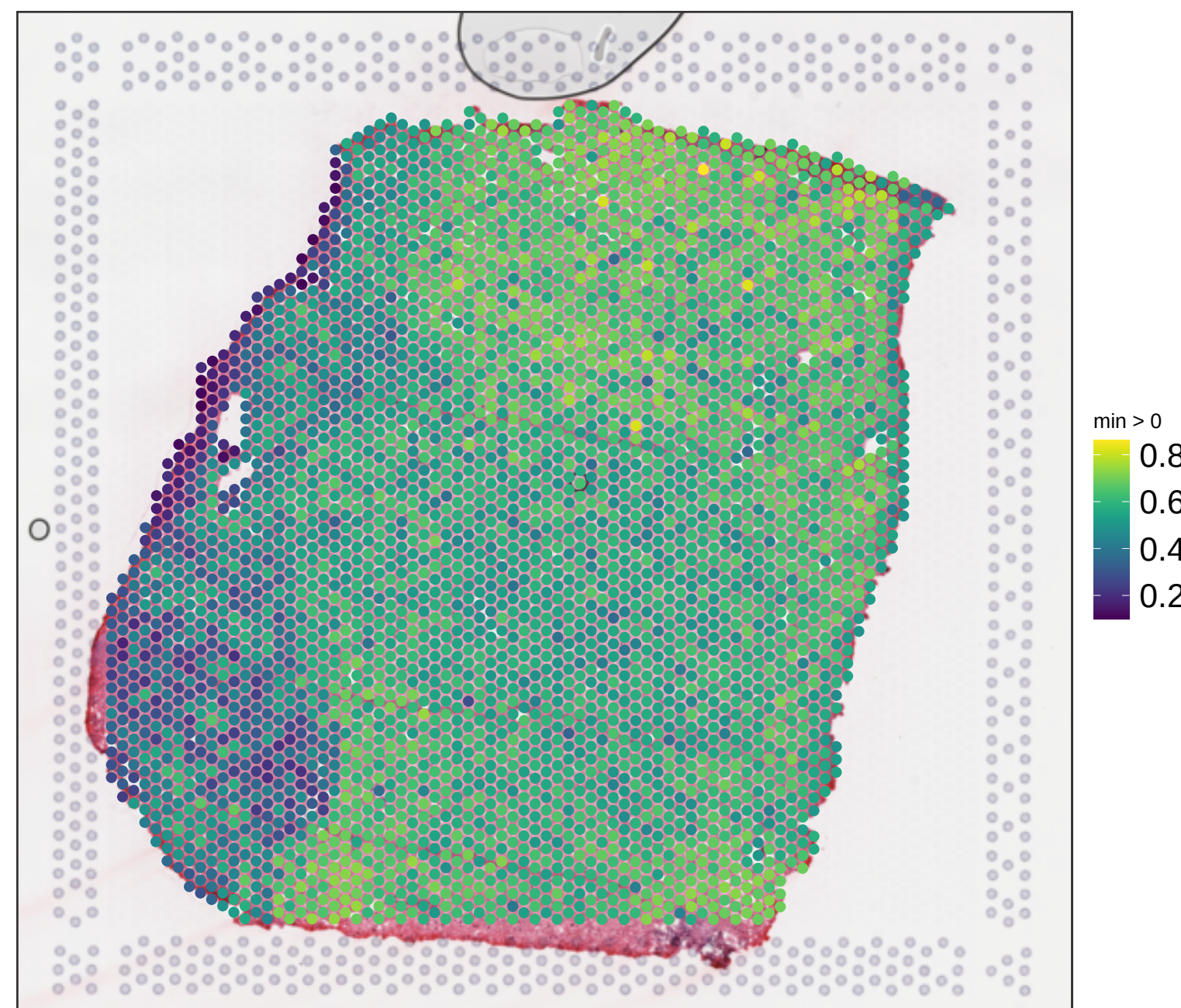
V13B23-285_A1 expr_chrM_ratio
