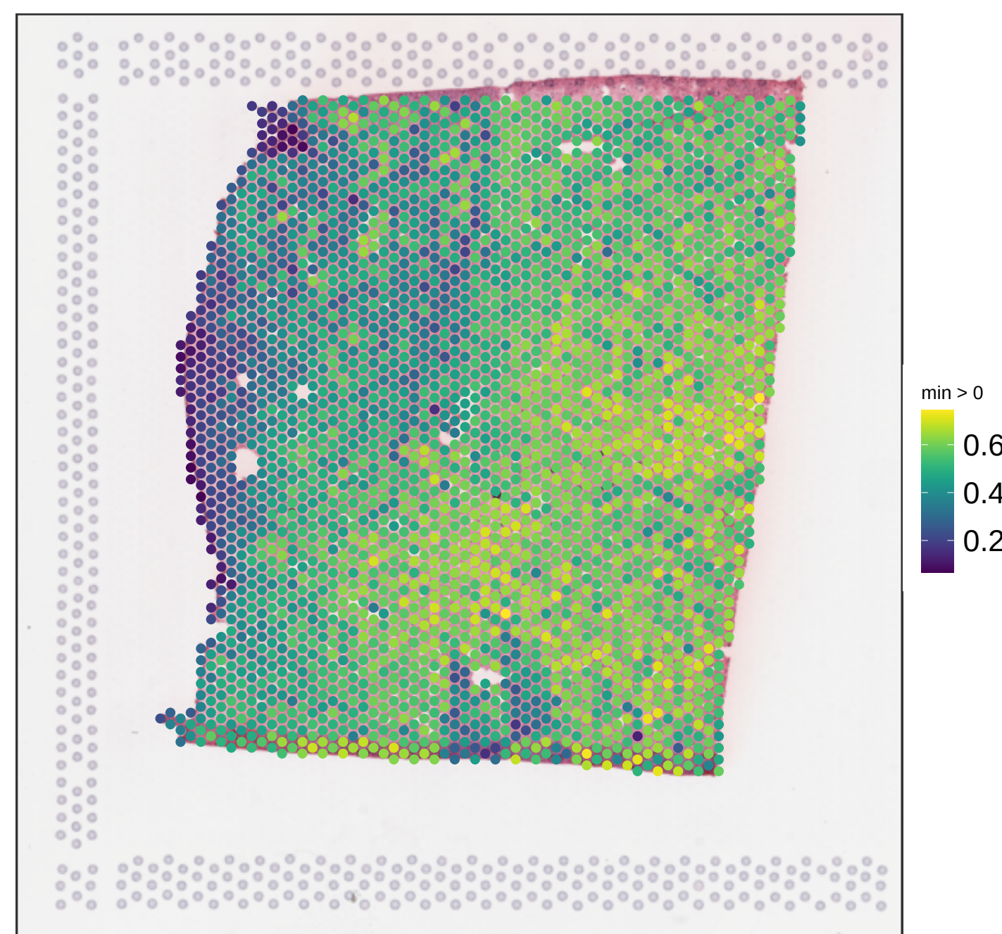
V13B23-285_D1 expr_chrM_ratio
