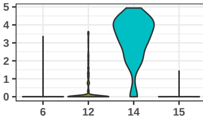
NEUROD1
