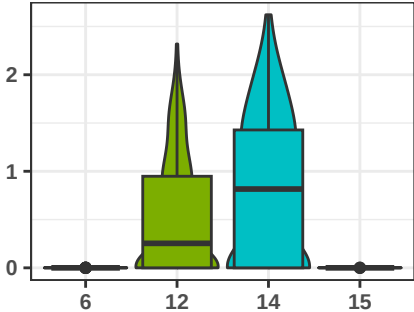
POU4F1
