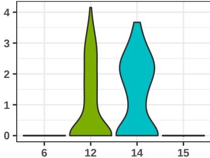
GPR151
