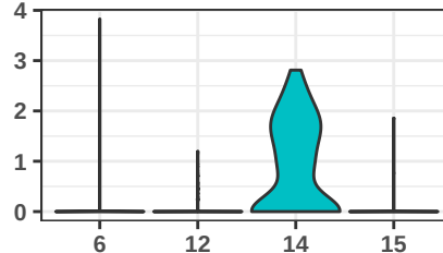
SCUBE1
