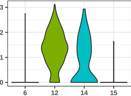
EPHA5
