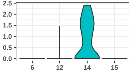
CHRNA3
