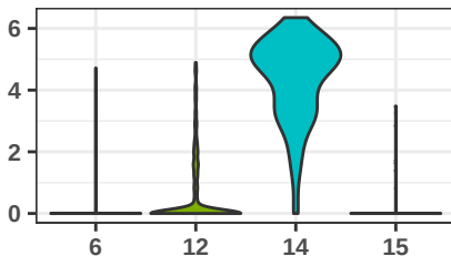
GNG8
