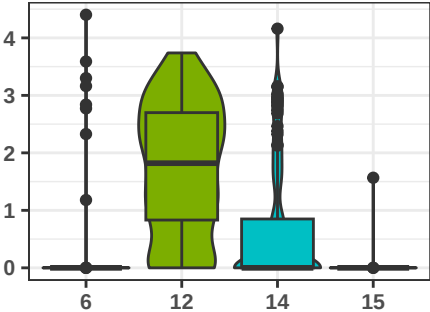
TLL1
