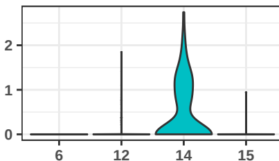
CD24
