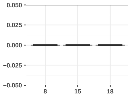
POU4F1
