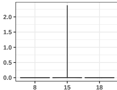
GPR151
