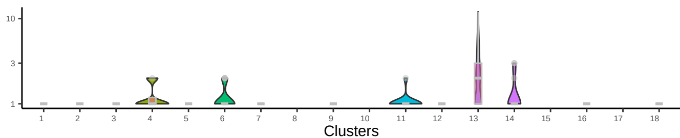
Log10 Exp – ANO3
