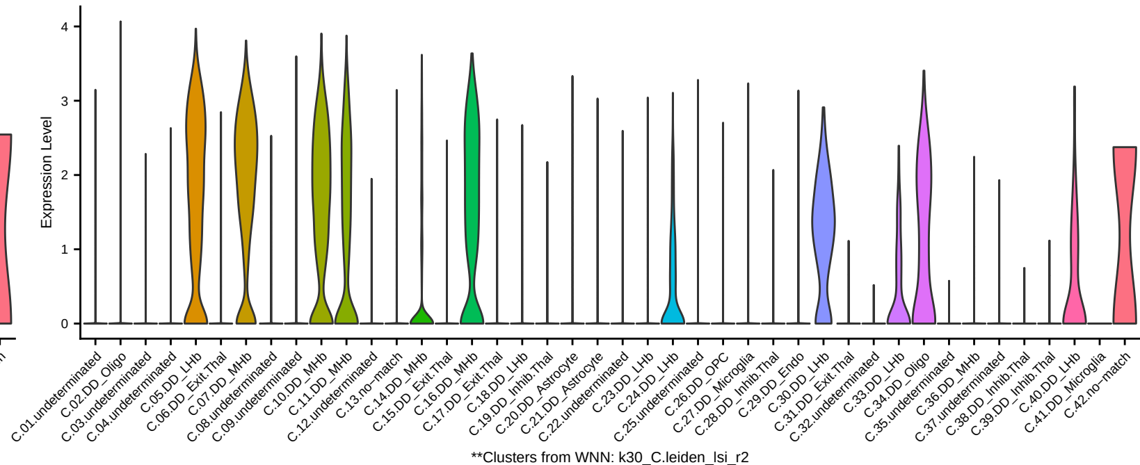
GPR151
