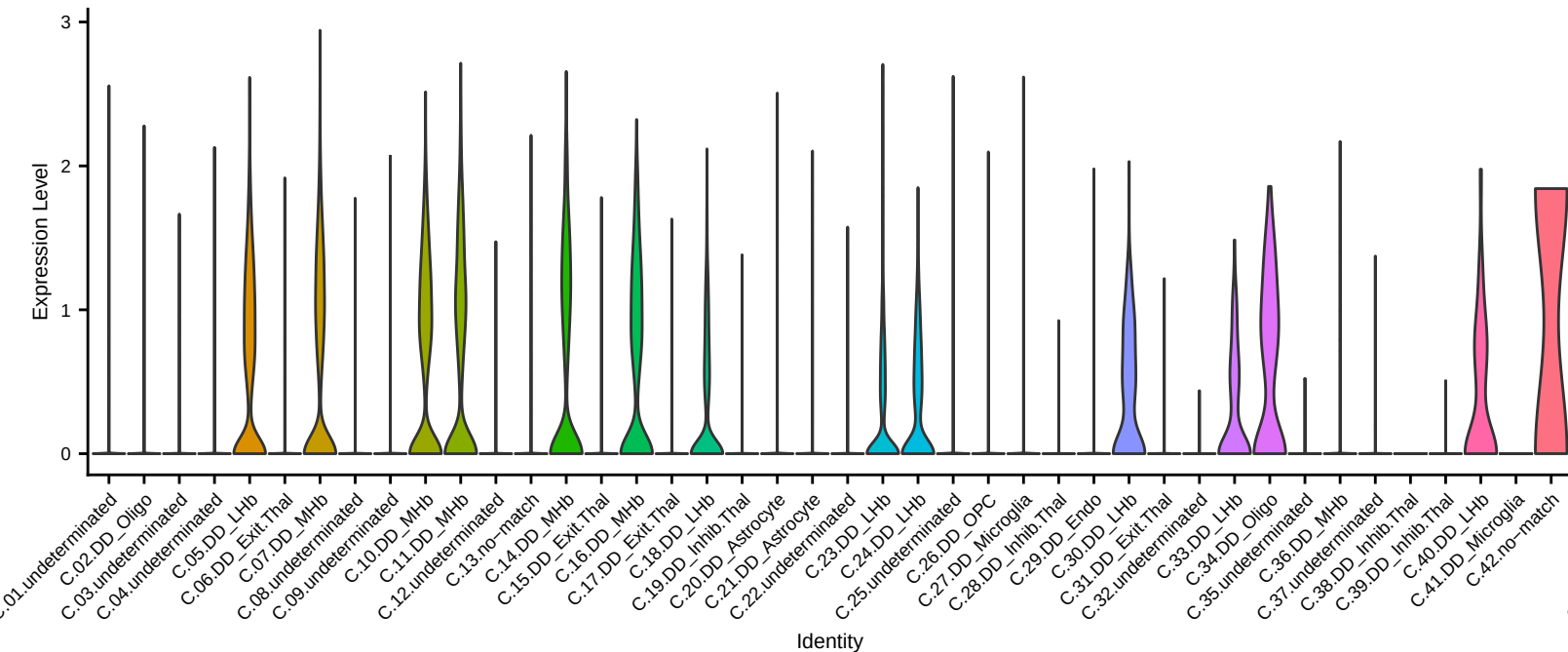
POU4F1
