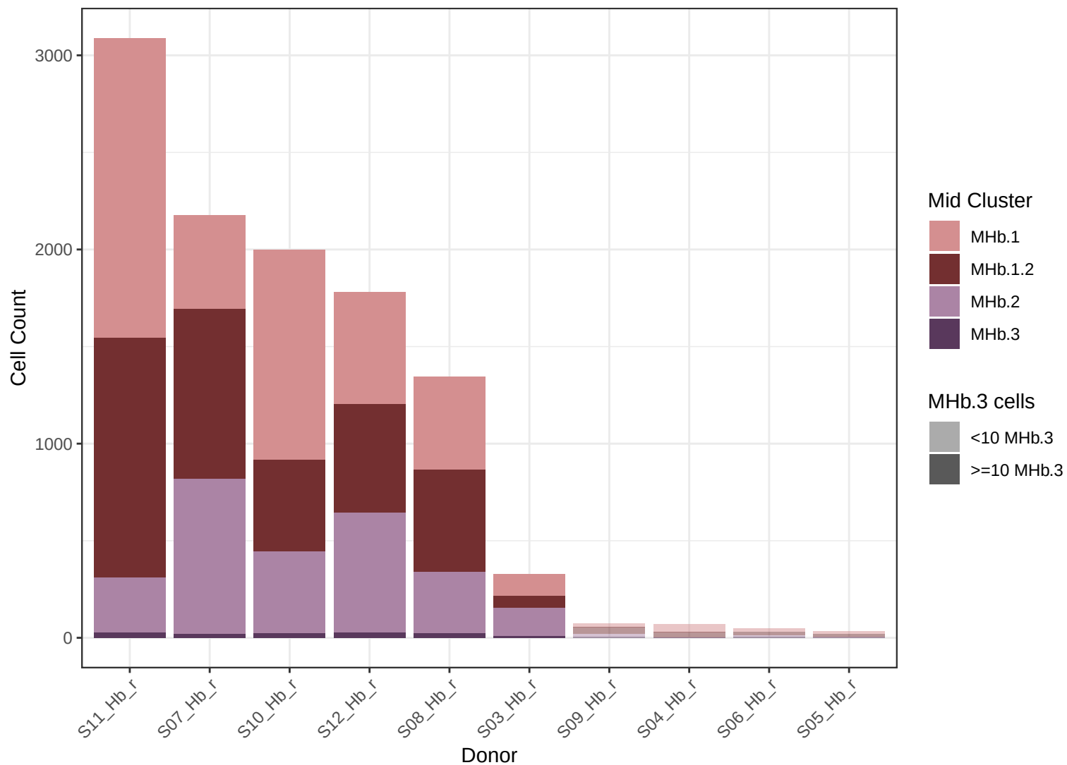
Medial habenula clusters per donor
